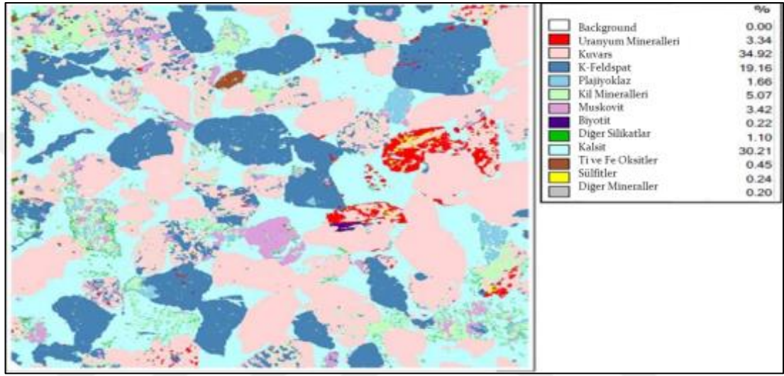
Şekil 6.5: Şekil 6.1'deki 4 numaralı alanın mikroskobik görüntüsü.
