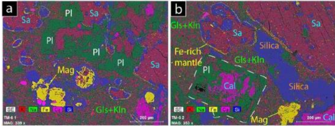
Şekil 6.21: TM6 numaralı örneğin SEM-EDS kullanılarak oluşturulmuş görüntüleri
