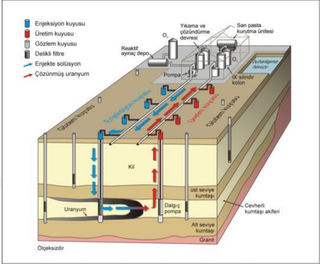
Şekil 9.2: Yerde Kazanım Yönteminin blok model üzerinde gösterilmesi.
