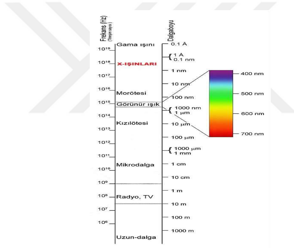
Şekil 2.5: Elektromanyetik spektrumda x-ışınlarının gösterimi.
