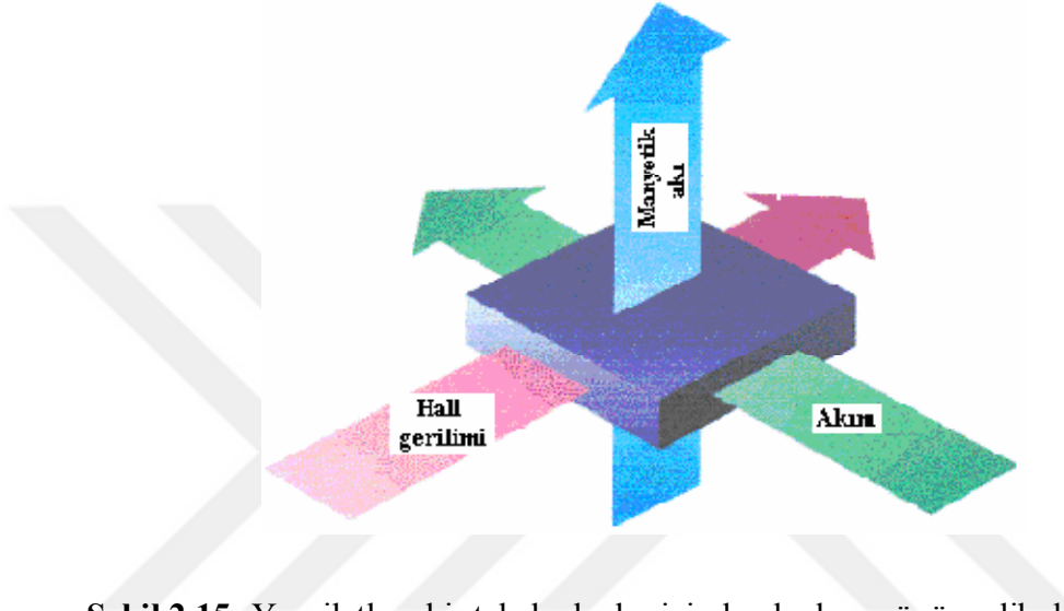
Şekil 2.15: Yarı iletken bir tabakada, harici olarak akım yönüne dik doğrultuda etkiyen manyetik bir alan etkisiyle oluşan Hall gerilimi [28].
