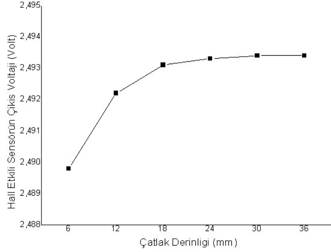
Şekil 4.9: Hall etkili sensörün çıkış voltajının yarım çatlak modelindeki çatlak derinliğine göre değişimi.
