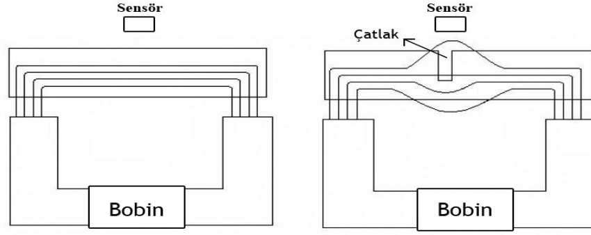
Şekil 2.11: Manyetize edilmiş malzeme üzerinde bulunan çatlak bölgesindeki manyetik akı çizgilerinin davranışı.
