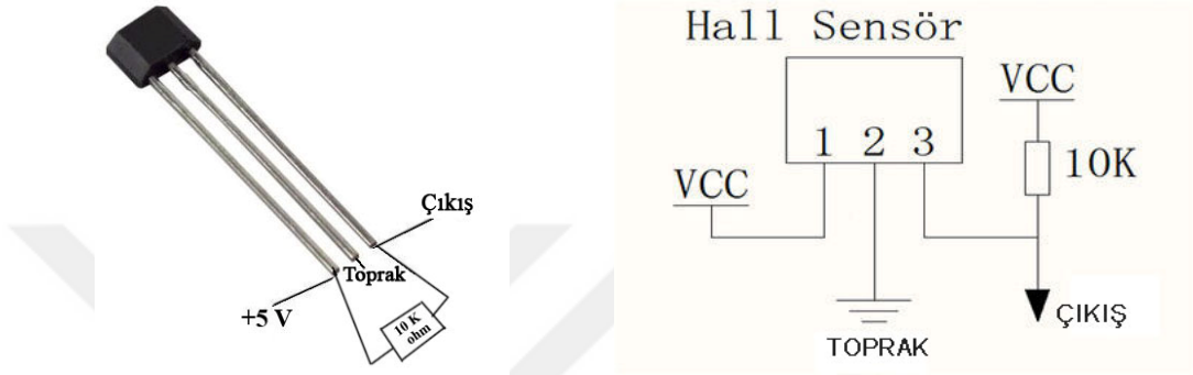
Şekil 2.19: Hall etkili sensör.
