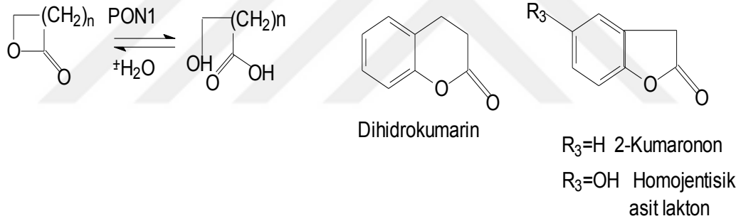
Şekil 1.4: Lakton hidrolizi [20].
