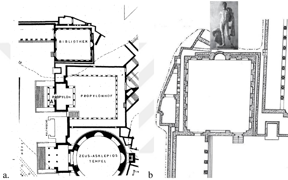
Şekil 3.49: Pergamon Asklepiyon Kütüphanesi Planı ve Plan Kesiti
