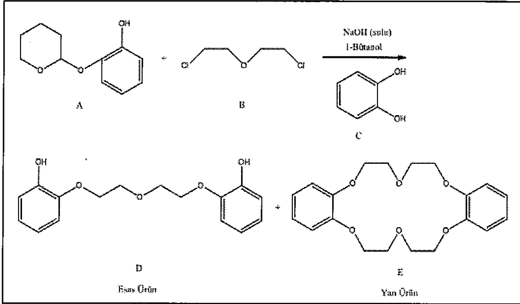
Şekil 1.1: Pedersen tarafından sentezlenen ilk crown eterler [5].
