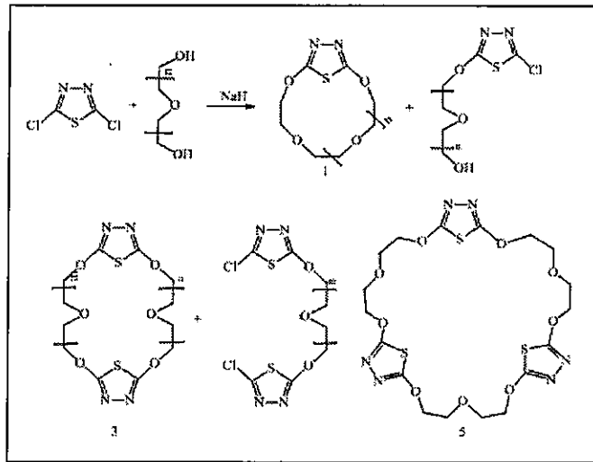
Şekil 1.2: Tiyadiazol kullanılarak yapılan halkalaşma reaksiyonları.
