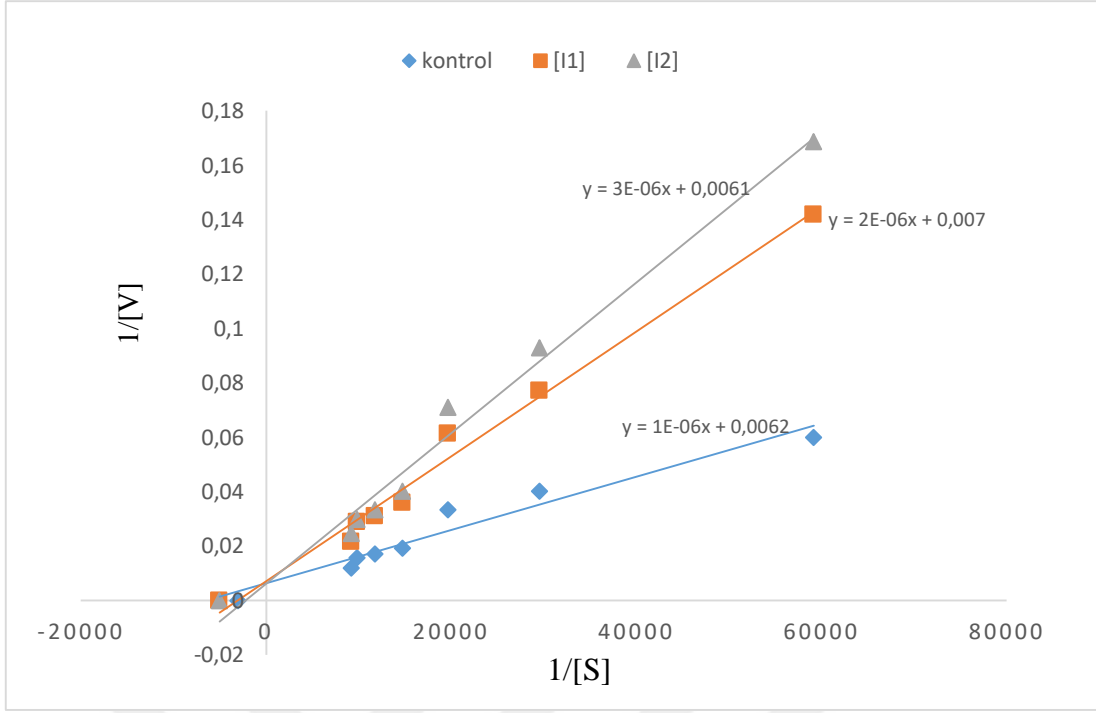
Şekil 3.22: Saflaştırılan LPO enzimi için ABTS substratı ve hekzan ile elde edilen 1/[S] - 1/V grafiği.
