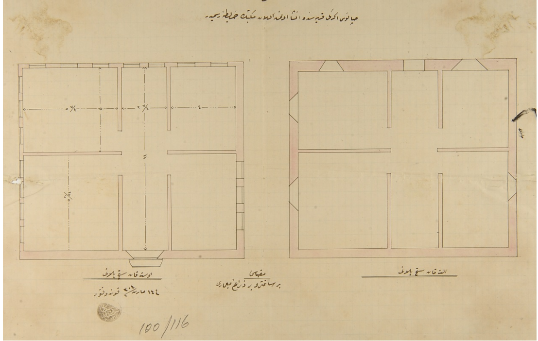
Resim Hapanos Ekreki Köyü'nde İnşa Edilen Mektebin Planı
