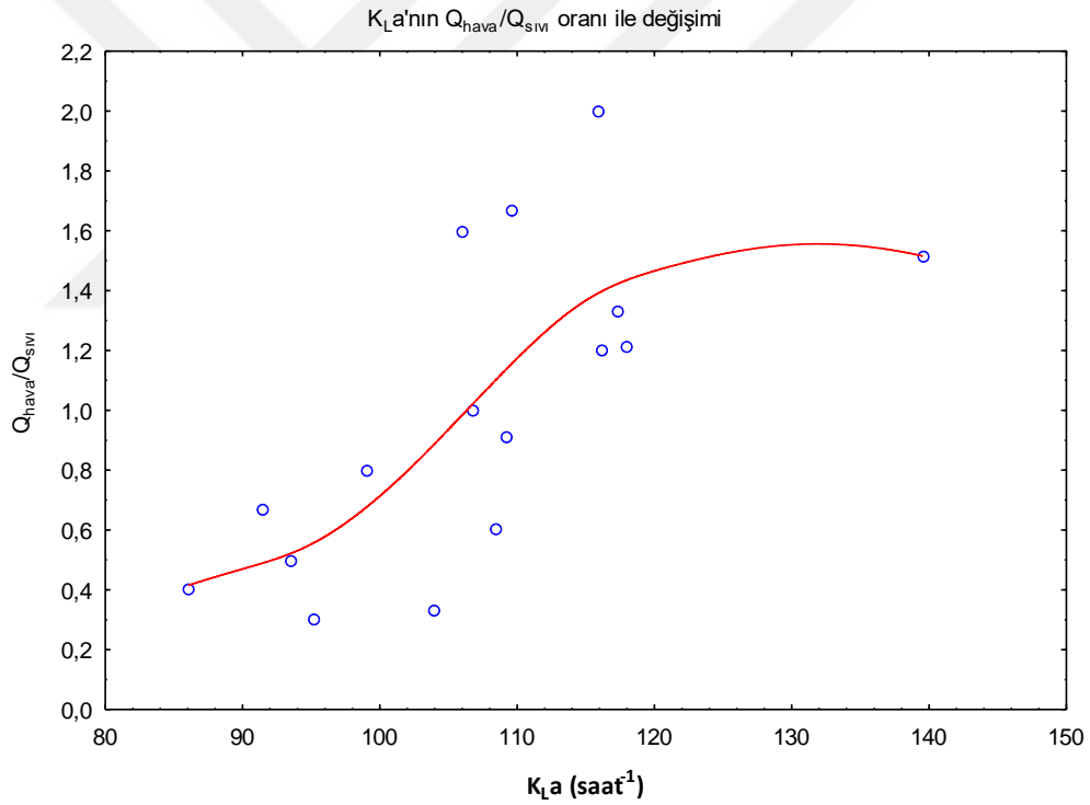
Şekil 5.3: K_{La} değerlerinin hava debileriyle değişimi
