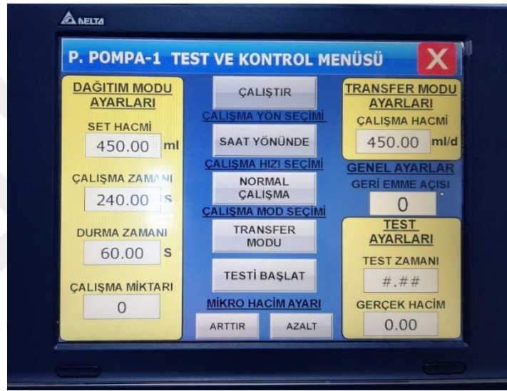
Şekil 4.18: Peristaltik pompa ayar ekranı.
