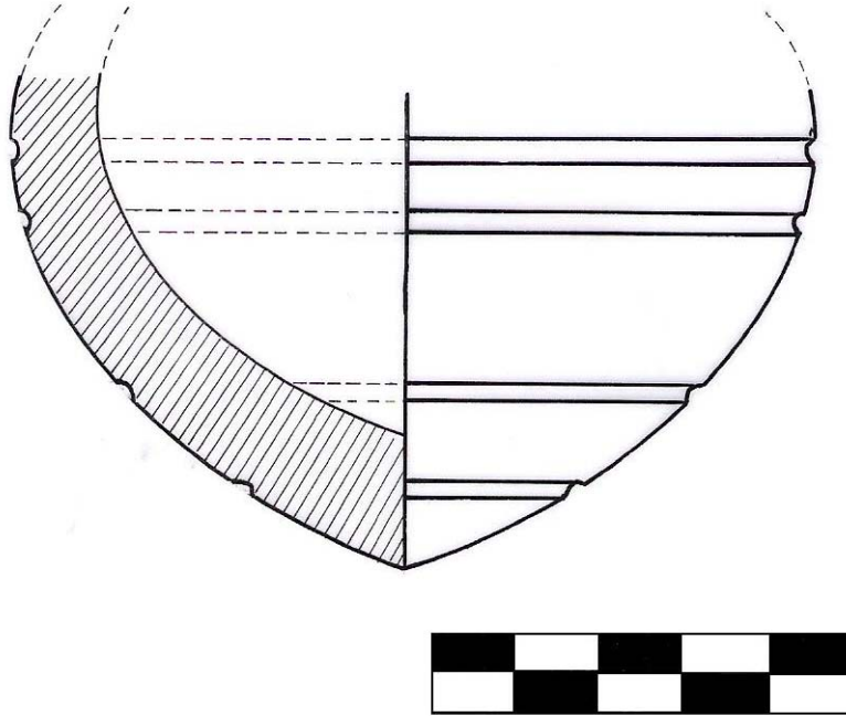
Çizim No: 22 Kürevî konik kap (Kız Kalesi)
