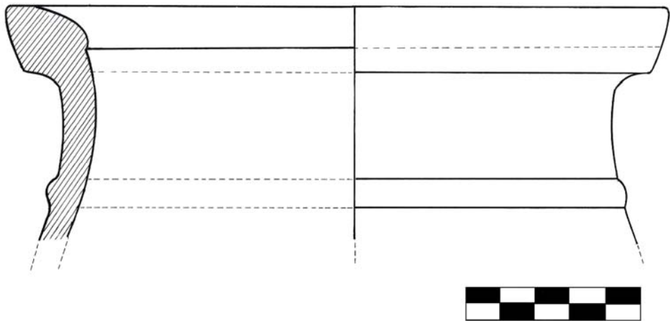
Çizim No: 19 Küp (Kız Kalesi)
