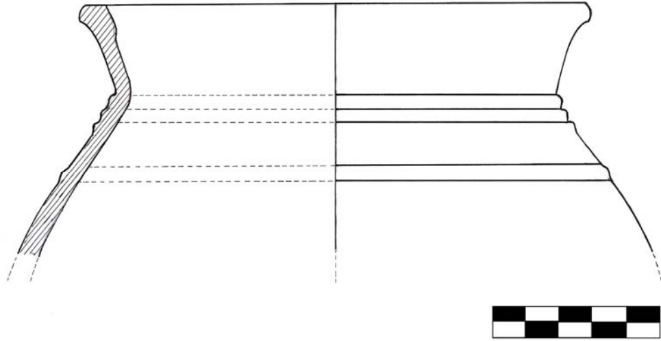
Çizim No: 6 Çömlek (Kız Kalesi)
