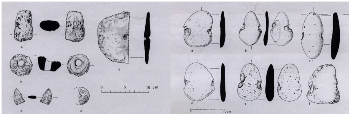
Resim 3.5. Çeşitli olta ağırlıklarına örnekler (Moore ve diğ. 2000:Res.7.13-14.)
