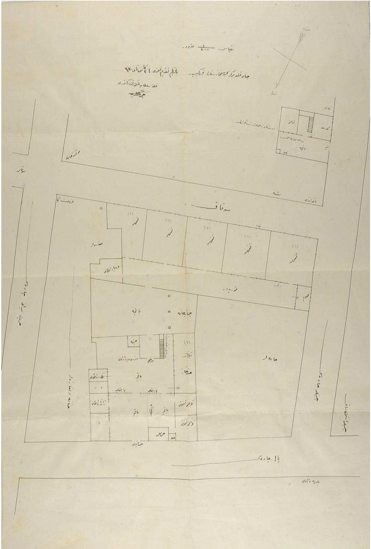
Şekil 3.1. 1921 Tarihli Kal'a-i Sultaniye Hapishanesinin Krokisi
