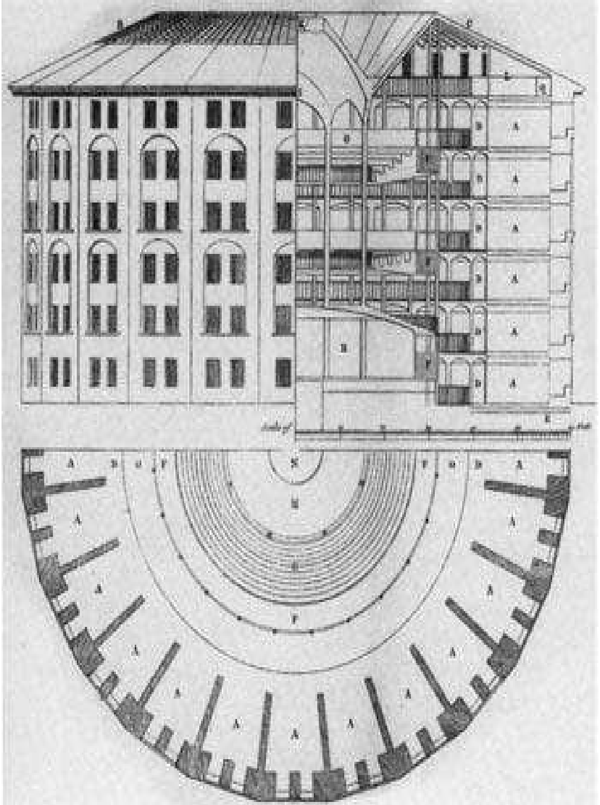
Ek.1. Panopticon Tarzı Hapishane Planı
