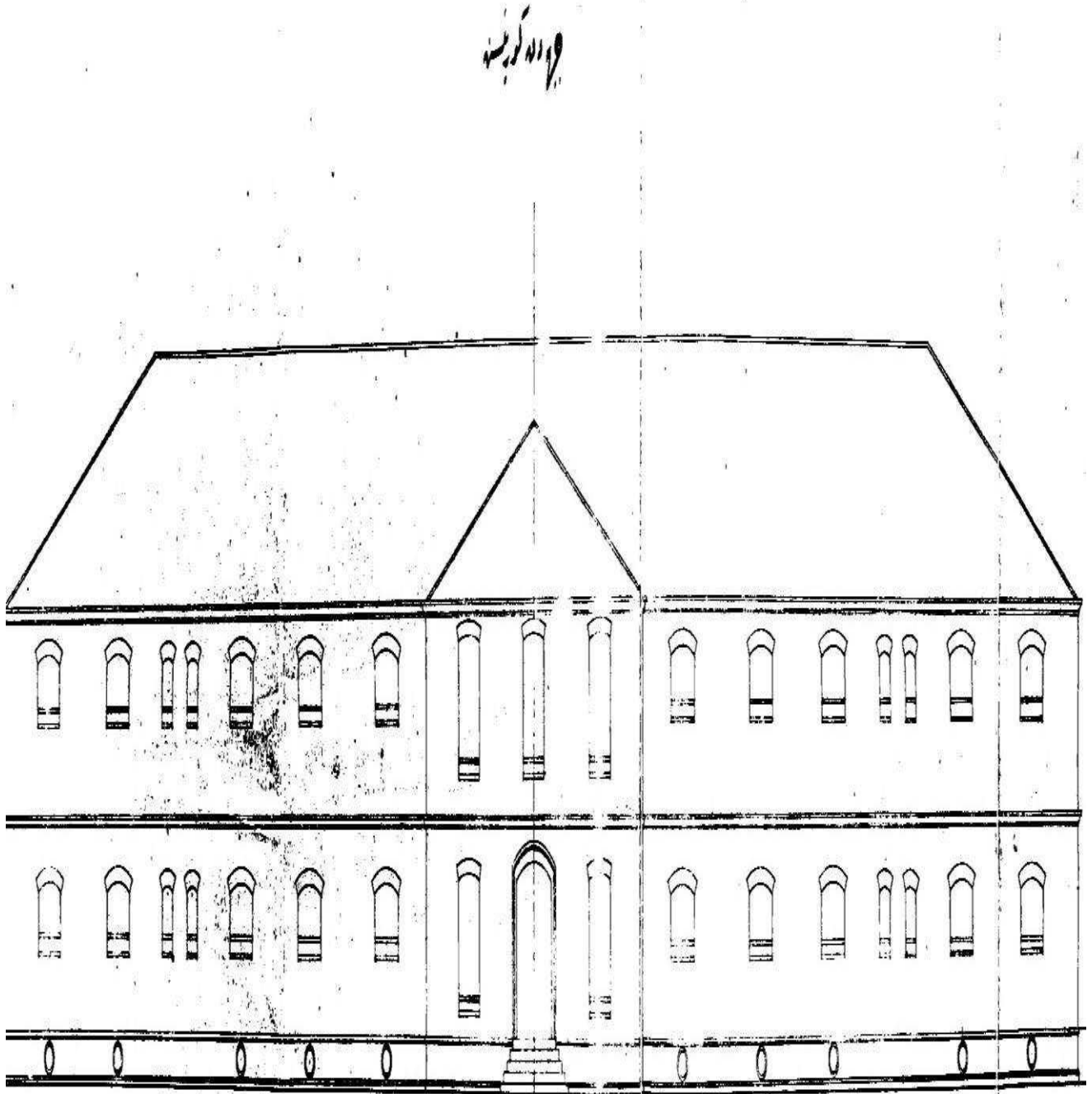
Ek.4. 1911 Yılında Numune Bahçe Dâhilinde Yapılması Düşünülen Kala-i Sultaniye Hapishanenin Dış Cepheden Görünüşü
