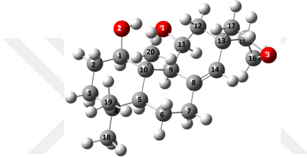
Şekil 6.9: Pimaran bileşiği atom numaralandırma.
