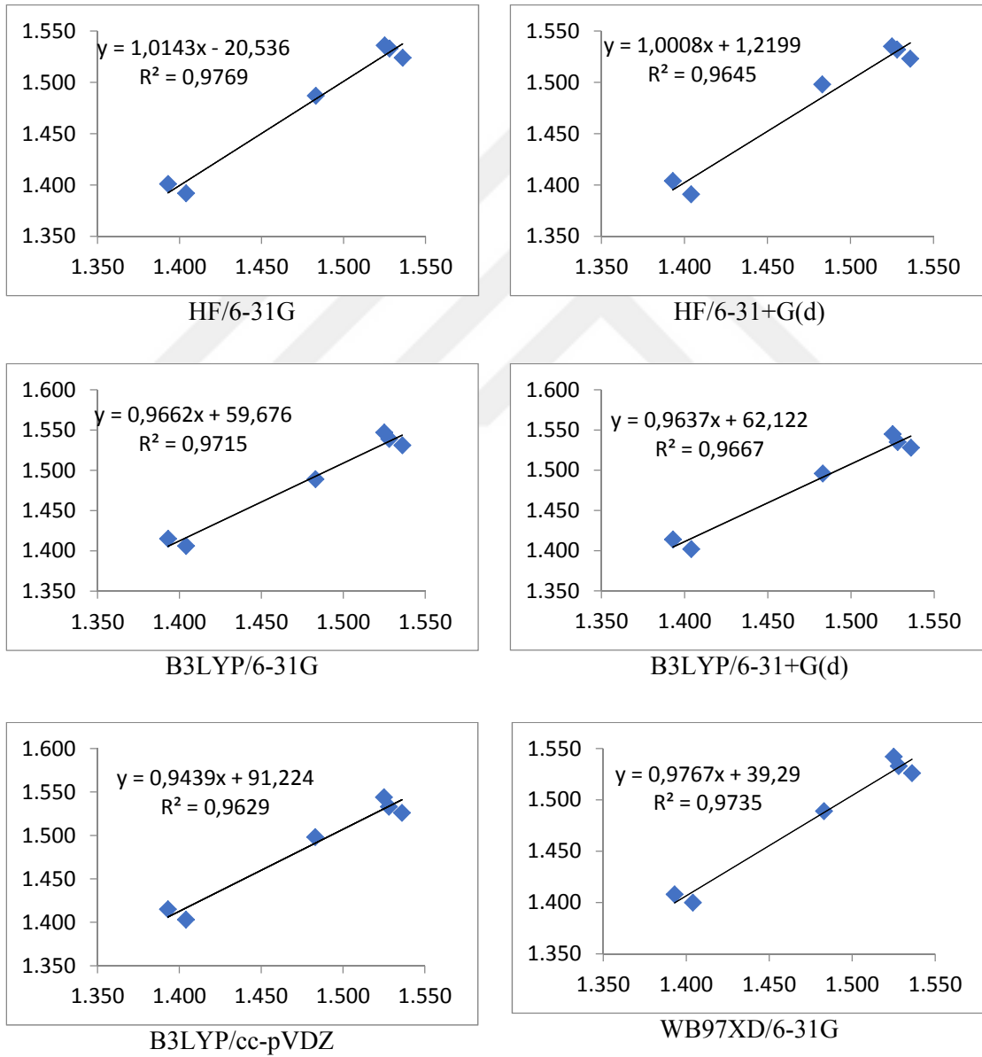
Şekil 6.2: Abietan/ deneysel karşı teorik bağ uzunlukları (Å) korelasyon grafikleri.
