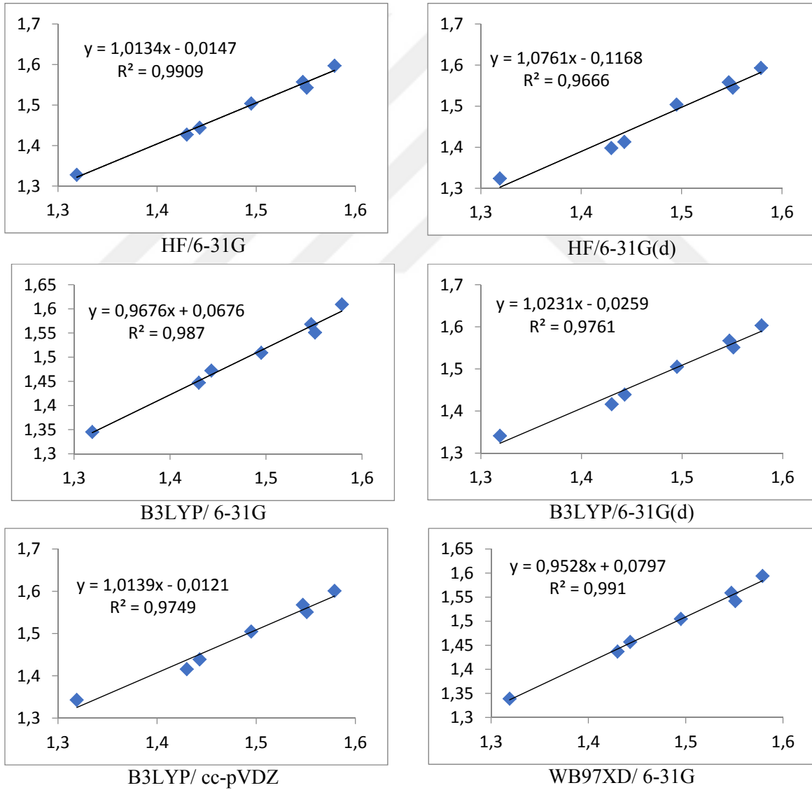
Şekil 6.10: Pimaran/ deneyselle karşı teorik bağ uzunlukları (Å) korelasyon grafikleri.
