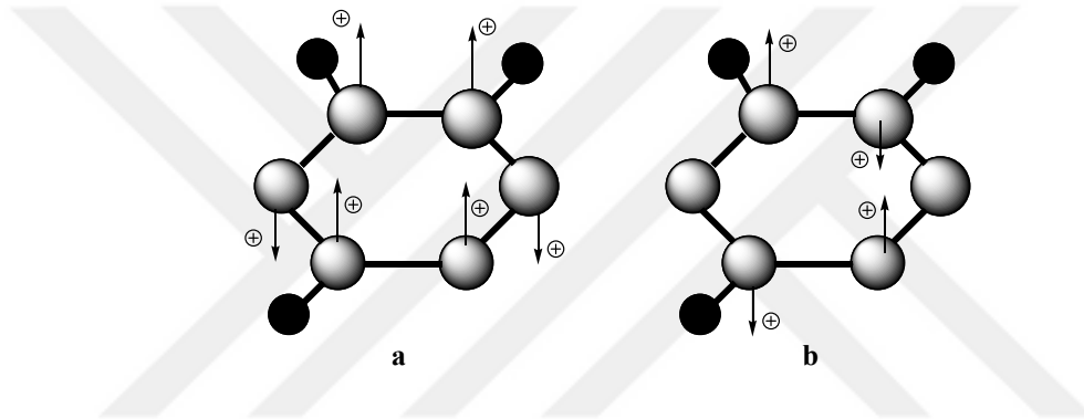
Şekil 3.9: a) Simetrik, b) Antisimetrik halka burulması
