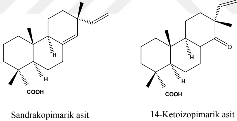
Şekil 1.11: Bazı Pimaranlar.
