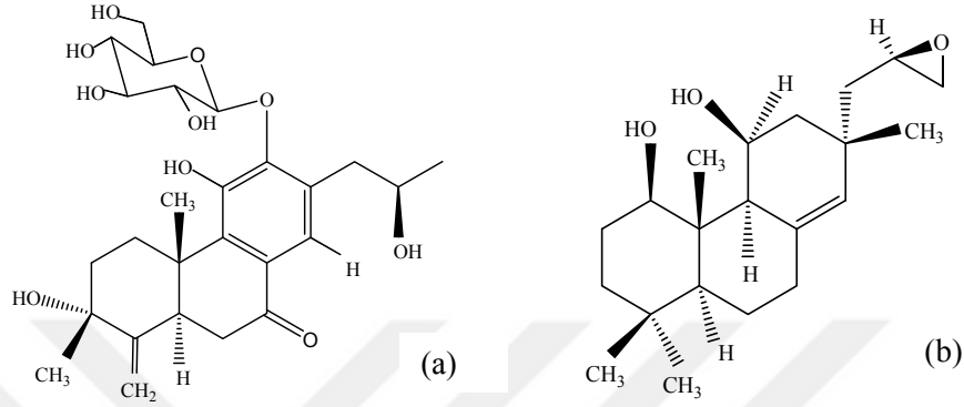
Şekil 5.1: a) IUPAC Adı: (3 R ,16 R )-12-O- \beta -D- glukopiranosil-3,11,16-trihidroksi-17(15 \rightarrow 16),18(4 \rightarrow 3)- dia-beo -4(19),8(9),11(12),13(14)-abietatetraen-7-on, Kısa adı: Szemaoneoid A, b) IUPAC Adı: 15 R ,16-epoksi- 8(14)-izopimaren-1 \beta ,11 \beta -diol, Kısa adı: Leucophleoksol bileşiklerinin çizgi gösterimi.
