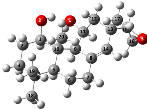
Şekil 6.12: Pimaran bileşiği IR atom numaralandırma.
