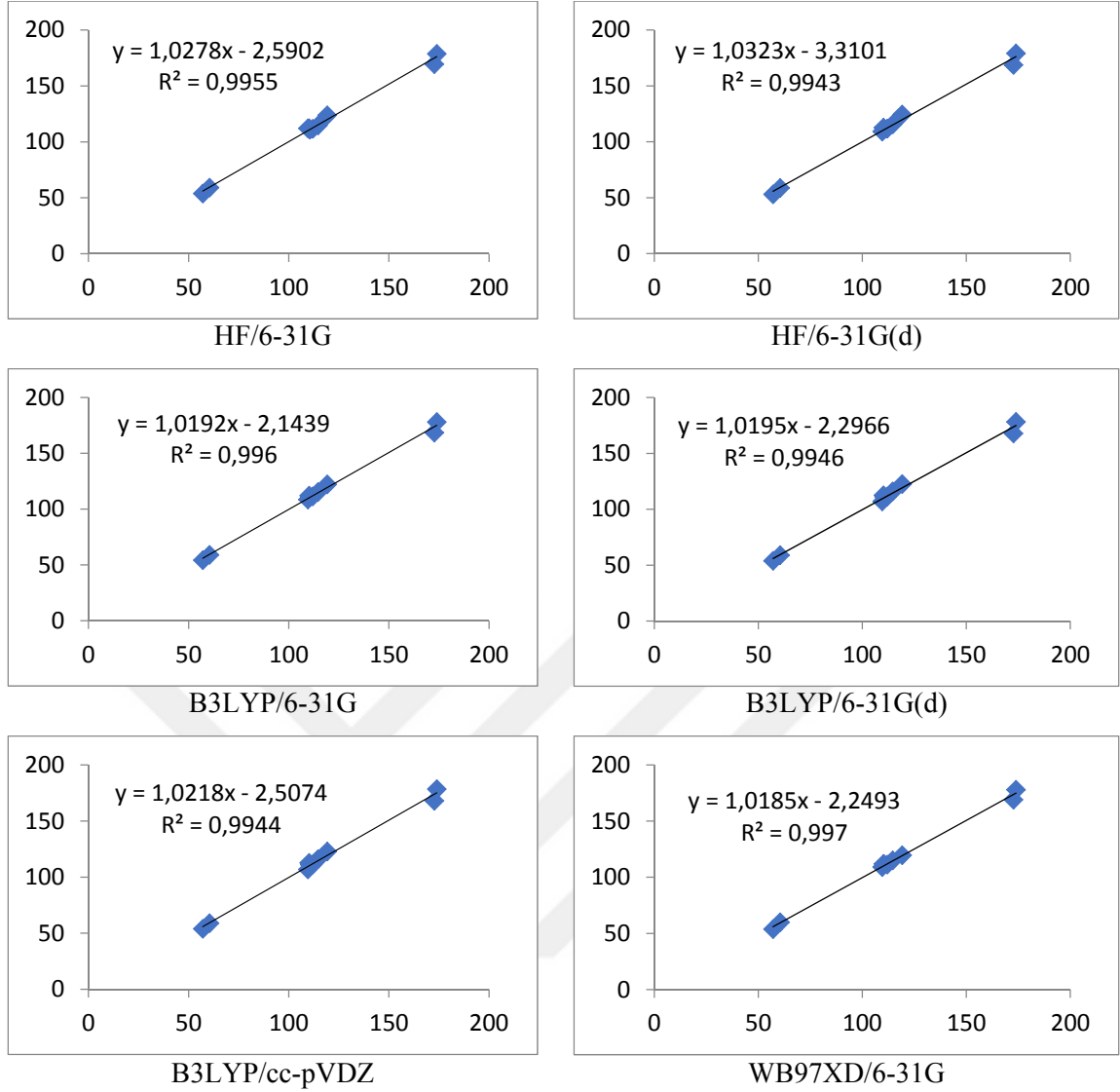
Şekil 6.11: Pimaran/ deneysel karşı teorik bağ ve dihedral açıları (°) korelasyon grafikleri.
