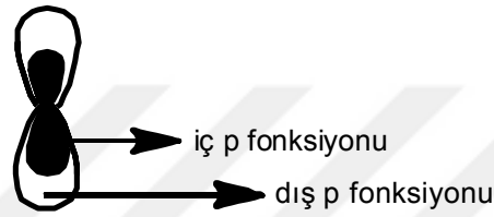
Şekil 2.1: Atomik p orbitali.
