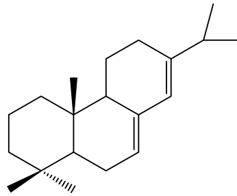
Şekil 1.4: Abietan iskeleti.
