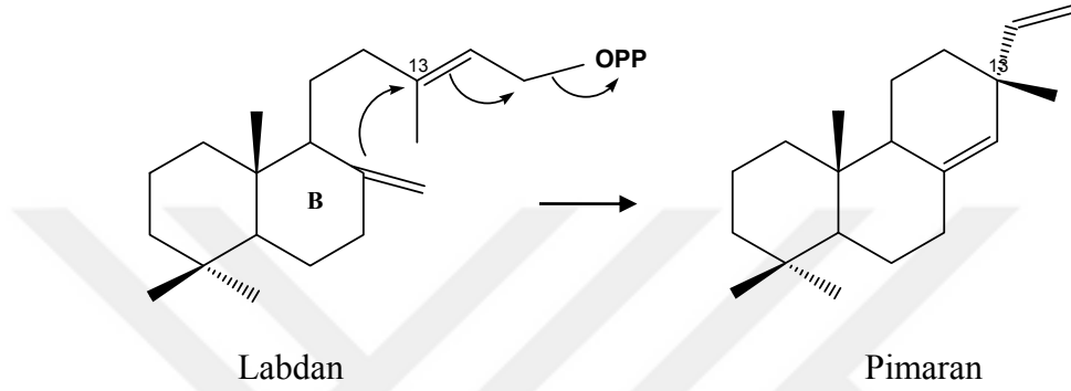
Şekil 1.10: Pimaranların oluşumu.
