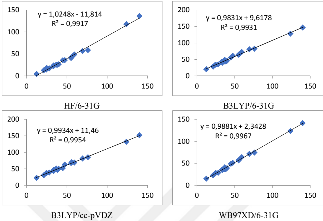
Şekil 6.13: Pimaran/deneysele karşı teorik 13 C-NMR kimyasal kayma değerleri korelasyon dağılım grafikleri.
