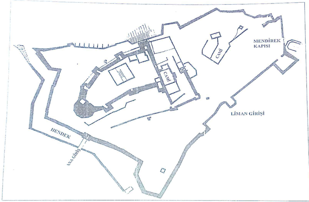
Bozcaada Kalesi planı
