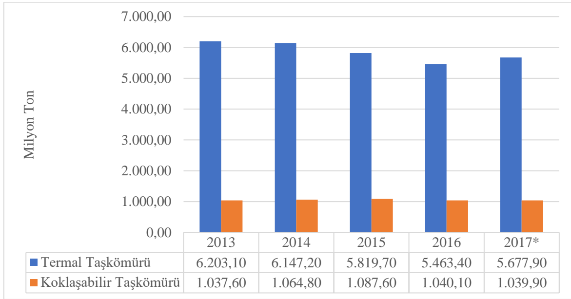
Şekil 2: Dünya Taşkömürü Üretiminin Yıllara Göre Değişimi
