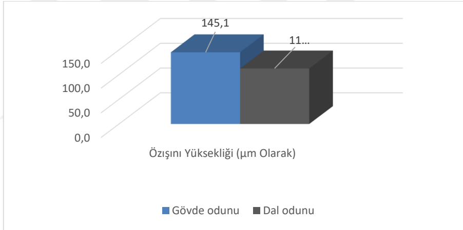
Şekil 25: Pinus brutia gövde ve dal odununda özişını yüksekliği (µm olarak).
