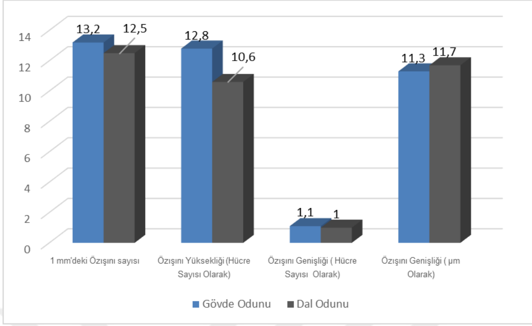
Şekil 28: Alnus glutinosa gövde ve dal odunu mm'deki özışını sayısı, özışını yüksekliği (hücre sayısı olarak), özışını genişliği (hücre sayısı ve µm olarak).
