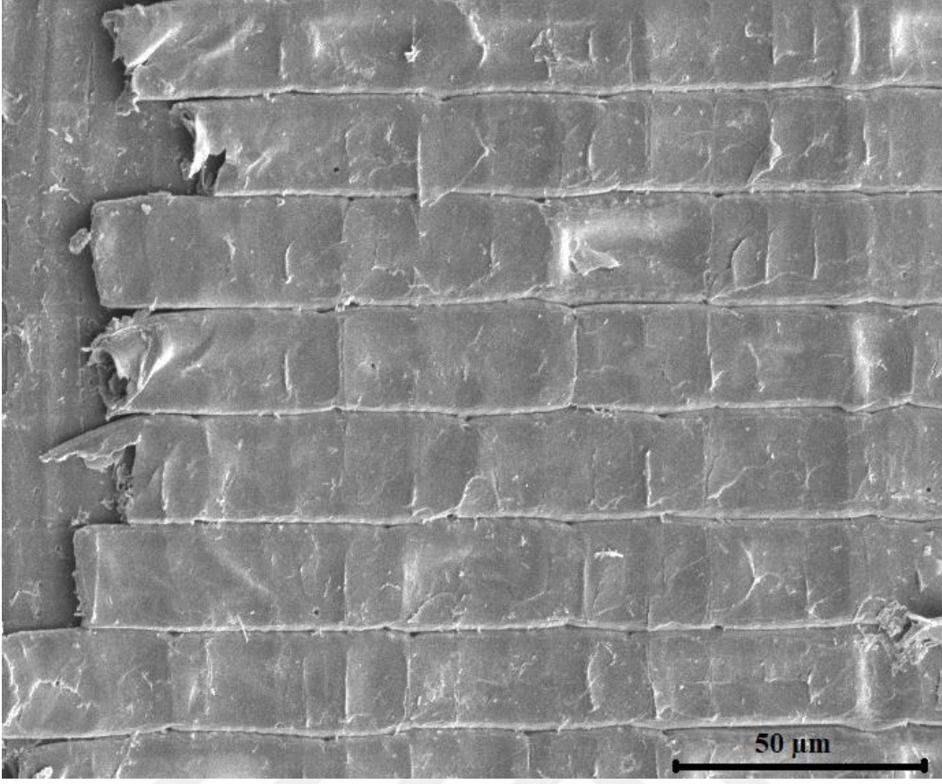
Şekil 11: Alnus glutinosa subsp. glutinosa dal odunu radyal kesiti. Yatık özışımı hücreleri.
