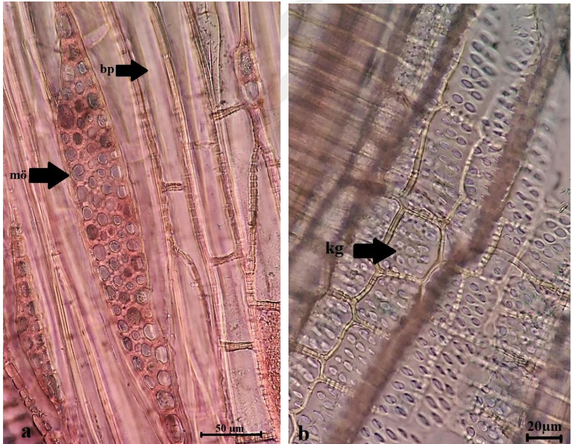
Şekil 15: Juglans regia gövde odunu teğet kesiti (a): multiseri özışınında paranzim hücreleri (mö), boyuna paranzim hücreleri (bp) ve radyal kesiti (b): trahe-paranzim hücresi karşılaşma yeri geçitleri (kg).
