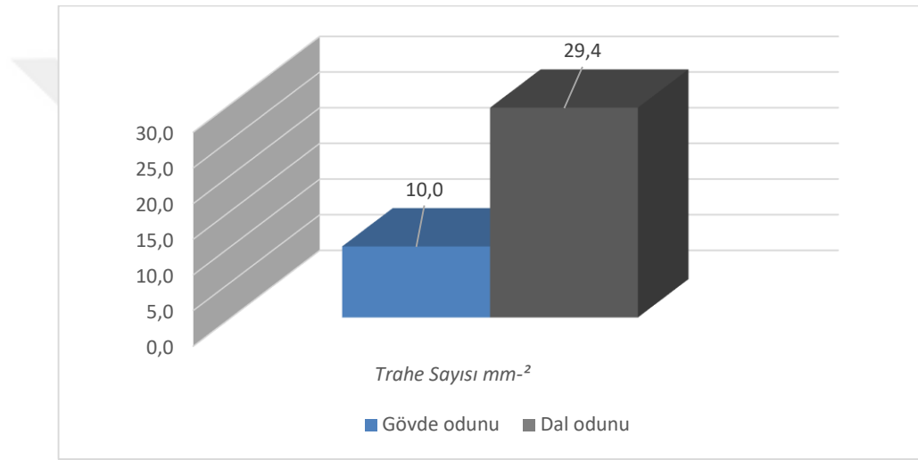
Şekil 30: Juglans regia gövde ve dal odununda \text{mm}^2 'deki trahe sayıları.
