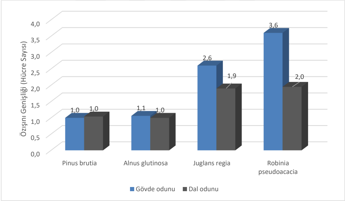
Şekil 41: İncelenen türlerin özışını genişlikleri (hücre sayısı olarak).
