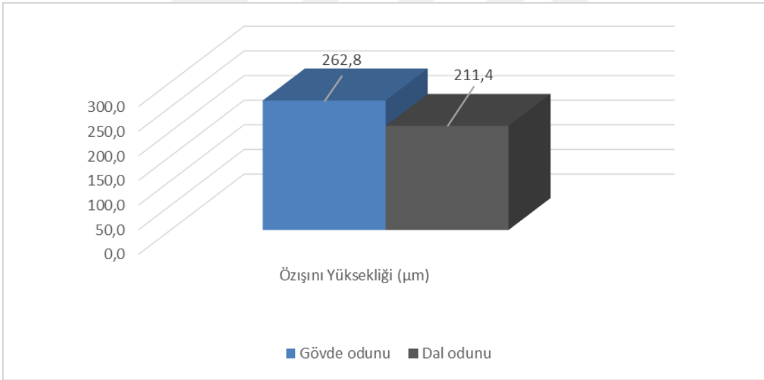
Şekil 29: Alnus glutinosa gövde ve dal odunu özışını yüksekliği (µm olarak).
