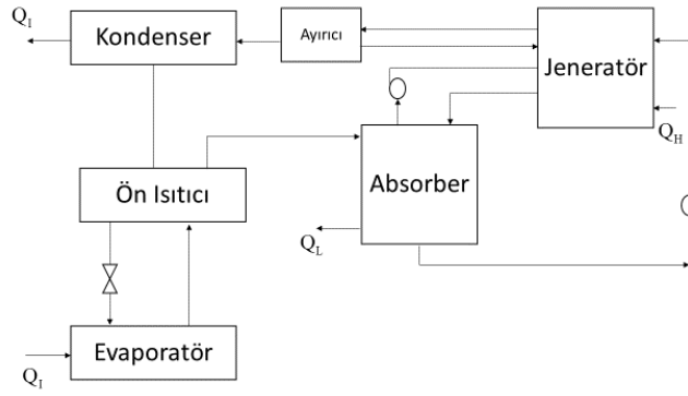
Şekil 1.4 GAX'lı Absorpsiyonlu Soğutma Çevrimi
