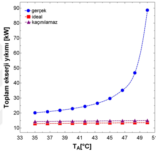
Şekil 3.17 Absorber sıcaklığı ile gerçek, ideal ve kaçınılmaz şartlar altındaki toplam ekserji yıkımlarının değişimi
