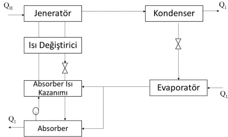
Şekil 1.5 Absorber-ısı Korunumlu Absorpsiyonlu Soğutma Çevrimi
