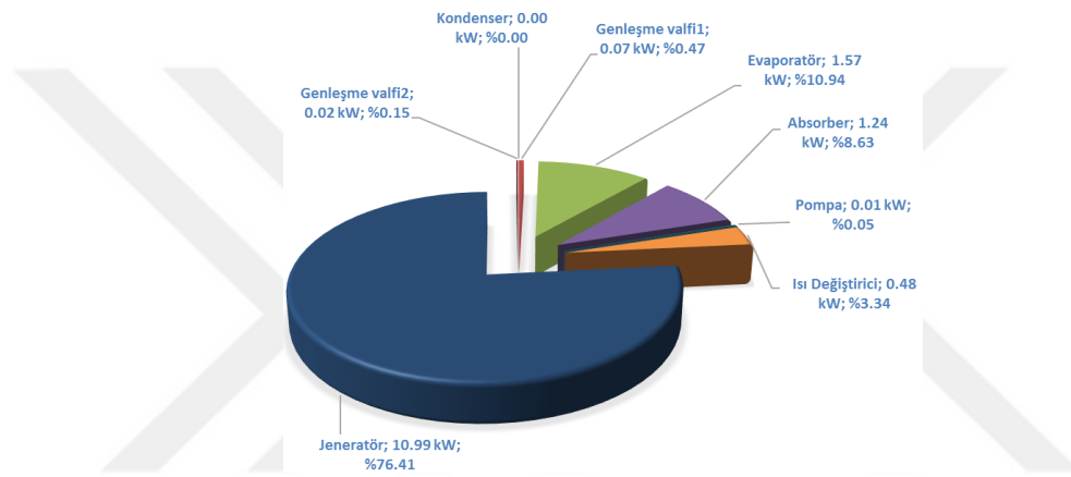
Şekil 3.22 Komponentlerin içsel ekserji yıkımlarının yüzde dağılımları
