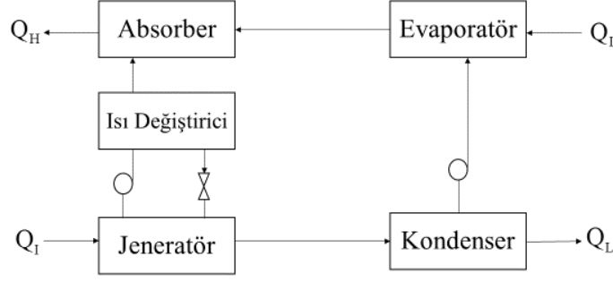
Şekil 1.2 Absorbsiyonlu Isı Yükselticileri
