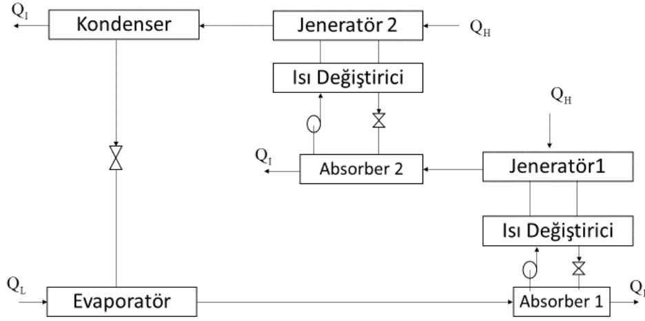
Şekil 1.6 Yarım Kademeli Absorpsiyonlu Soğutma Çevrimi
