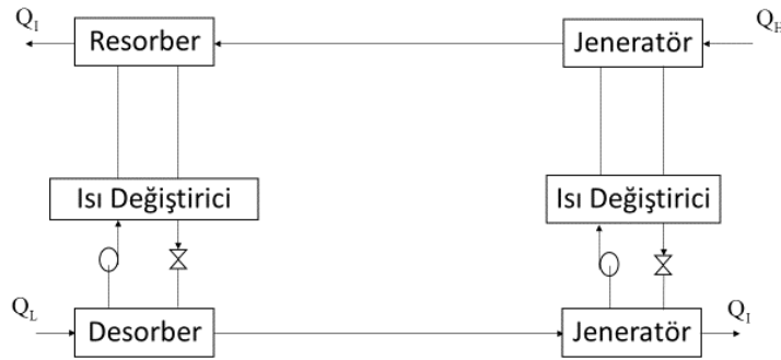
Şekil 1.7 Kombine Buhar Absorpsiyon Sıkıştırma Çevrimi
