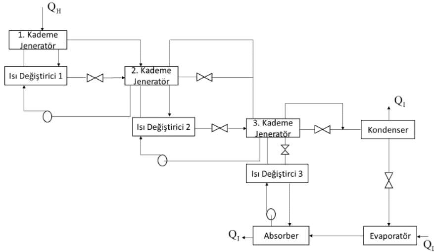
Şekil 1.3 Çok Kademeli Absorbsiyonlu Soğutma Sistemi
