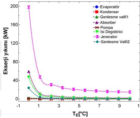
Şekil 3.8 Evaporatör sıcaklığı ile komponentlerdeki ekserji yıkımlarının değişimi
