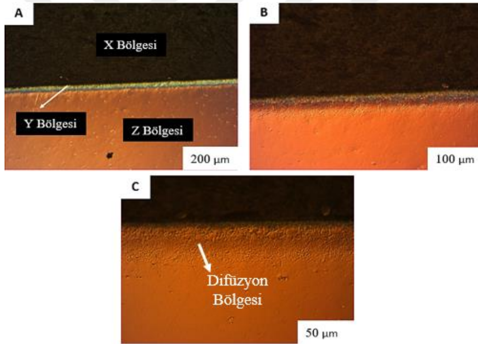
Şekil 6.2: 950 °C'de 4 saat boyunca borlamaya tabi tutulan numunelerin, a) 50X büyütme, b) 100X büyütme ve c) 200X büyütmelemlerden alınmış görüntüleri.
