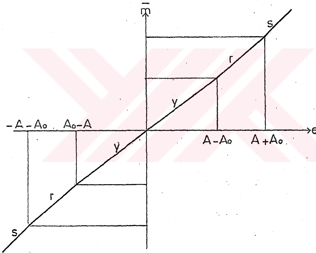
Şekil 3.30. Testere dişi şeklinde salınım sinyali uygulandığında m - e karakteristiği ( |A| > 2|A_0| olması hali)
