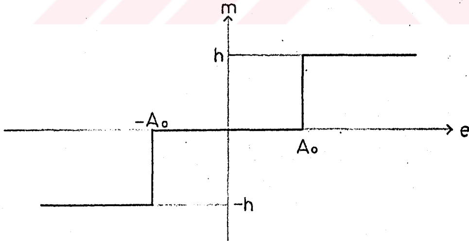
Şekil 1.4. Ölü bölgeyi çift yönlü röle karakteristiği
