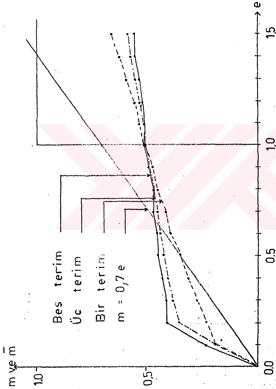
Şekil 4.64. Şekil 1.4'de gösterilen orijinal karakteristiğe, yaklaştırılmak istenen lineer karakteristiğin eğimi olan K=0.7 için 4.2.4. bölümünde bulunan optimum salınım sinyallerinin uygulanarak elde edilen \bar{m} ortalama çıkış sinyalleri.
