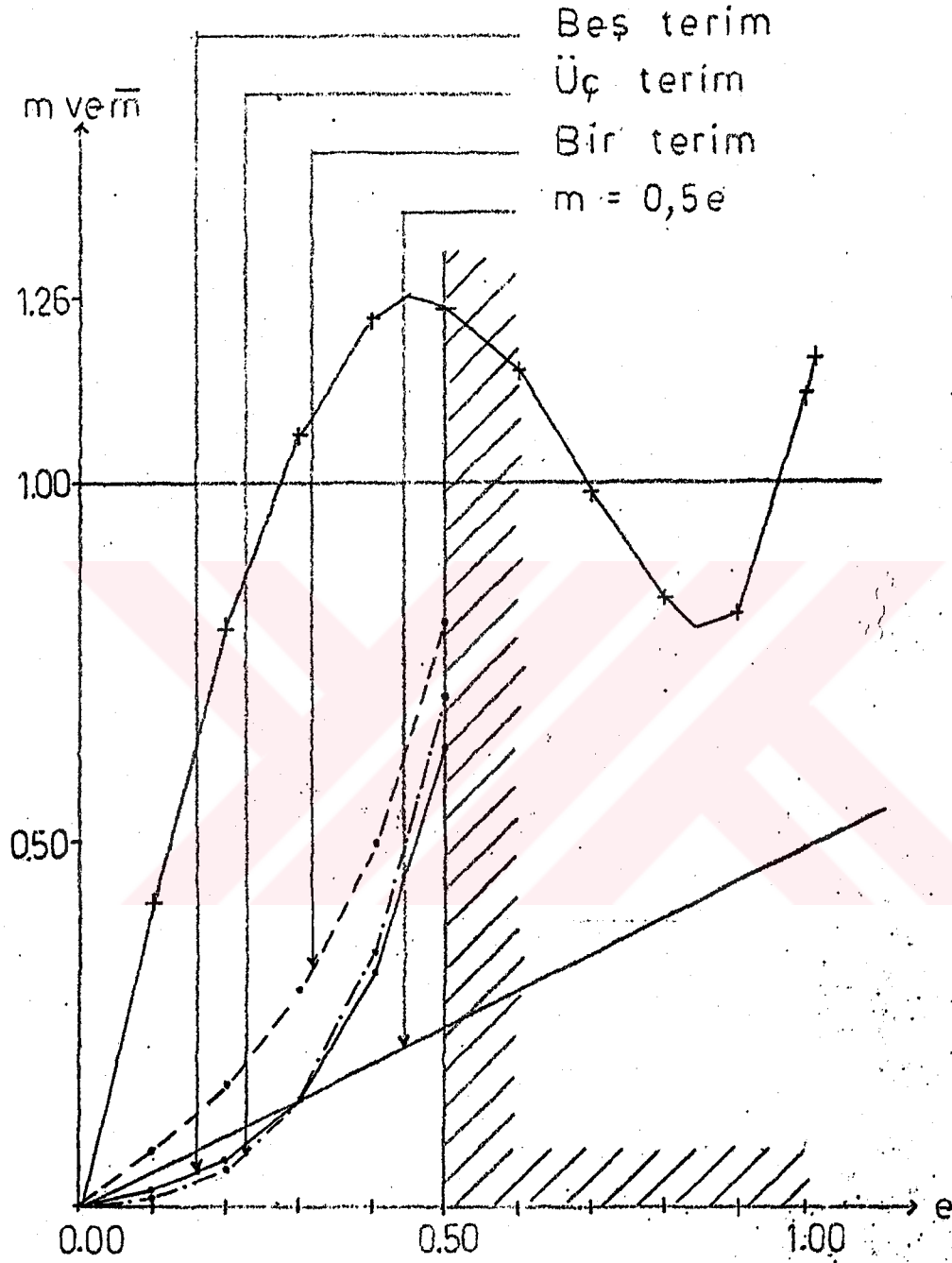
Şekil 4.9. Şekil 4.1'de gösterilen karakteristiğe uygulanan salınım sinyali, neticesinde yaklaştırılmak istenen lineer karakteristiğin eğimi K=0.5 için Fourier serisinden ilk bir, üç ve beş terim alınarak elde edilen m ortalama çıkış sinyali
