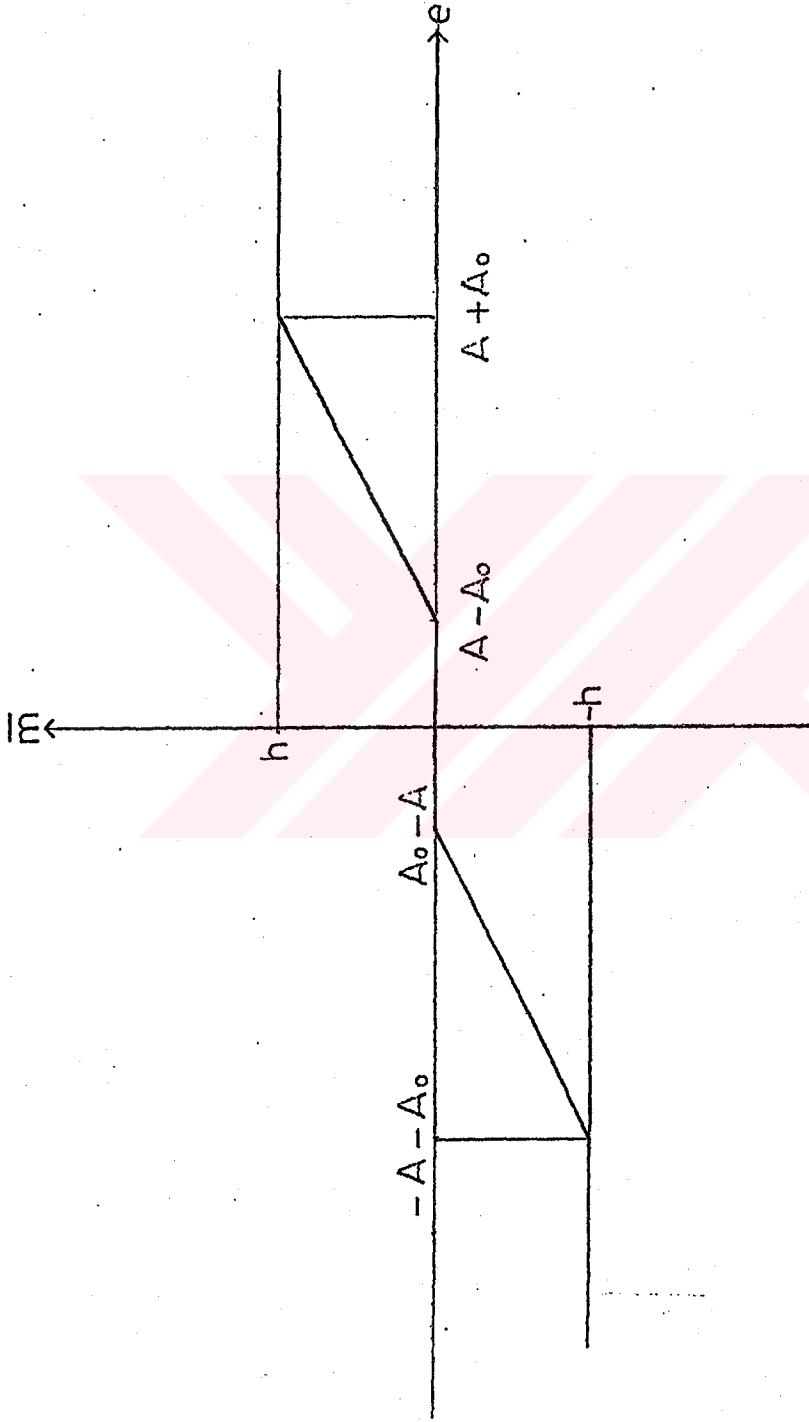
Şekil 3.18. Kare seklinde salınım sinyali uygulandığında \bar{m} -e karakteristiği (|A| > 2|A_0| \text{ olması halinde})
