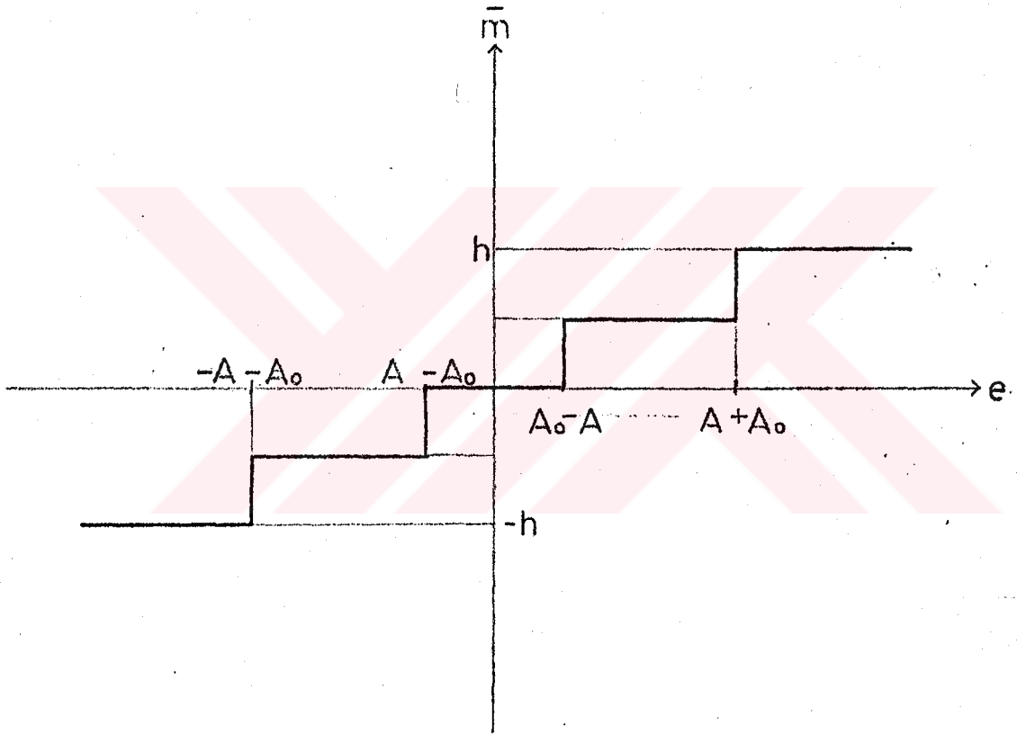
Şekil 3.52. Kare şeklinde salınım sinyali uygulandığında \bar{m} - e karakteristiği ( 2|A_0| > |A| > |A_0| olması hali)
