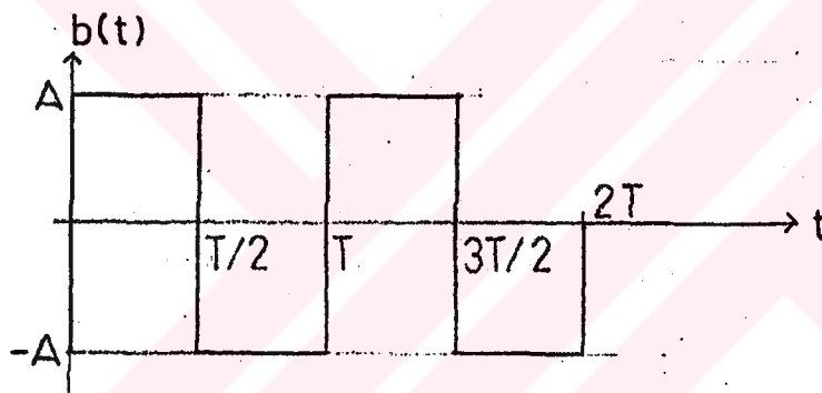
Şekil 1.6. Kare salınım sinyali
