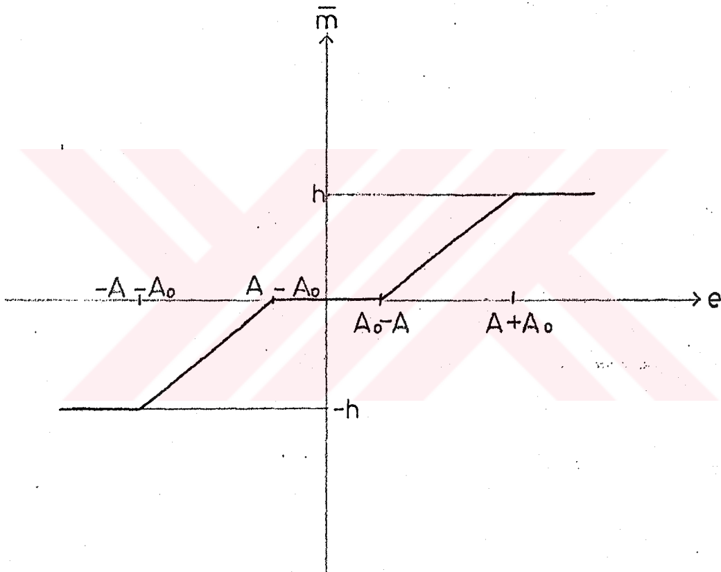
Şekil 3.44. Testere dişi şeklinde salınım sinyali uygulandığında m - e karakteristiği ( |A_0| > |A| olması hali)
