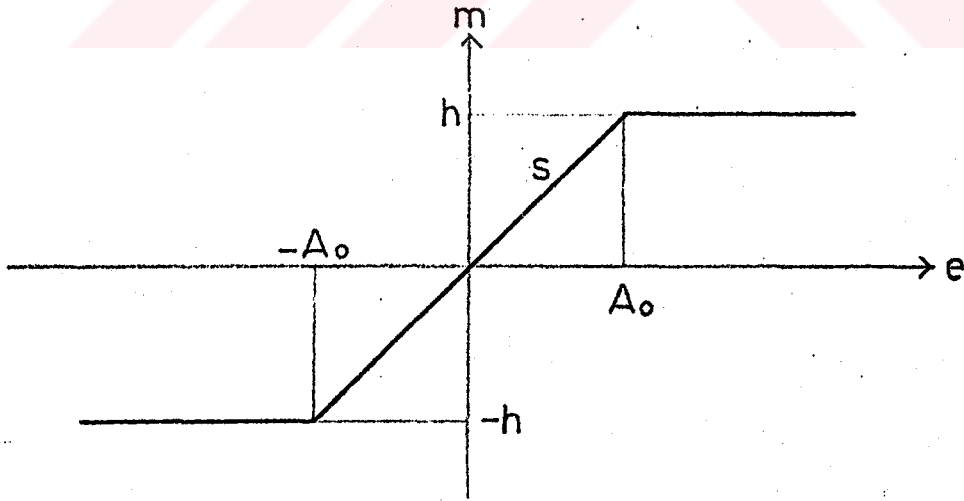
Şekil 1.2. Doyma eğrisi
