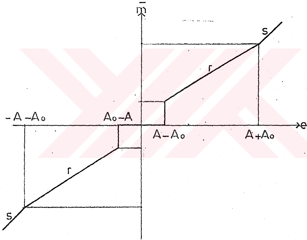
Şekil 3.36. Kare şeklinde salınım sinyali uygulandığında m - e karakteristiği ( |A| > 2|A_0| olması hali)
