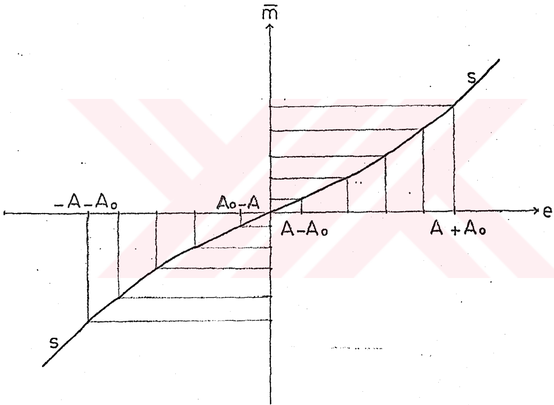
Şekil 3.42. Sinüzoidal şekilde salınım sinyal uygulandığında m-e karakteristiği ( |A| > 2|A_0| olması hali),
