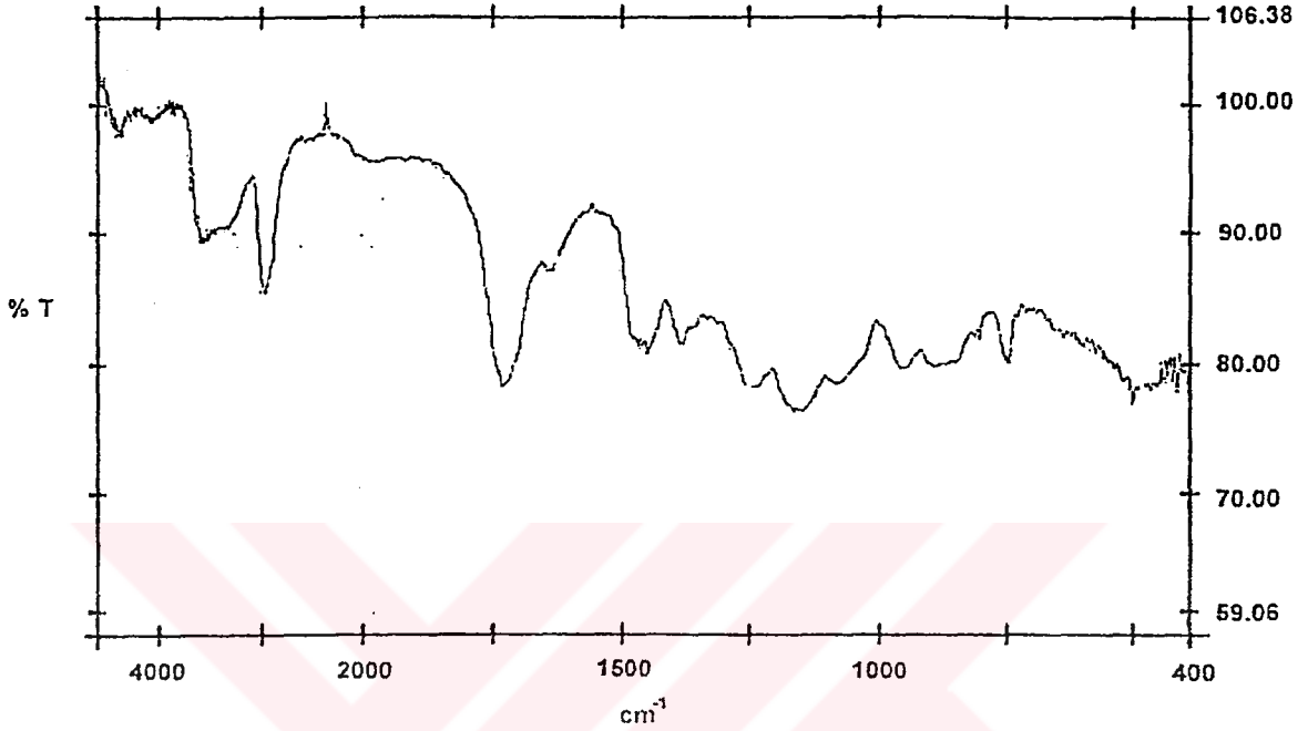
Şekil 3.5. p(HEMA-co-MAH) mikrokürelerin FTIR spektrumu
