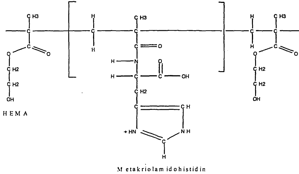
Şekil 3.3. p(HEMA-co-MAH) mikrotürelerin molekül formülü
