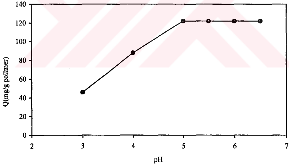
Şekil 3.9. Polimerik mikrokürelere adsorplanan Cu(II) miktarının pH ile deęişimi; MAH yükleme
