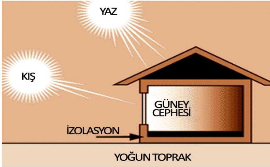
Şekil 2.3. Pasif Güneş Sistemi İçin Şematik Konumlandırma (http 9)
