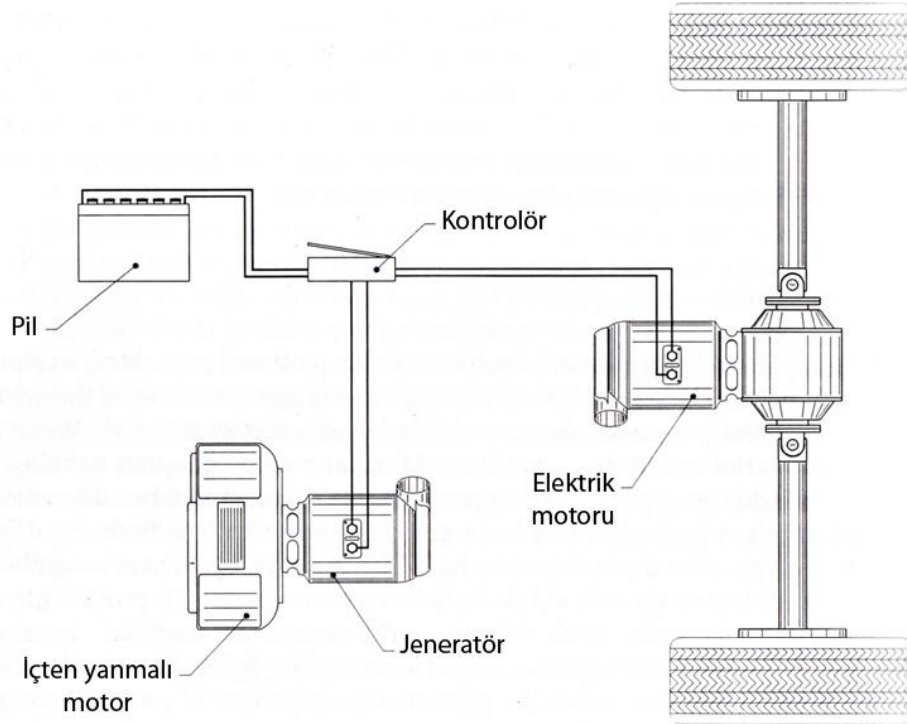
Şekil 4.4. Seri hibrit bir aracın hareket sisteminin şematik gösterimi (Riley 1994).
