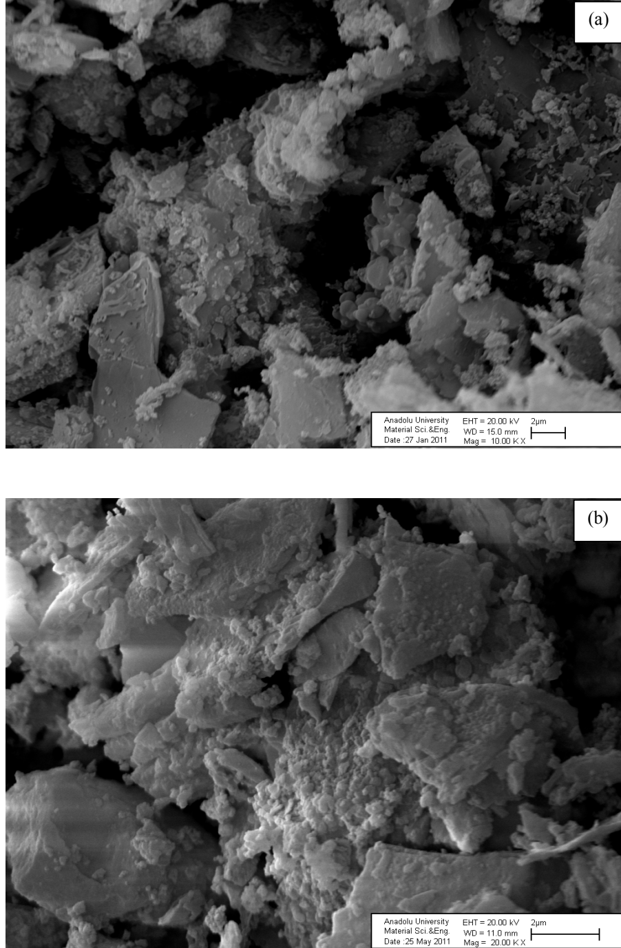
Şekil 5.28. MCM-48 malzemelerine ait SEM görüntüleri (a) HTS ve (b) HTS-%30TPA
