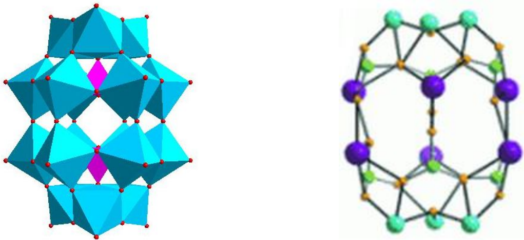
Şekil 3.2. Wells-Dawson yapısındaki heteropoli asit [191,192]
