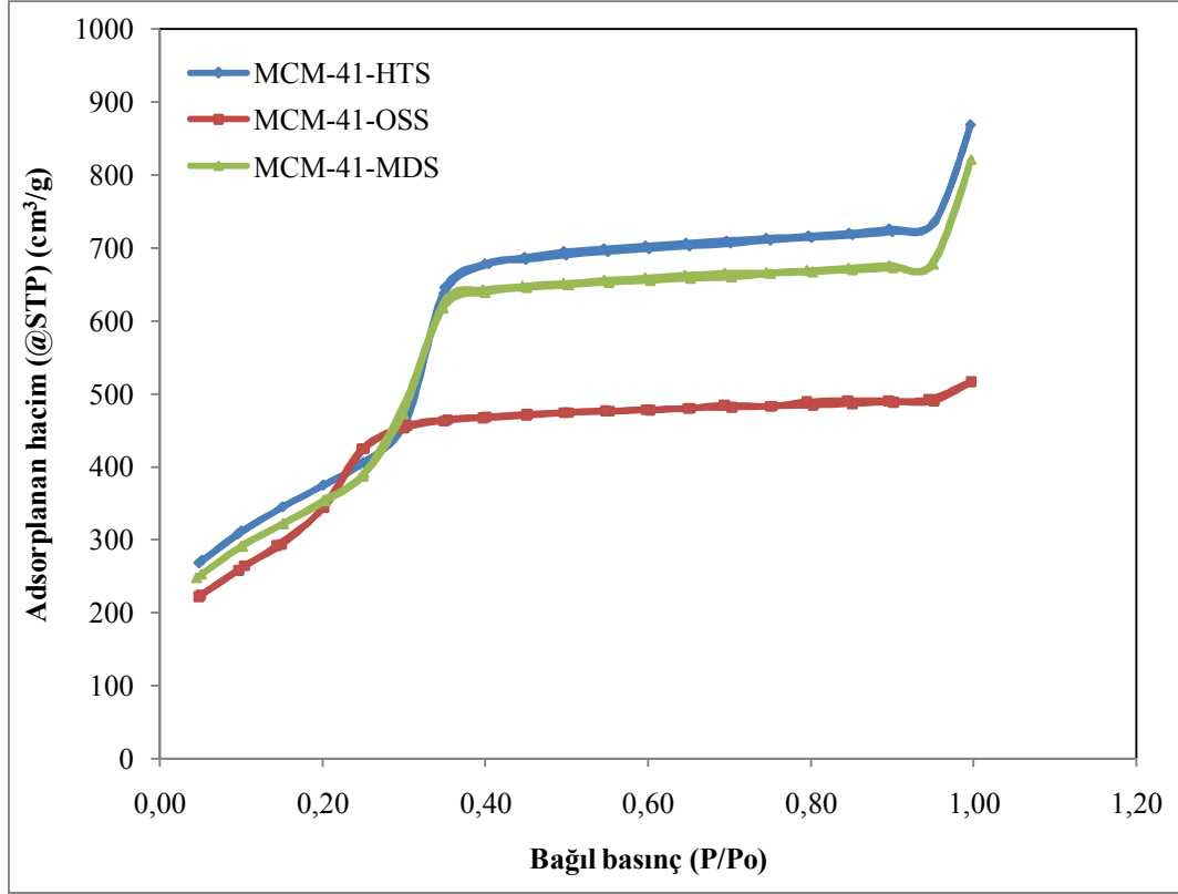
Şekil 5.5. HTS, OSS ve MDS metotları ile sentezlenen saf MCM-41 malzemelerinin azot adsorpsiyon/desorpsiyon izotermeleri
