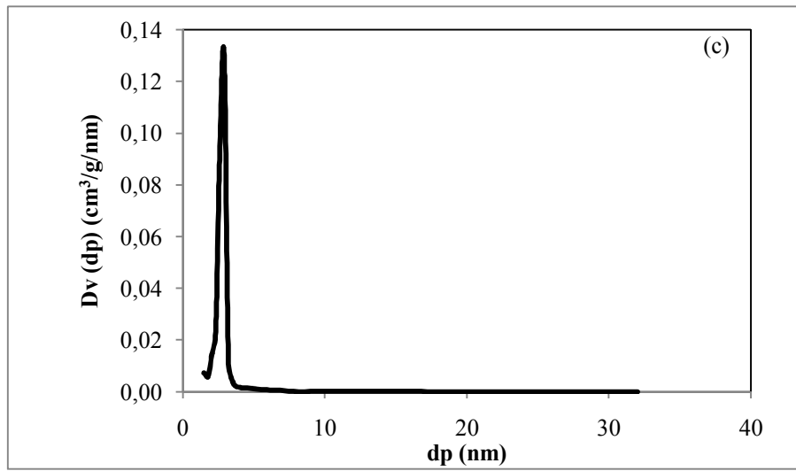
Şekil 5.6. (a) MCM-41-HTS, (b) MCM-41-OSS ve (c) MCM-41-MDS malzemelerinin gözenek boyut dağılımları
