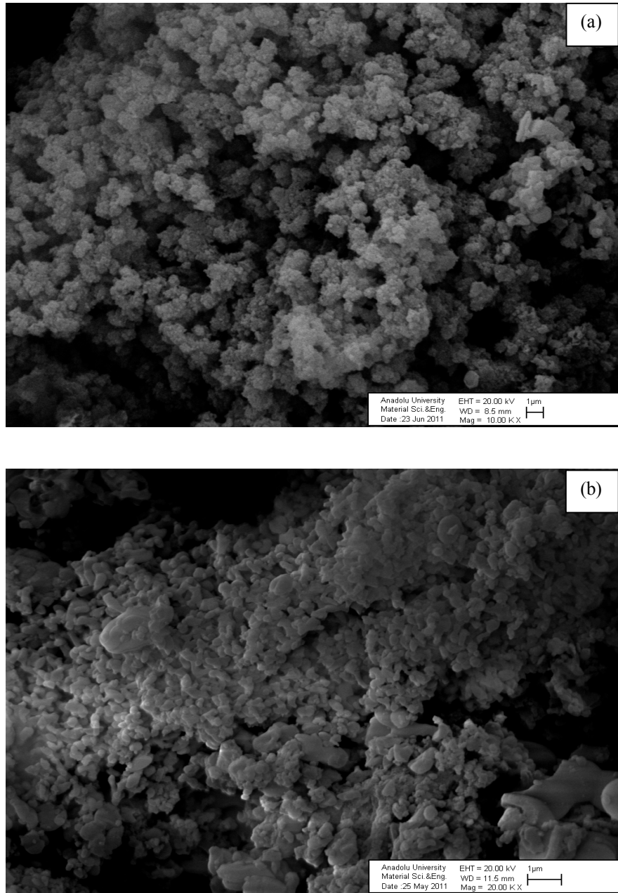
Şekil 5.30. MCM-48 malzemelerine ait SEM görüntüleri (a) MDS ve (b) MDS-%30TPA
