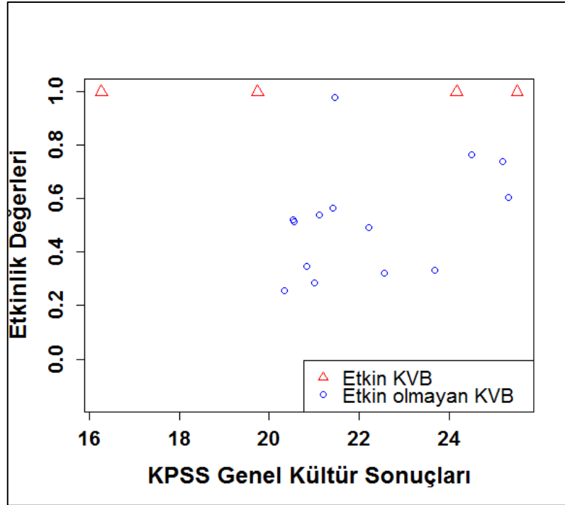
Şekil 4.4 Etkinlik - KPSS Genel Kültür Sonuçları Saçılım Grafiği
