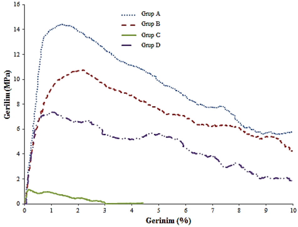
Şekil 4.23 Başlangıç köpük numunesi ile farklı yüzey işlemleri görmüş yaklaşık % 62.4 gözenek miktarına sahip Ti6Al4V alaşım köpüklerinin gerilim-gerinim eğrileri
