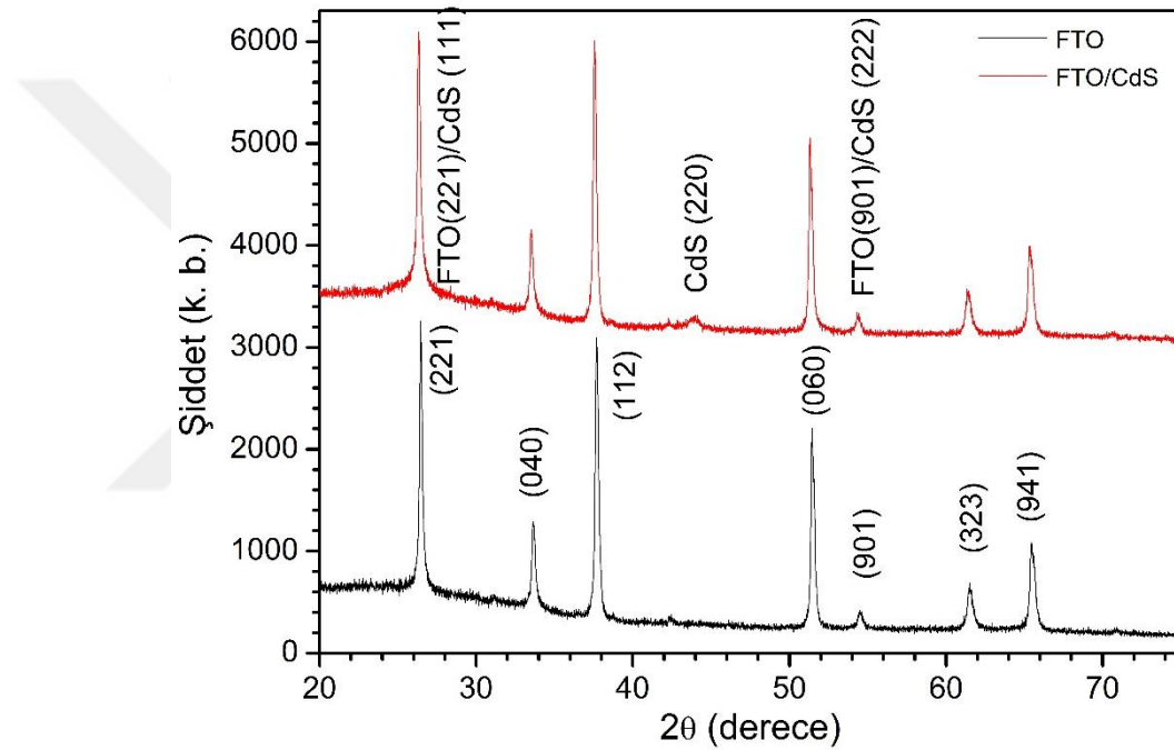
Şekil 4.4. FTO ve FTO/CdS filmlerine ait x-ışını kırınım desenleri.
