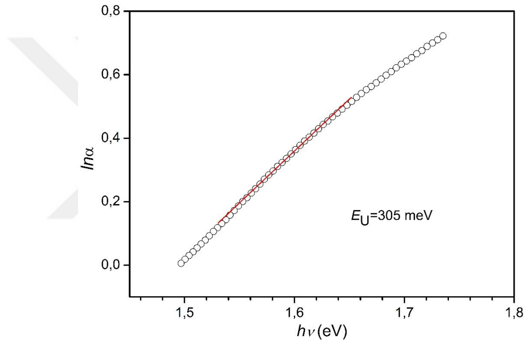
Şekil 5.17. Cam taban üzerine elde edilen CuO filminin \ln\alpha-h\nu grafiği.
