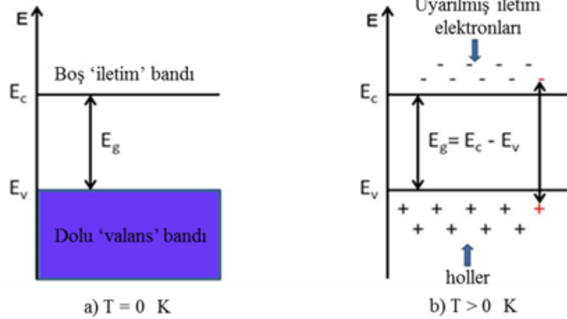
Şekil 2.2. Bir has yarıiletkenin a) T=0 \text{ K} 'de, b) T>0 \text{ K} 'de şematik enerji-bant diyagramı [50].
