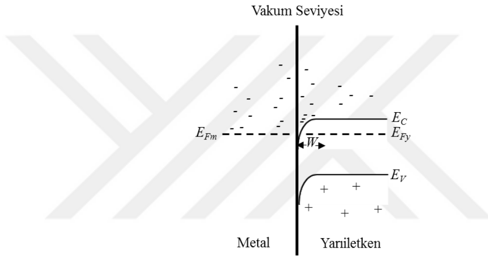
Şekil 8.2. Metal/n-tipi yarıiletken ohmik kontağın kontak oluşturduktan sonraki enerji bant diyagramı [95, 50].
