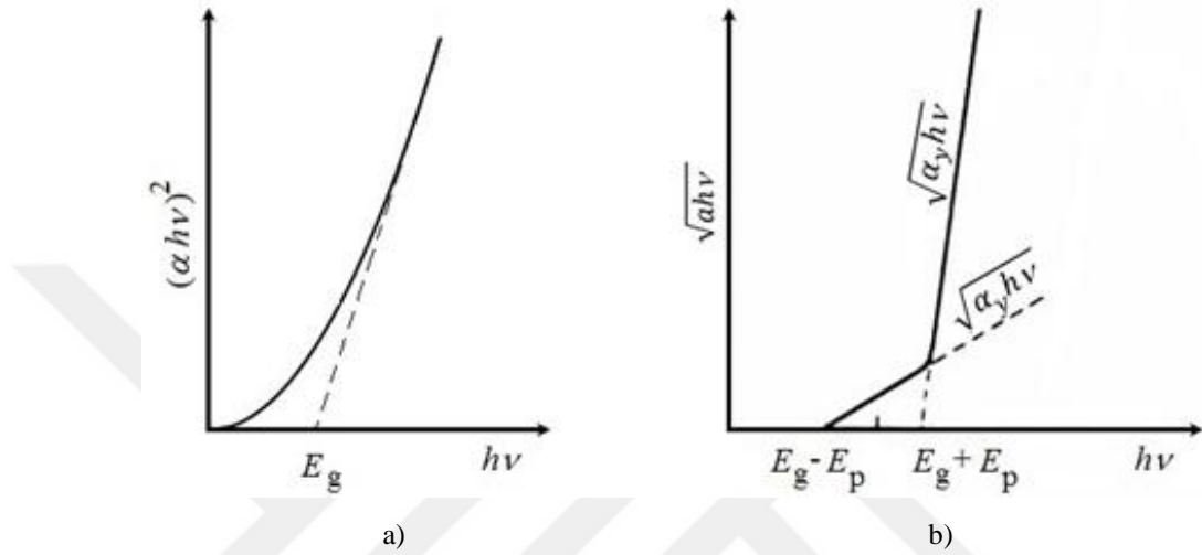
Şekil 5.6. a) Yarıiletkenlerde direkt b) indirekt bant geçişinin grafiksel gösterimi [67].
