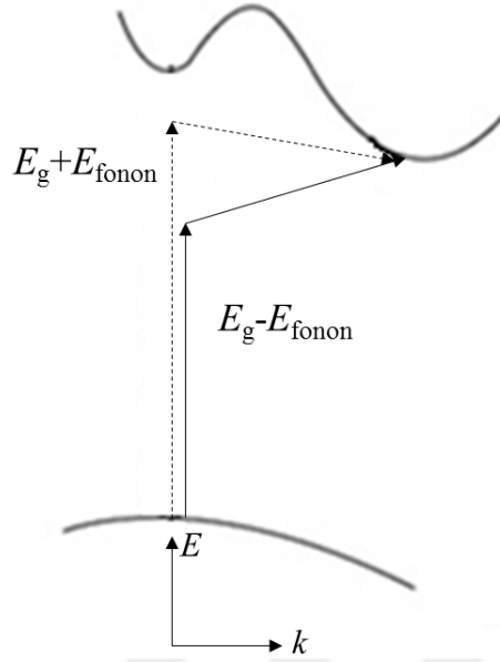
Şekil 5.5. Bir yarıiletkende indirekt bant geçişinin şematik gösterimi [67].
