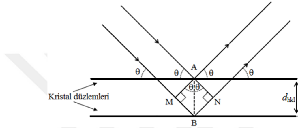
Şekil 4.2. X-ışınlarının kristal düzlemleri tarafından kırınımı [65].
