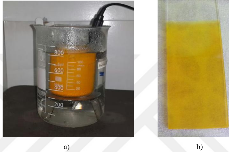
Görsel 3.1. a) CdS filmi oluşumunda kullanılan kimyasal reaksiyon banyosu. b) Cam taban üzerine elde edilen CdS filmi.
