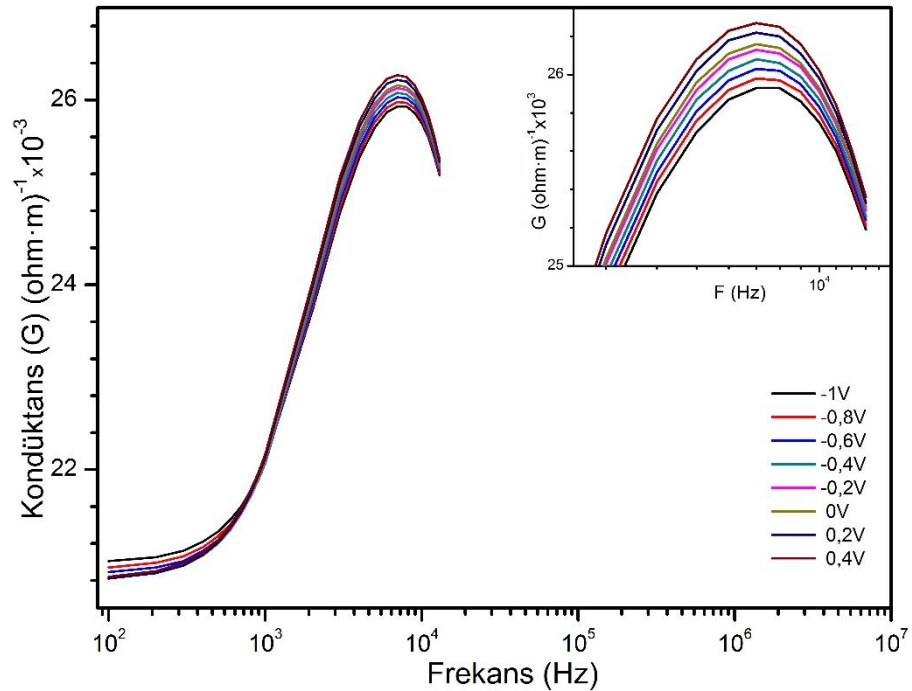
Şekil 8.17. FTO/n-CdS/Au yapısının farklı voltajlarda elde edilmiş kondüktans-frekans grafiği.
