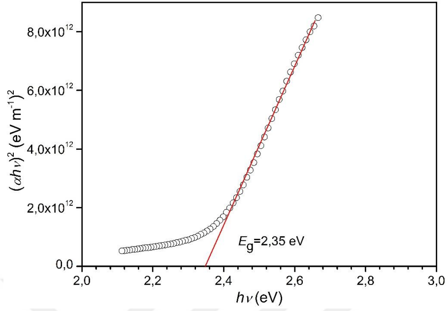
Şekil 5.12. FTO taban üzerine elde edilen CdS filminin (\alpha hv)^2-h\nu grafiği.
