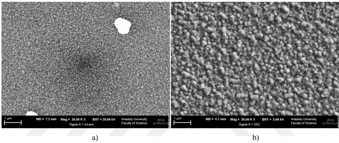
řekil 7.8. a) Cam taban ve b) FTO taban üzerine elde edilen CdS filmlerinin SEM görüntüleri.
