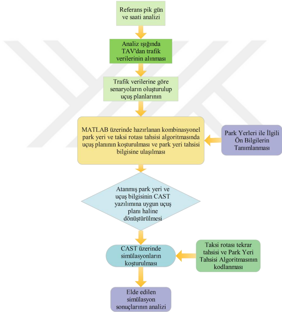
Şekil 6.10. Önerilen park yeri ve taksi rotası tahsisi modelinin sınanması sürecinde yapılan işlemler
