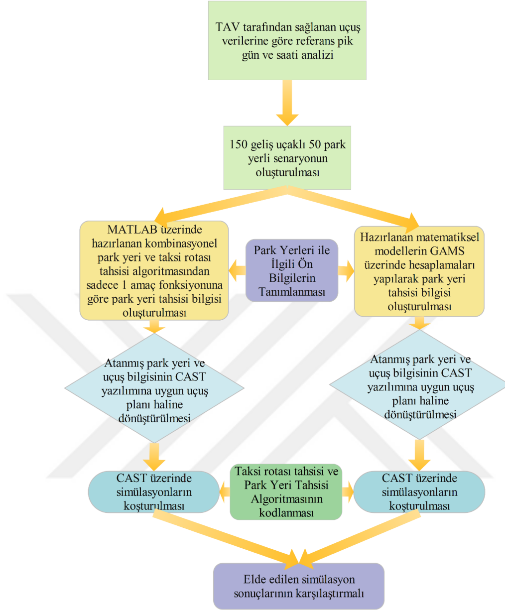
Şekil 6.9. Önerilen kombinasyonel park yeri taksi rotası tahsisi algoritması SA ve GAMS sonuçları karşılaştırmasının yapılması için izlenen adımlar
