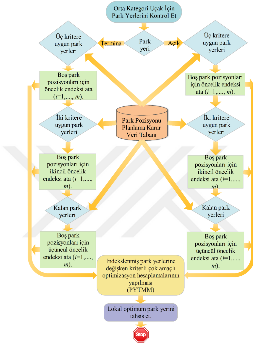
Şekil 3.2. "Alt-Algorithm 1": Park yeri tahsisi algoritması
