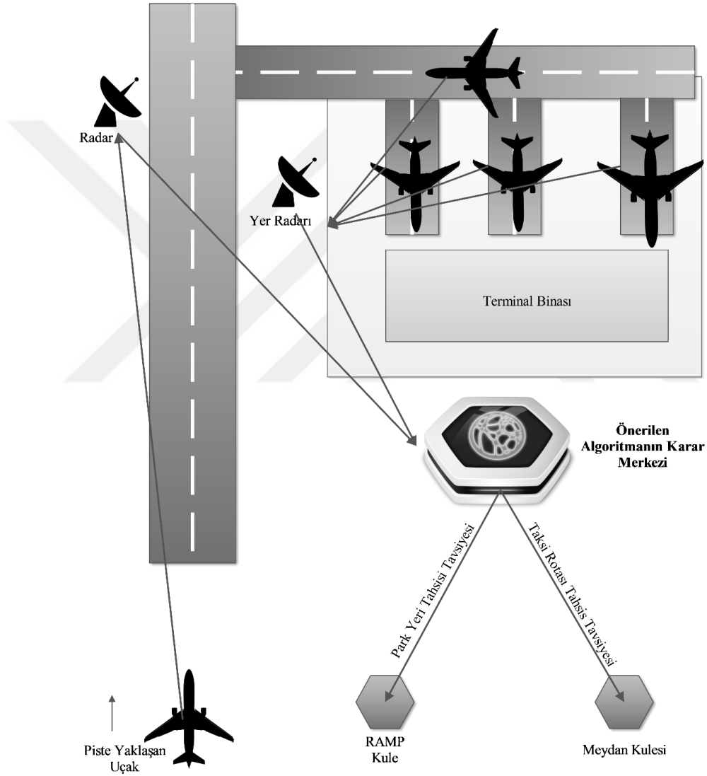
Şekil 6.3. Kombinasyonel park yeri ve taksi rotası tahsis algoritması veri hattı şeması
