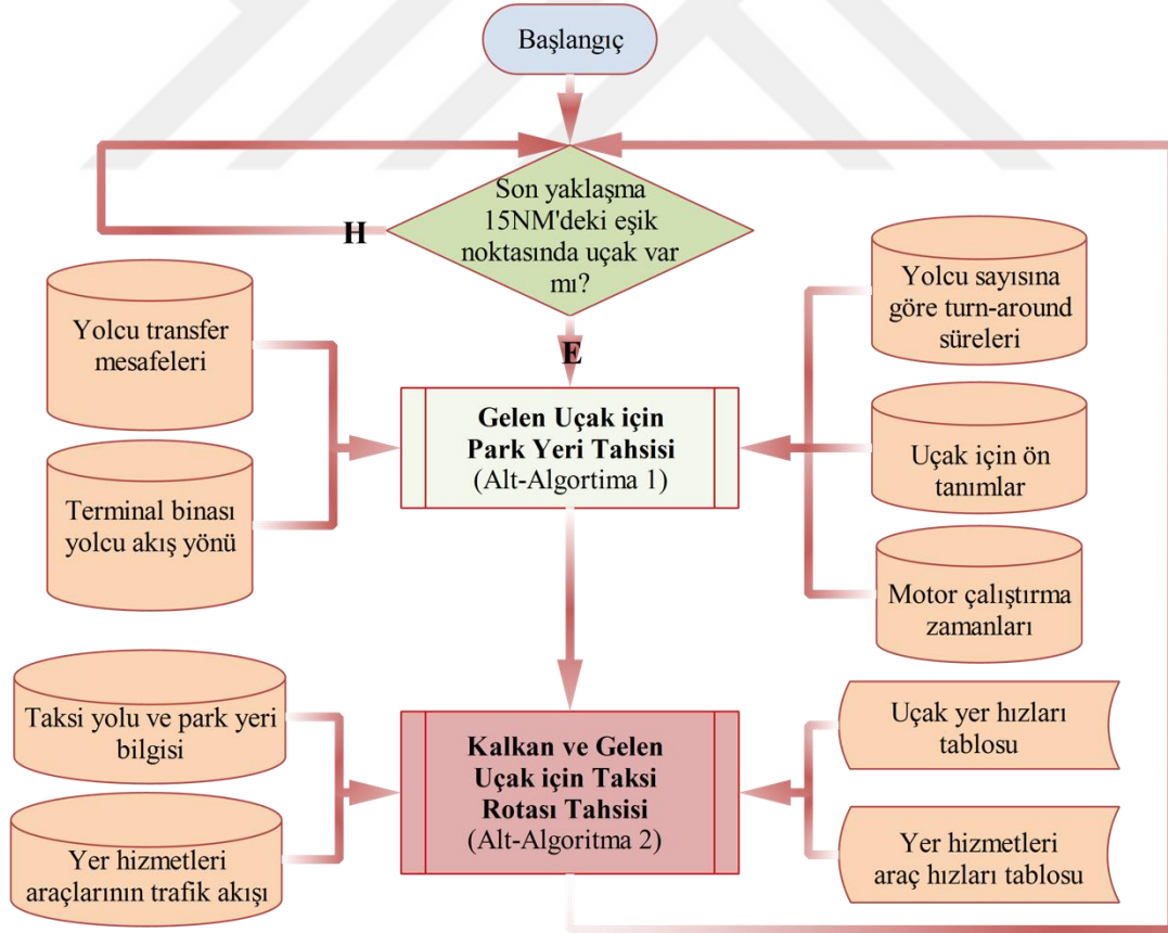
Şekil 3.1. Park yeri ve taksi rotası tahsisi genel algoritması
