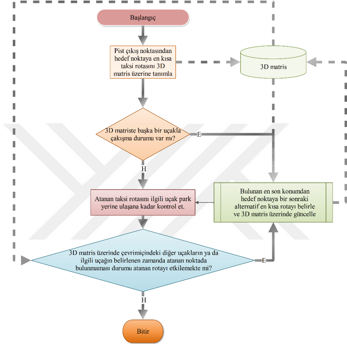
Şekil 3.4. "Alt-Algorithm 2": Taksi rotası tahsisi algoritması
