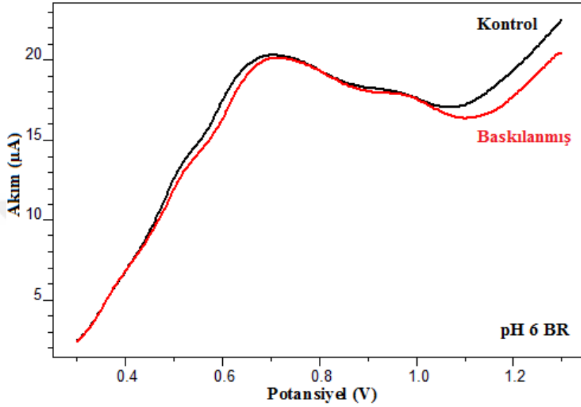
Şekil 4.6. 10^{-3} M monuron'un pH 6 BR tamponunda polimerizasyonu sonucu elde edilen elektrot (baskılanmış) ve monuron içermeyen sadece p-fenilendiamin içeren çözelti ile polimerize edilmiş elektrotun (kontrol) diferansiyel puls voltamogramları
