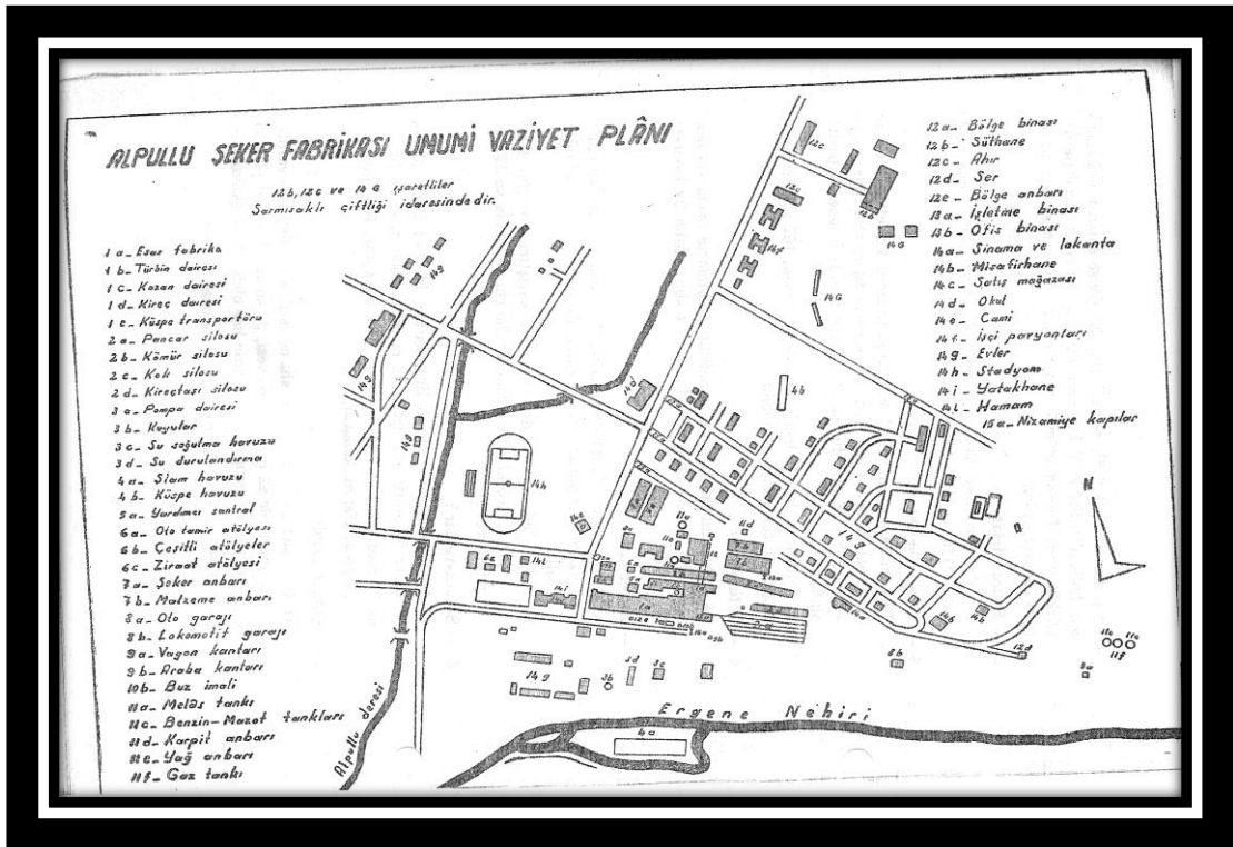
Plân 2: Alpullu Şeker Fabrikası Umumi Vaziyet Plânı
