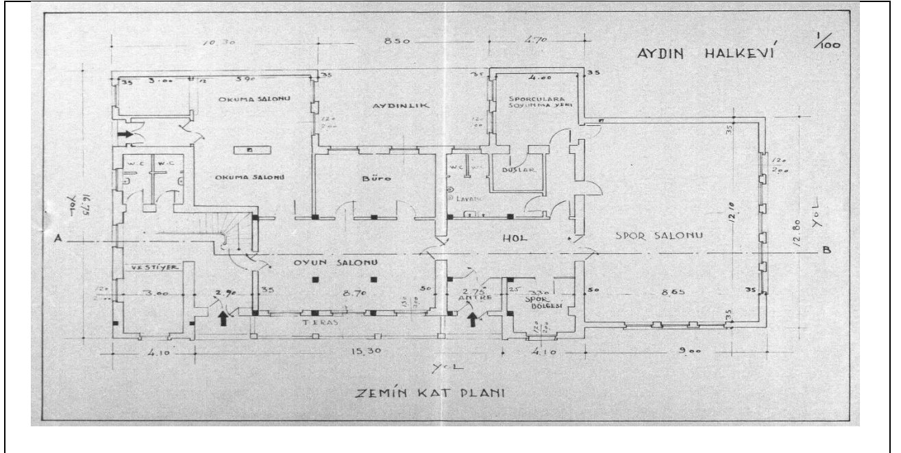
K-2: Aydın Halkevi Binasının Zemin Kat Krokisi
