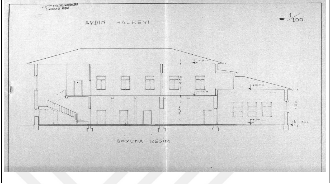
K-1: Aydın Halkevi Binasının Yandan Kroki Çizimi
