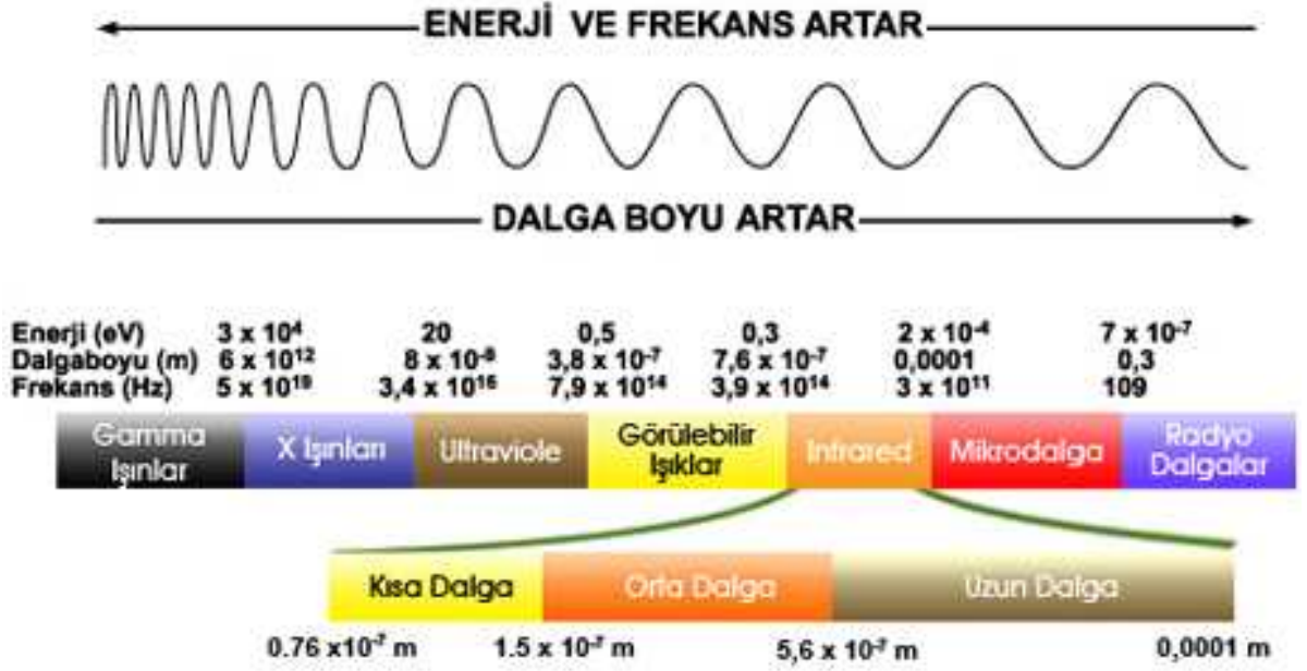
Şekil 7. Elektromanyetik Spektrum
