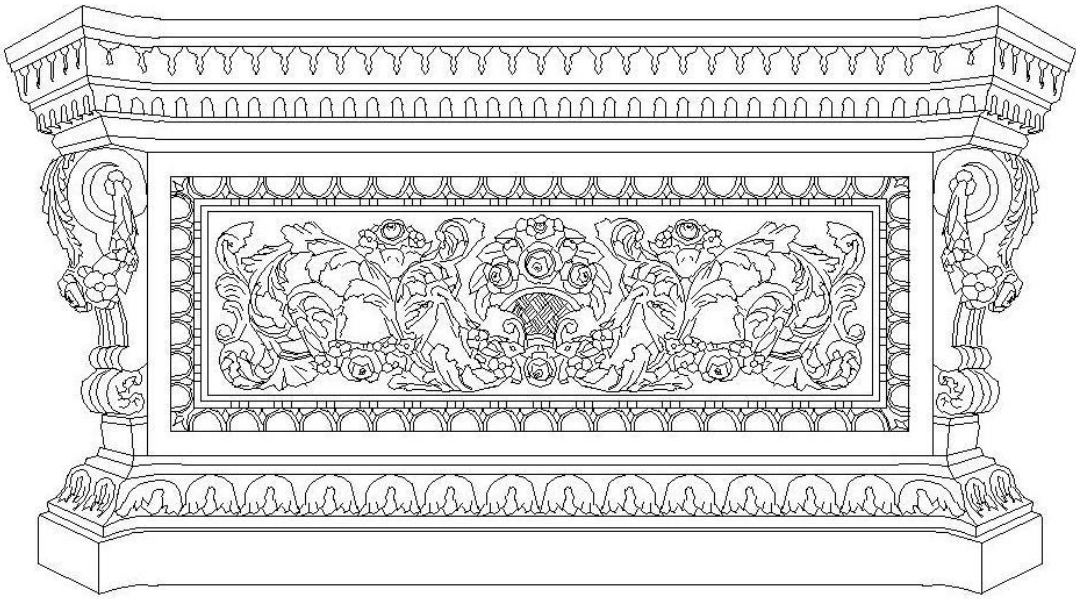
Çizim 59: 49 Nolu Mezarın Uzun Yüzeyi
