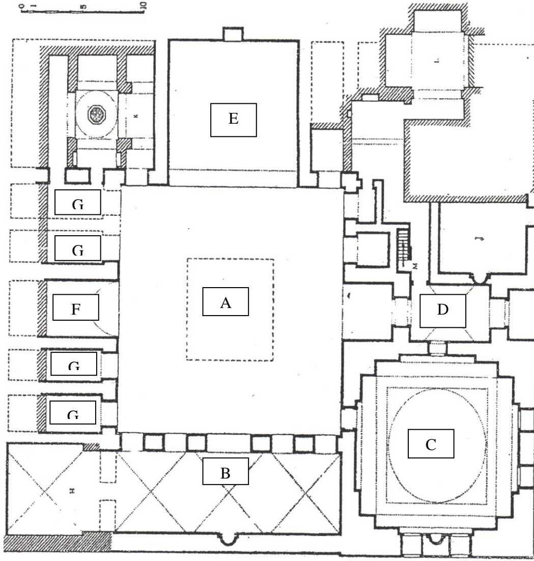
Resim 25 : Adilîye Medresesi planı
