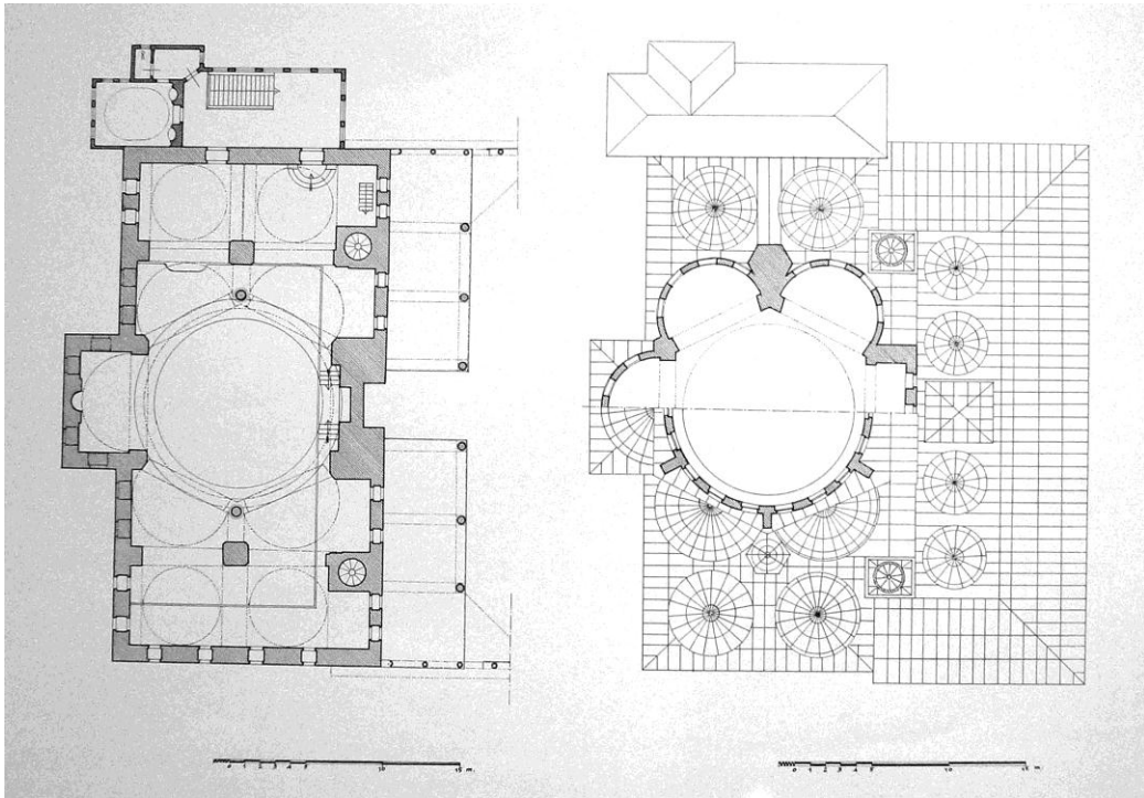
Plan 7: Vâlide-i Atik Camii Örtü Tabakaları. A. S. ÜLGEN, Mimar Sinan Yapıları , Ankara, 1989.
