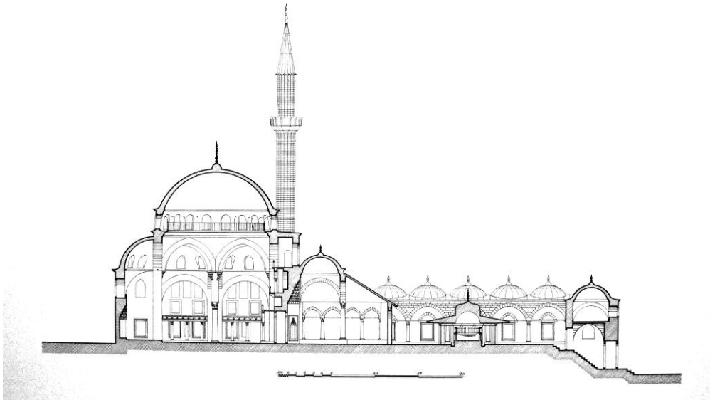
Plan 9: Vâlîde-i Atîk Camii Kesiti. A. S. ÜLGEN, Mimar Sinan Yapıları , Ankara, 1989.
