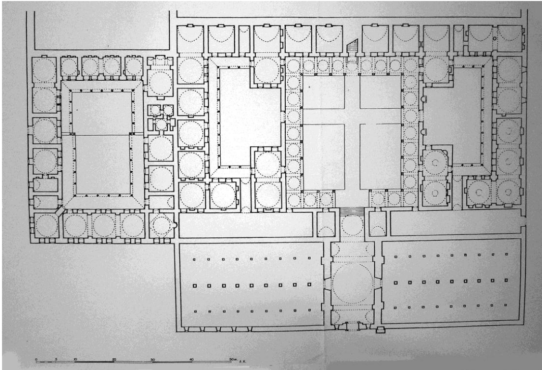
Plan 4: Vâlîde-i Atîk İmâreti Restitüsyonu. A. KURAN, Mimar Sinan , İstanbul, 1986.
