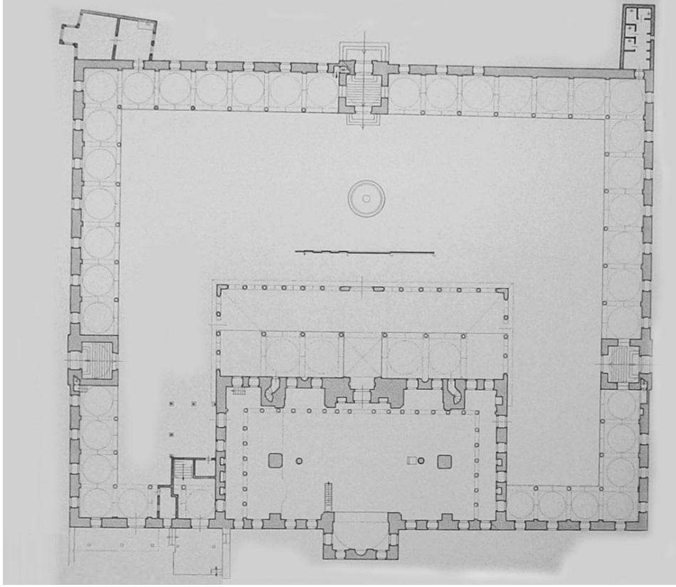
Plan 8: Vâlîde-i Atîk Camii. A. S. ÜLGEN, Mimar Sinan Yapıları , Ankara, 1989.
