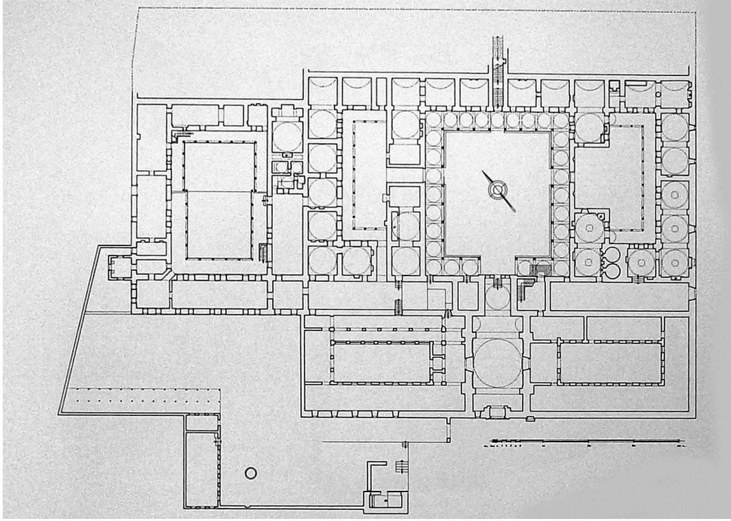
Plan 3: Vâlîde-i Atîk İmâreti. A. S. ÜLGEN, Mimar Sinan Yapıları , Ankara, 1989.
