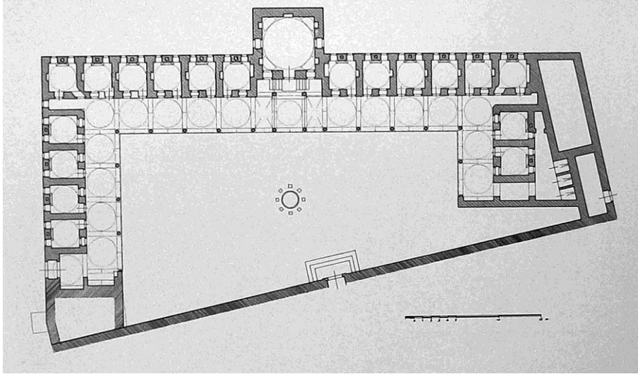
Plan 11: Vâlîde-i Atik Tekkesi. A. S. ÜLGEN, Mimar Sinan Yapıları , Ankara, 1989.
