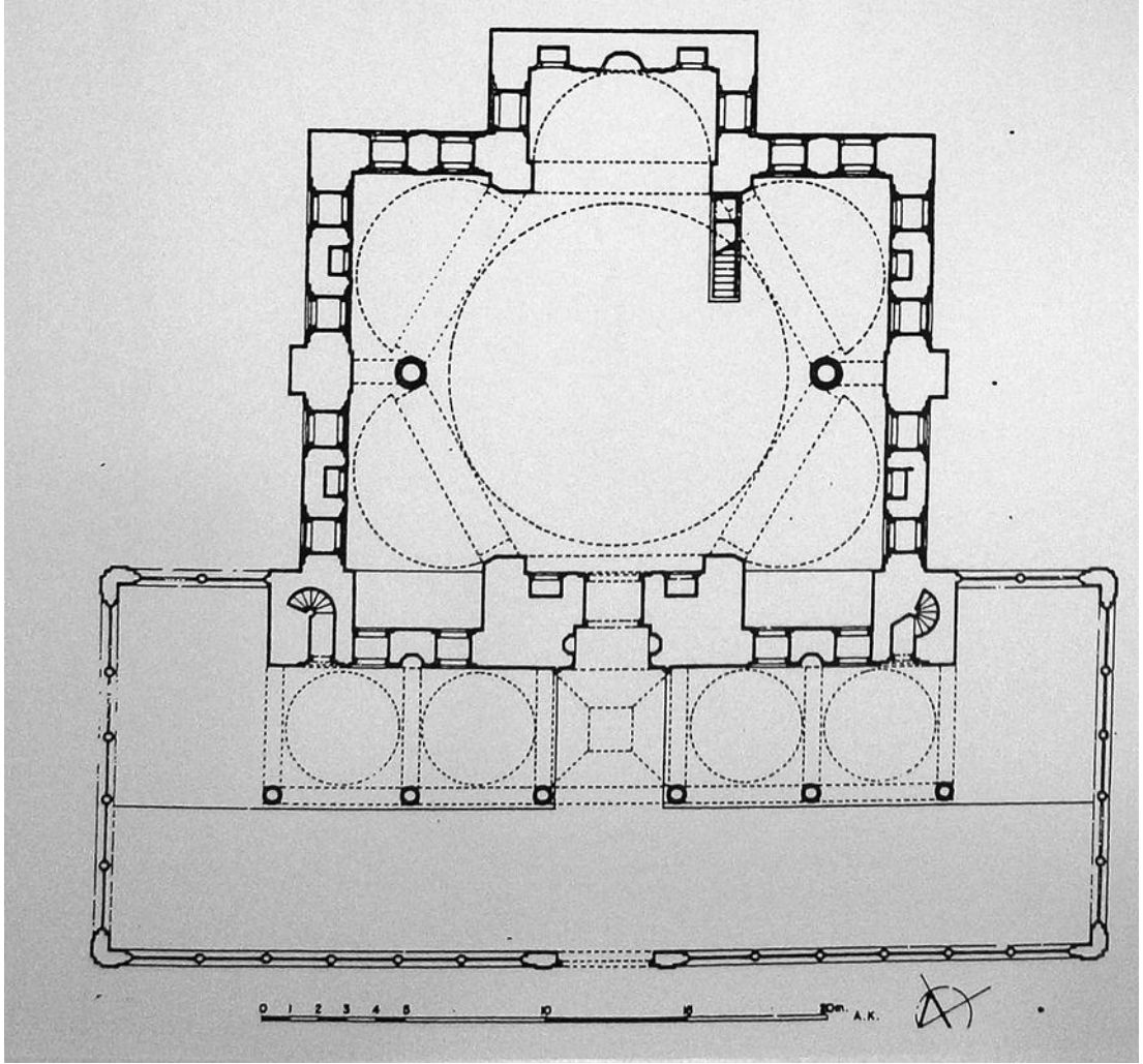
Plan 5: Vâlide-i Atik Camii'nin Yan Sahınlar Eklemlenmeden Önce Varsayılan Planı. A. KURAN, Mimar Sinan , İstanbul, 1986.
