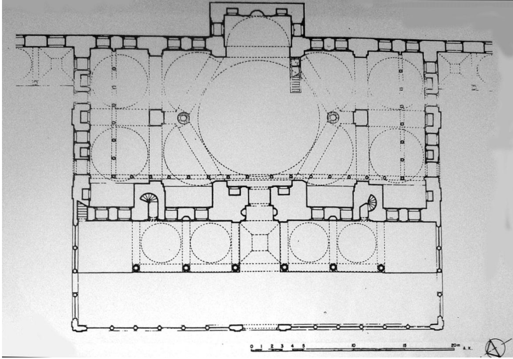
Plan 6: Vâlide-i Atik Camii. A. KURAN, Mimar Sinan , İstanbul, 1986.
