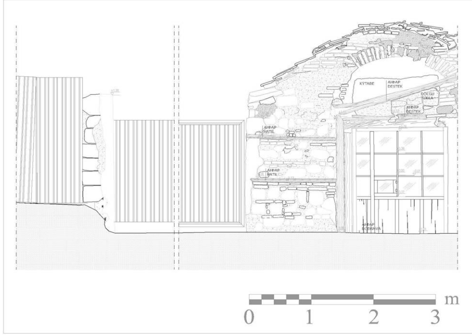
Şekil 2.11 Veli Dede Tekkesi, Giriş Kapısı arka görünüşü (2009, EM.Arşivi)
