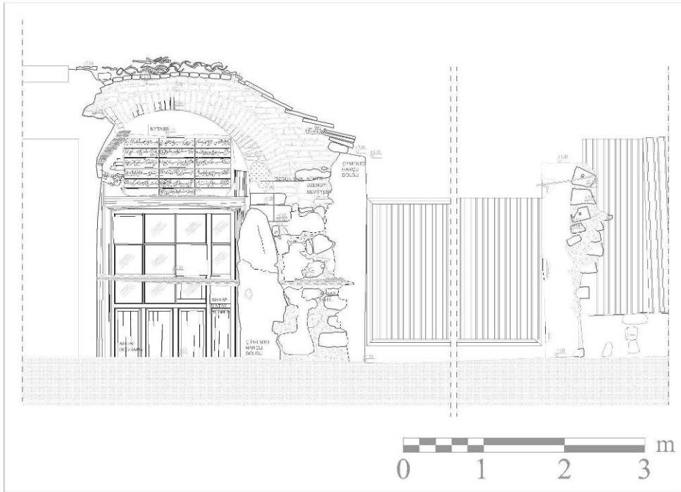
Şekil 2.10 Veli Dede Tekkesi, giriş kapısı ön görünüşü (2009, EM.Arşivi)
