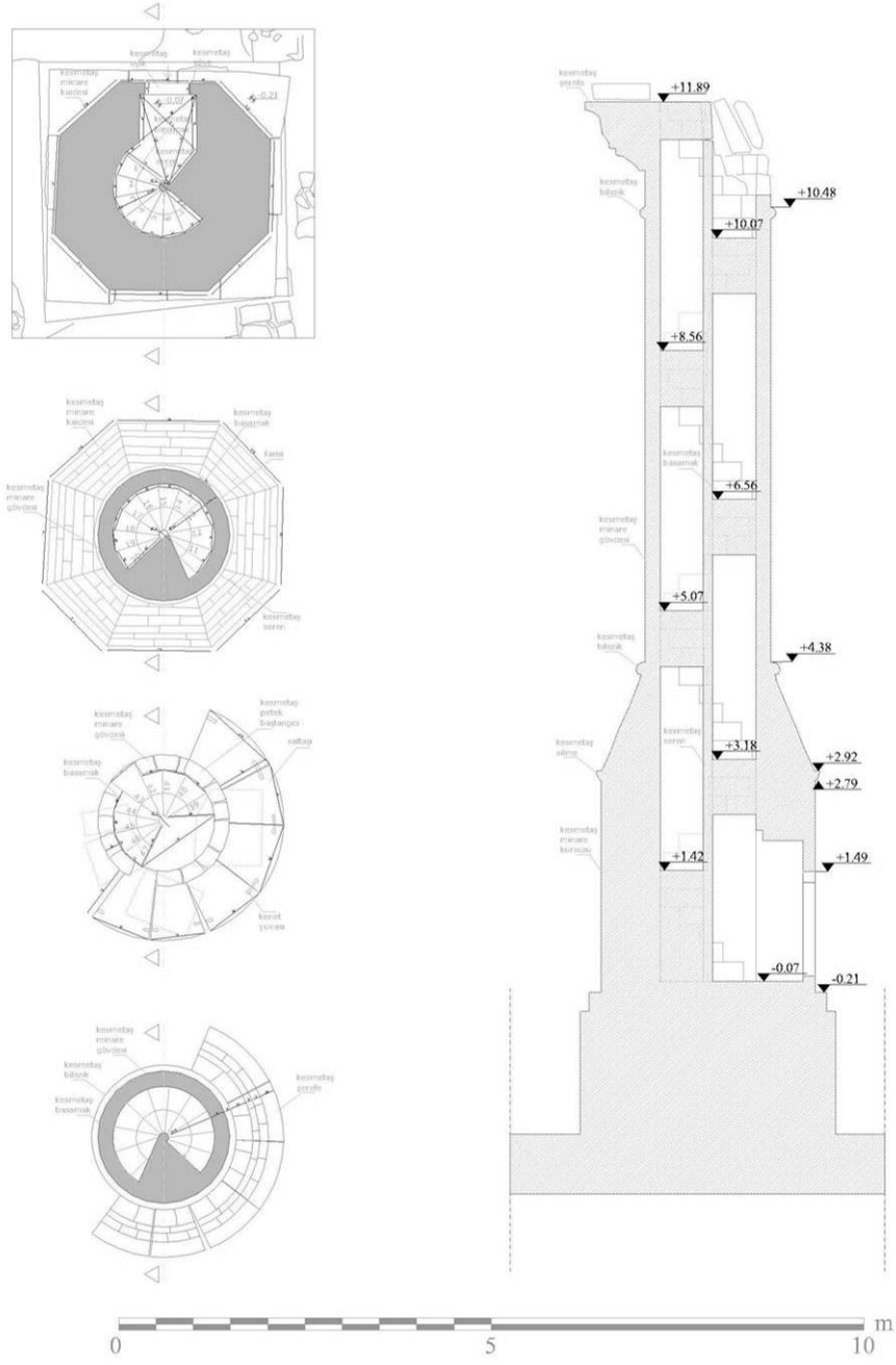
Şekil 2.13 Minare, plan ve kesit (2009, EM.Arşivi)
