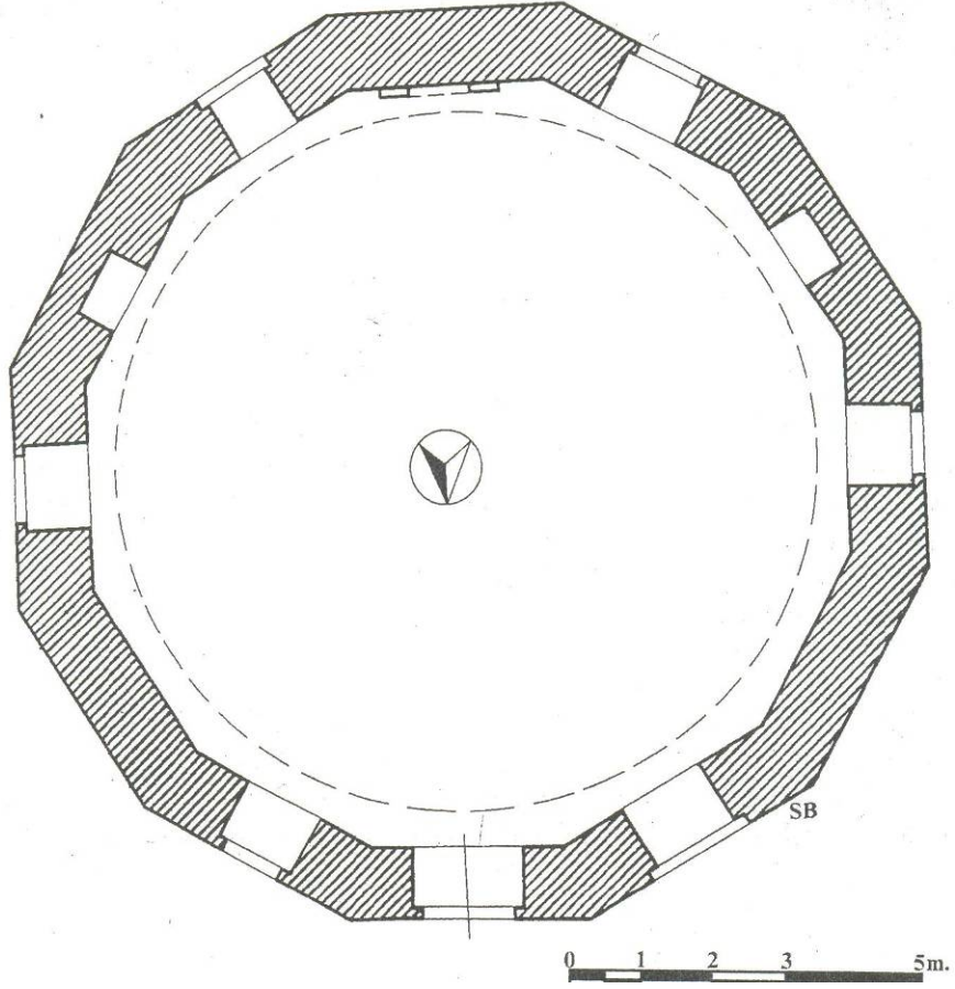
Şekil 2.2 Tütünsüz Baba Türbesi, plan (S.Bayrakal, 2002, s.124)
