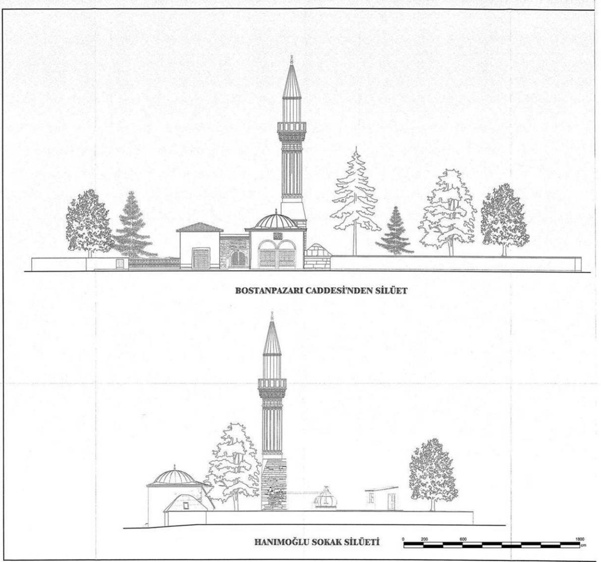
Şekil 2.4 Hasan Sezaî Tekkesi, görünüş (2007, EKVTVKBK.Arşivi)
