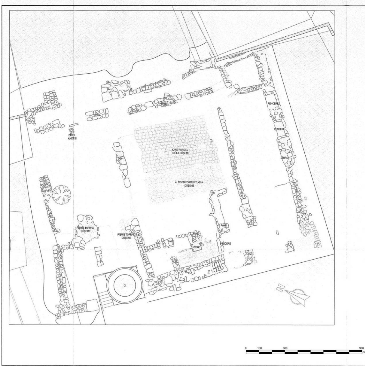
Şekil 2.8 Hasan Sezaî Tekkesi, Kazı Rölövesi (2007, EKVTVKBK.Arşivi)
