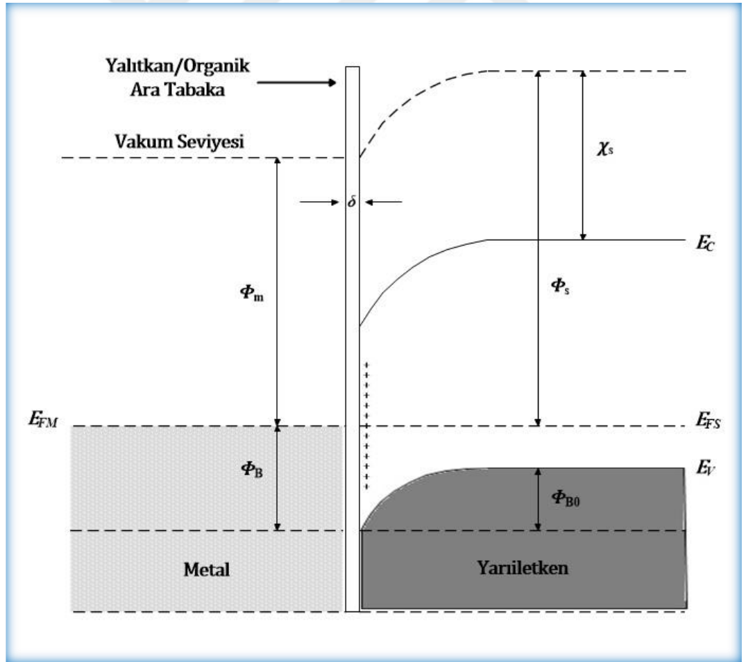
Şekil 2.3. P-tipi yarıiletkene sahip bir MIS/MPS yapısındaki enerji bant diyagramı.
