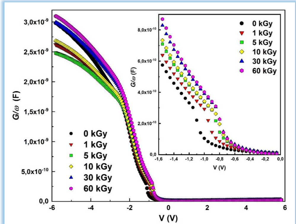
Şekil 6.2. MPS tipi SD'nin ışınlamadan önce ve sonraki G/\omega - V karakterisitikleri.
