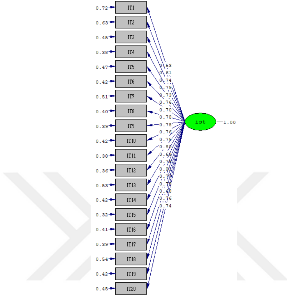
Şekil 16. İş Tatmini Ölçeği için DFA PATH Diyagramı
