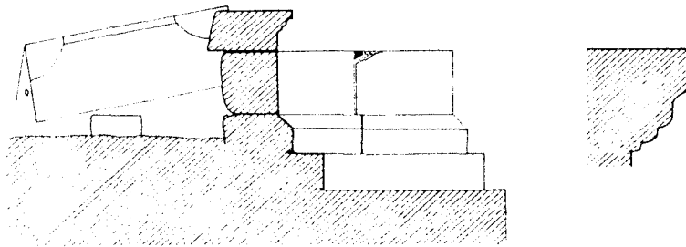
c- Patara Akdam sunakgömüt, AA' kesiti.
