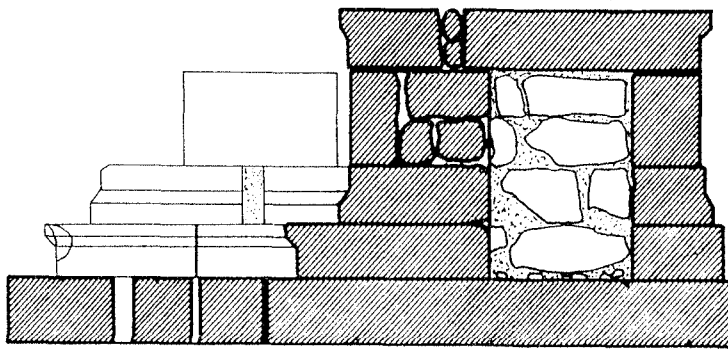
c- Patara Ambaryanı sunakgömüt, BB' kesiti.
