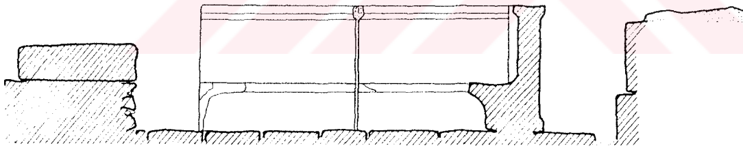
b- Patara M73 gömütü, AA' kesiti.
