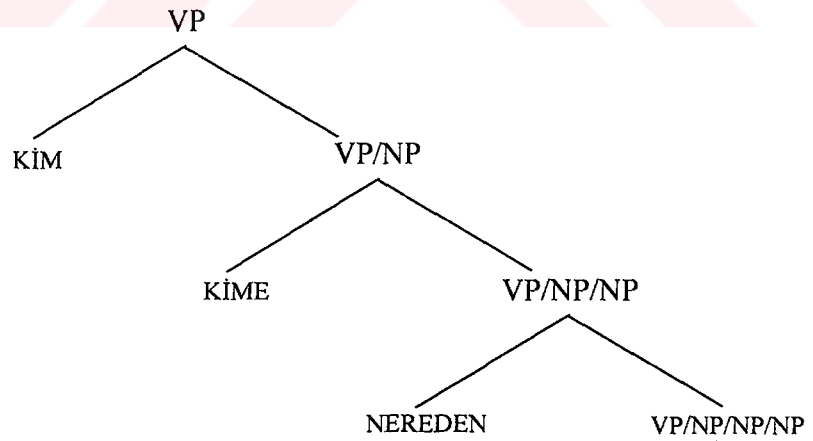
Şekil 6.3 Üç parametrelî fiiller için programımızın kullandığı sözdizim ağacı
