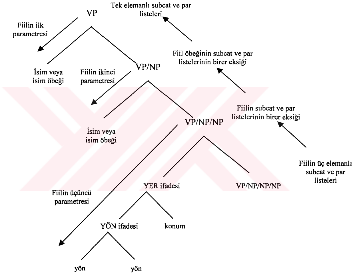
Şekil 7.1 Üç parametrelili fiiller için fiilin parametrelerinin belirlenmesi ve eşleşme işlemi
