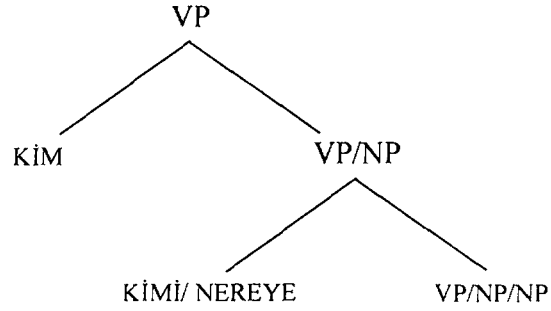
Şekil 6.2 İki parametrelî fiiller için programımızın kullandığı sözdizim ağacı
