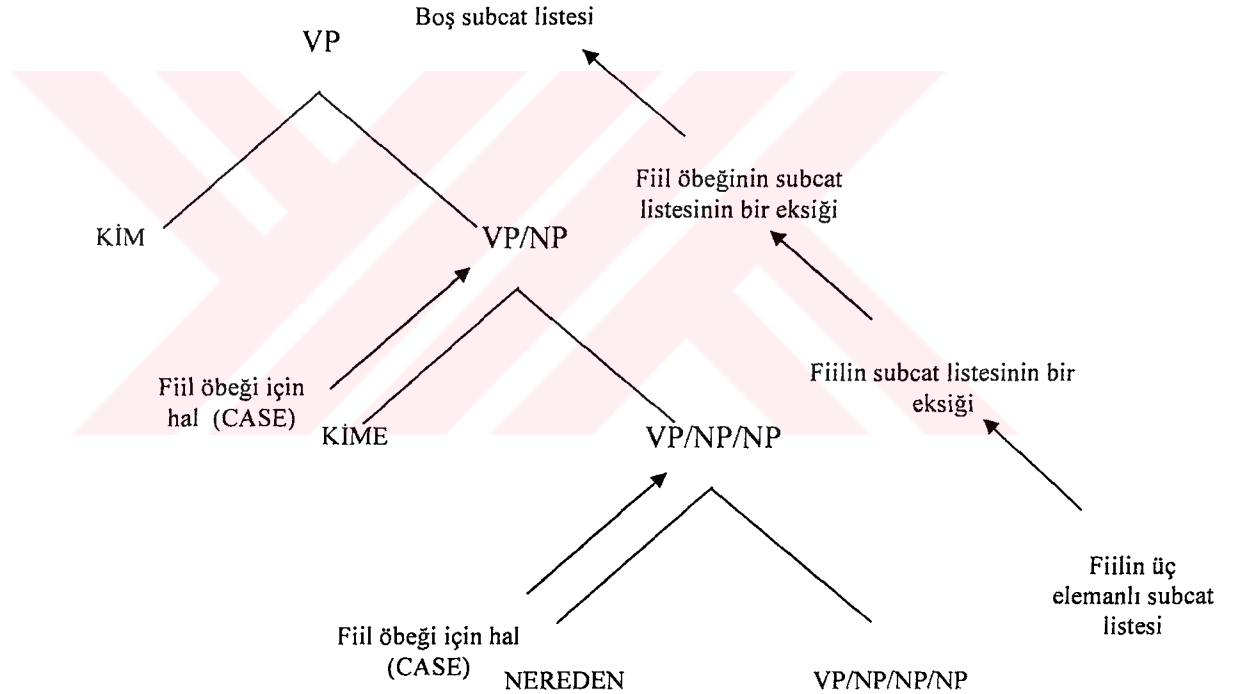
Şekil 6.4 Üç parametrelili fiiller için özelliklerin alındığı yerler
