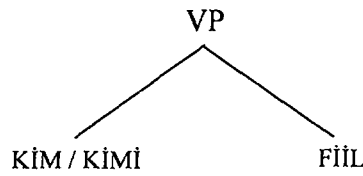
Şekil 6.1 Tek parametrelili fiiller için programımızın kullandığı sözdizim ağacı
