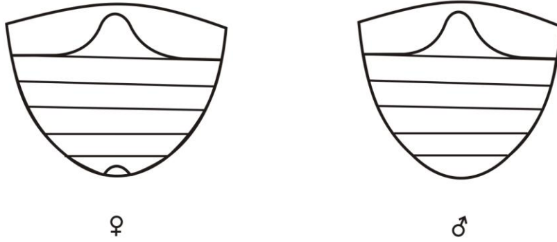
Őekil 3. Propylea quatuordecimpunctata 'da cinsiyet tayini. Abdominal segmentler eřeyler arasındaki farkı gstermektedir. (Majerus, 1989) dan.
