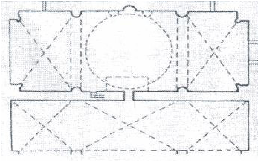
Plan 4: Eski Ömeriye Camii ( Cihat Kütükçüođlu )
