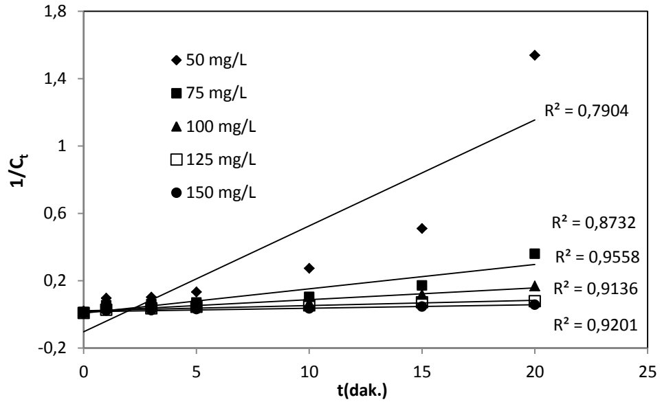
Şekil 4.22. Farklı DB71 konsantrasyonlarının Fenton oksidasyonu ile renk giderimindeki ikinci derece kinetik modeli *( Fe^{2+}=3.0 \text{ mgL}^{-1} , H_2O_2=125 \text{ mgL}^{-1} , pH=3.0 , T=20^0C )
