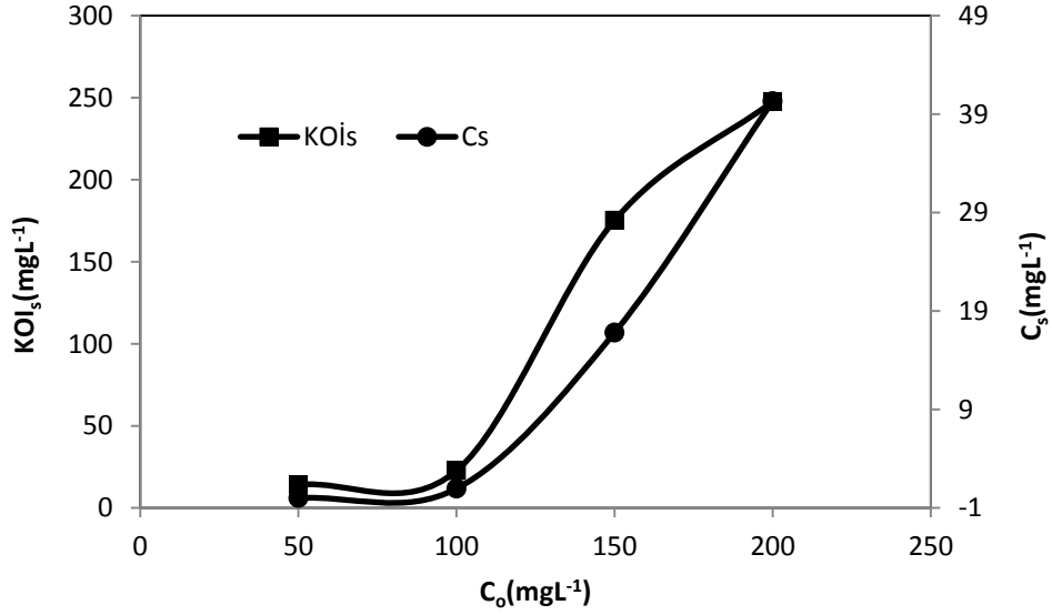
Şekil 4.13. BB9'un Fenton-benzeri oksidasyonunda boya konsantrasyonunun renk ve KOİ giderimine etkisi ( Fe^0=0,1 \text{ gL}^{-1} , H_2O_2=75 \text{ mgL}^{-1} , pH=3,0 , T=20^0C , t=20 \text{ dak.} )
