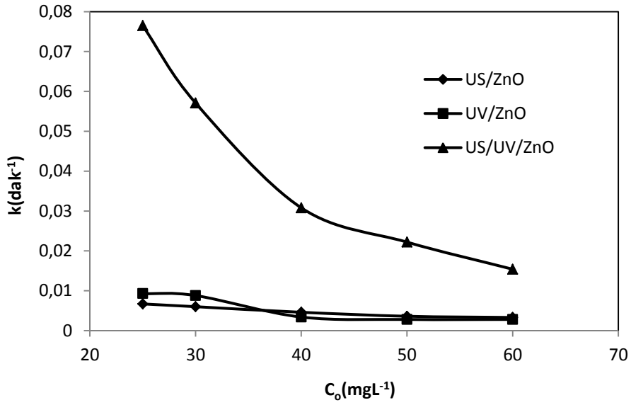
Şekil 4.78. BB9'un farklı şartlardaki renk giderimine başlangıç konsantrasyonunun etkisinin birinci derece hız sabiti ile değerlendirilmesi *(ZnO=400 mgL -1 , pH=5.5, T=20 0 C, t=60 dak.)
