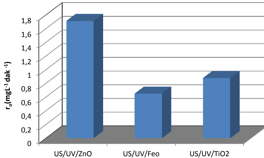
Şekil 4.82. BB9’un sonofotokatalitik oksidasyon ile renk giderimine farklı katalizörlerin etkisi
