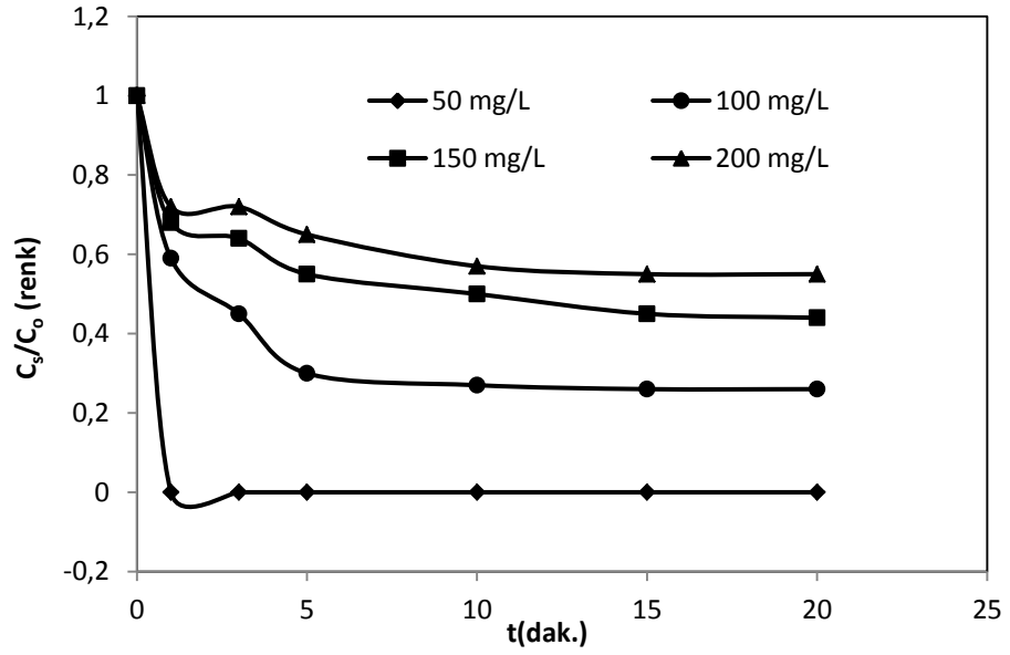
Şekil 4.45. DB71'in ultrasonik parçalanmasına boyar madde konsantrasyonunun etkisi *(pH=2.5, TiO_2=1gL^{-1} , amplitude=%90, T=20^0C , t=20 dak.)
