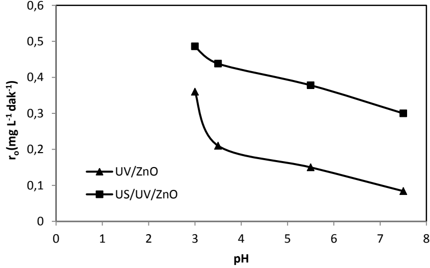
Şekil 4.73. DB71'in farklı şartlardaki renk giderimine pH'nın etkisi *(C o =60 mgL -1 , ZnO=400 mgL -1 , T=20°C, t=60 dak.)
