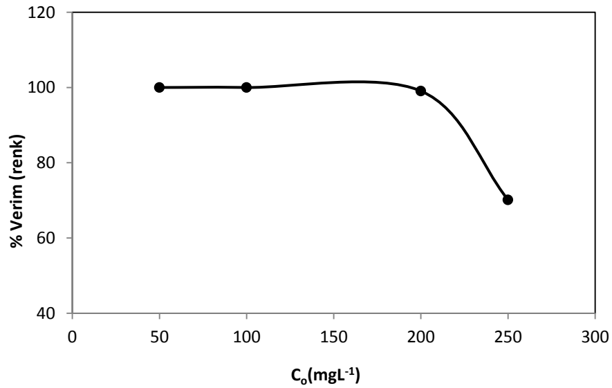
Şekil 4.42. DB71'in ultrasonik parçalanmasına başlangıç boyar madde konsantrasyonlarının etkisi *(pH=2.5, \text{ZnO}=2 \text{ gL}^{-1} , amplitude=%90, T=20^\circ\text{C} , t=20 \text{ dak.} )
