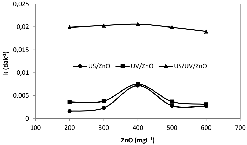
Şekil 4.69. DB71'in farklı şartlardaki renk giderimine ZnO'nun etkisi *(C 0 =30 mgL -1 , pH=5.5, T=20 0 C, t=60 dak.)
