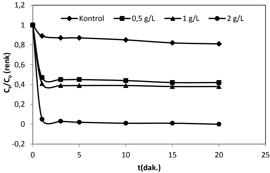
Şekil 4.40. DB71'in ultrasonik parçalanmasına ZnO'nun etkisi
