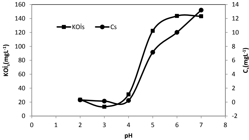
Şekil 4.5. BB9'un Fenton oksidasyonunda pH'nın renk ve KOİ giderimine etkisi *( C_0=100 \text{ mgL}^{-1} , KOİ_0=147,8 \text{ mgL}^{-1} , Fe^{2+}=3 \text{ mgL}^{-1} , H_2O_2=100 \text{ mgL}^{-1} , T=20^{\circ}C , t=20 \text{ dak.} )
