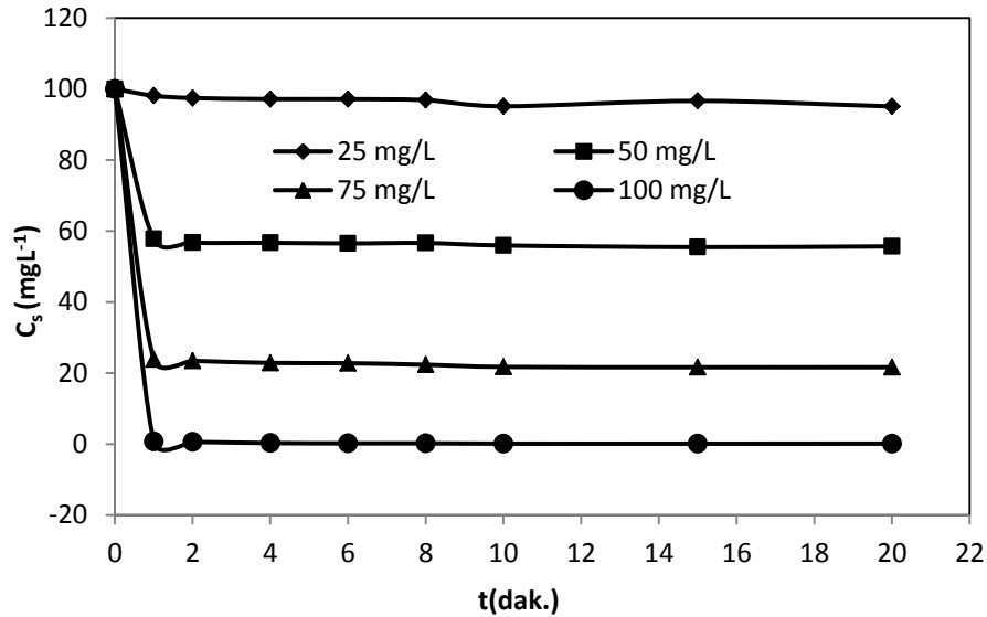
Şekil 4.3. BB9'un Fenton oksidasyonunda H_2O_2 miktarının renk giderimine etkisi *( C_0=100\text{ mgL}^{-1} , Fe^{2+}=3\text{ mgL}^{-1} , pH=3.0 , T=20^\circ C , t=20\text{ dak.} )
