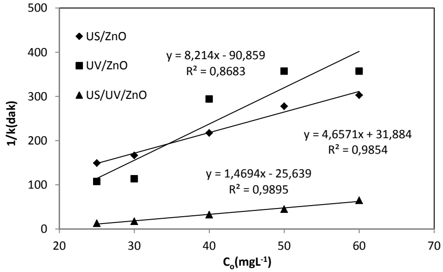
Şekil 4.81. BB9 boyar maddesinin Langmuir-Hinshelwood Kinetiği *( ZnO=400 \text{ mgL}^{-1} , pH=5.5 , T=20^{\circ}\text{C} , t=60 \text{ dak.} )
