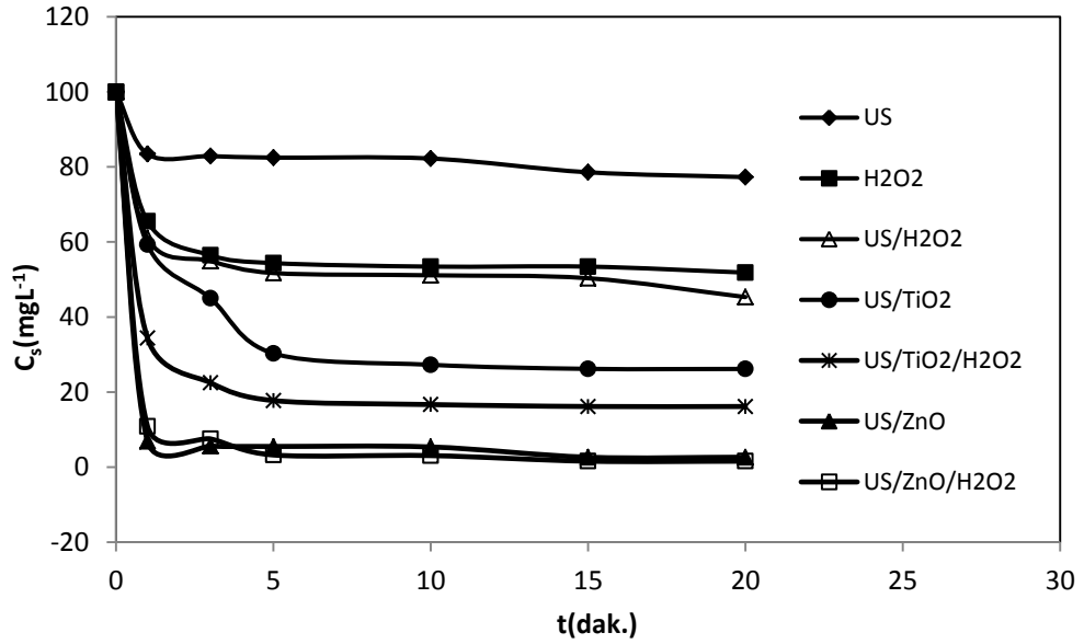
Şekil 4.53. DB71'in heterojen US oksidasyonu sonucu kalan boyar madde konsantrasyonu
