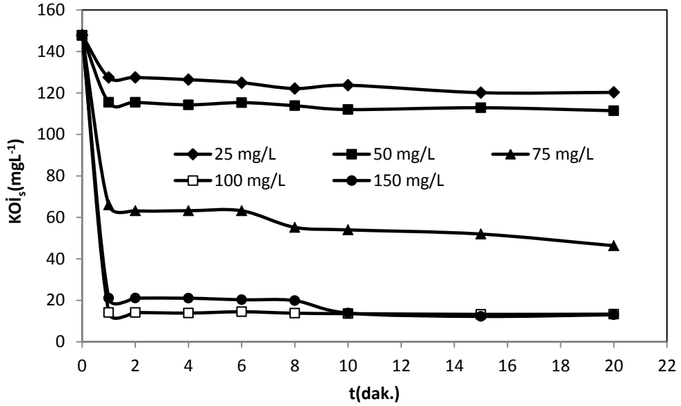
Şekil 4.4. BB9'un Fenton oksidasyonunda H_2O_2 miktarının KOİ giderimine etkisi *( C_0=100 \text{ mgL}^{-1} , KOİ_0=147,8 \text{ mgL}^{-1} , Fe^{2+}=3 \text{ mgL}^{-1} , pH=3,0 , T=20^0C , t=20 \text{ dak.} )
