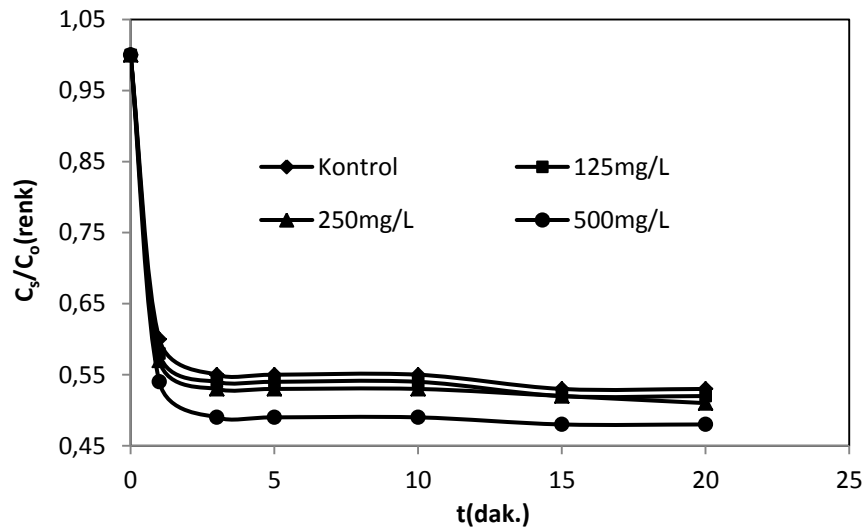
Şekil 4.50. DB71'in ultrasonik parçalanmasına butanol'un etkisi *( C_0=50 \text{mgL}^{-1} , pH=2.0, amplitude=%90, T=20^\circ\text{C} , t=20 dak.)
