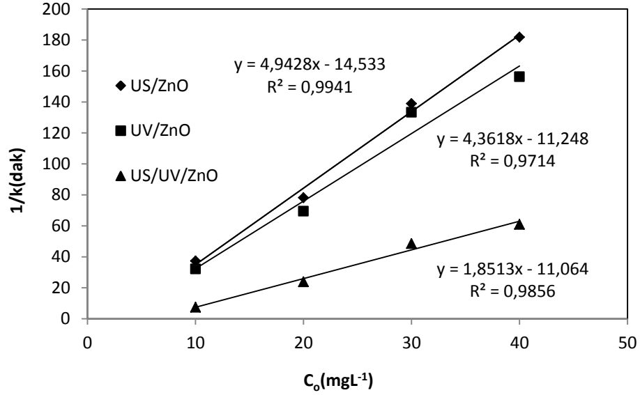
Şekil 4.74. DB71 boyar maddesinin Langmuir-Hinshelwood Kinetiği *(ZnO=400 mgL -1 , pH=5.5, T=20°C, t=60 dak.)
