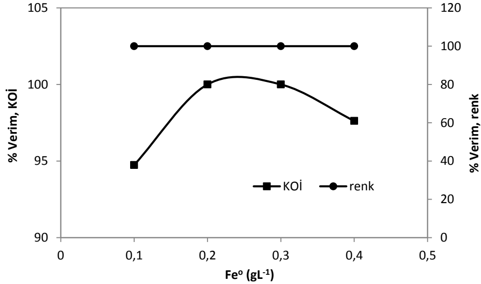
Şekil 4.23. DB71'in Fenton-benzeri oksidasyonunda Fe^0 miktarının renk ve KOİ giderme verimine etkisi
