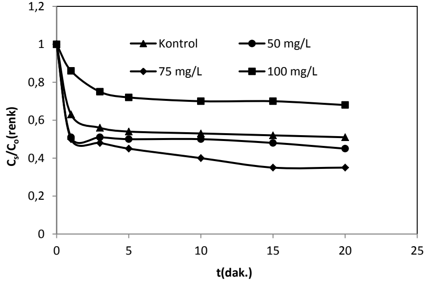
Şekil 4.37. DB71'in ultrasonik parçalanmasına H 2 O 2 'nin etkisi * (C 0 =50 mgL -1 , pH=2.5, amplitude=%90, T=20 0 C, t=20 dak.)
