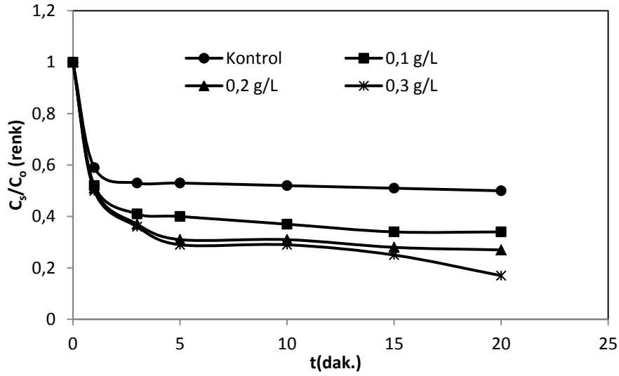
Şekil 4.33. DB71'in ultrasonik parçalanmasına Fe 0 'in etkisi *(C 0 =50 mgL -1 , pH=2,5, amplitude=%60, T=20 0 C, t=20dak.)
