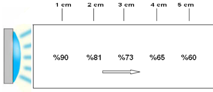
Şekil 2.2. UV ışın yoğunluğunun su içerisindeki difüzyonu
