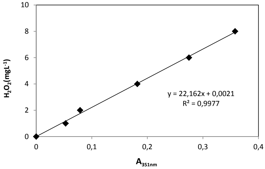
Şekil 3.13. H 2 O 2 kalibrasyon eğrisi.
