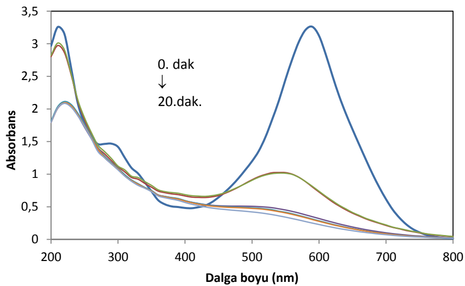
Şekil 4.15. DB71'in Fenton oksidasyonu ile renk gideriminin absorbans azalması *( C_0=60 \text{ mgL}^{-1} , \text{H}_2\text{O}_2=50 \text{ mgL}^{-1} , \text{Fe}^{2+}=1,5 \text{ mgL}^{-1} , \text{pH}=3.0 , t=20 dak.)
