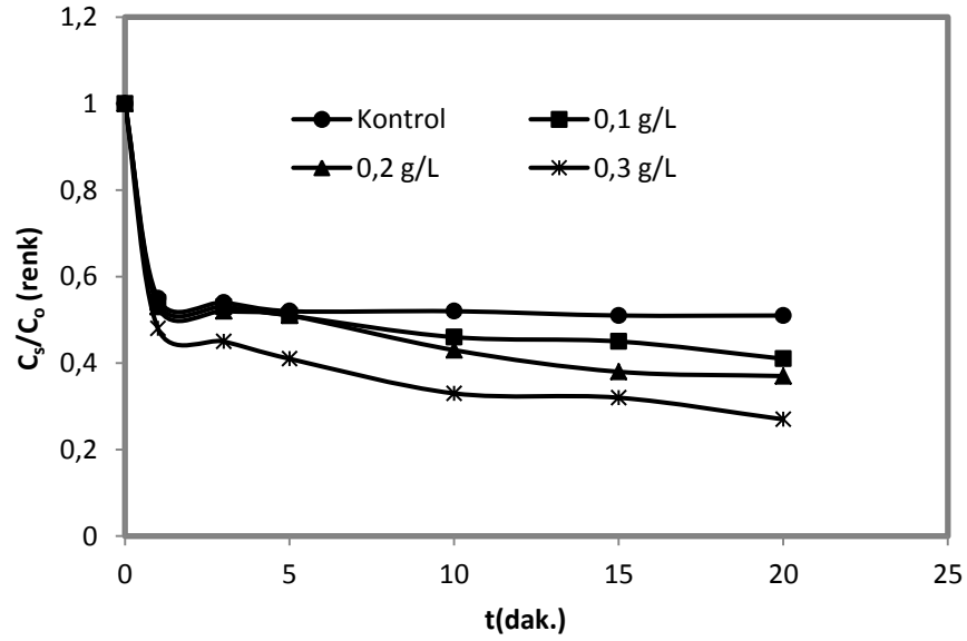
Şekil 4.32. DB71'in ultrasonik parçalanmasına Fe 0 'in etkisi *(C 0 =50 mgL -1 , pH=2,5, amplitude=%30, T=20 0 C, t=20dak.)
