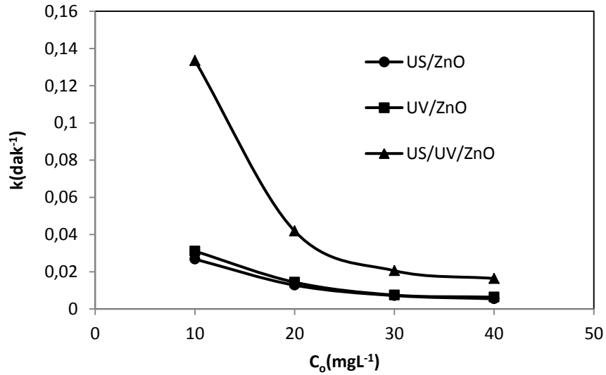
Şekil 4.71. DB71'in farklı şartlardaki renk giderimine başlangıç konsantrasyonun etkisinin birinci derece hız sabiti ile değerlendirilmesi
