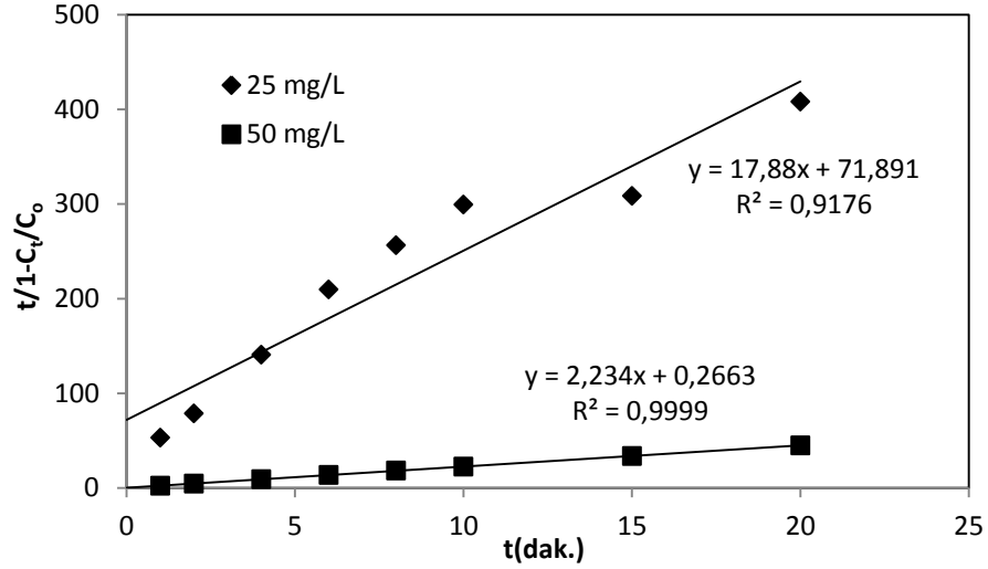
Şekil 4.8. Farklı H 2 O 2 konsantrasyonları ile BB9'un Fenton oksidasyonu ile renk giderimindeki BMG kinetik modeli *(C 0 =100 mgL -1 , Fe 2+ =3 mgL -1 , pH=3.0, T=20 0 C)
