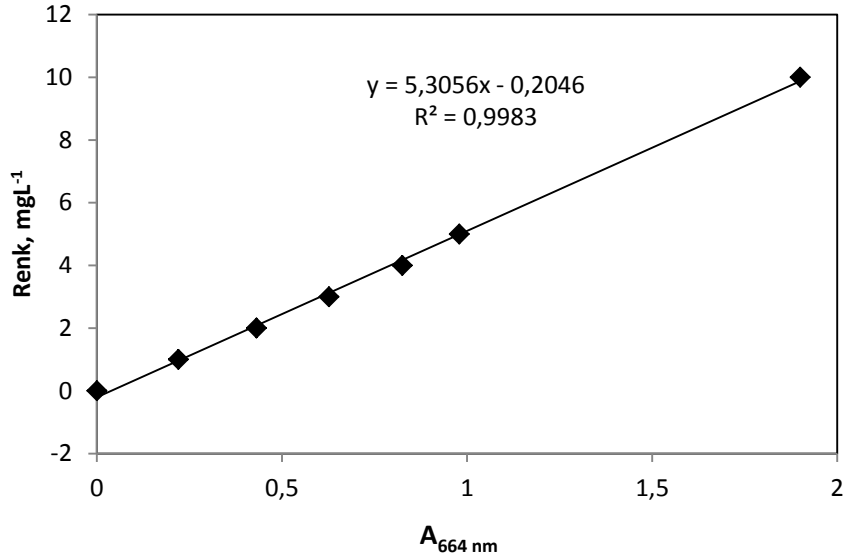
Şekil 3.9. BB9 boyar maddesi için kalibrasyon eğrisi.
