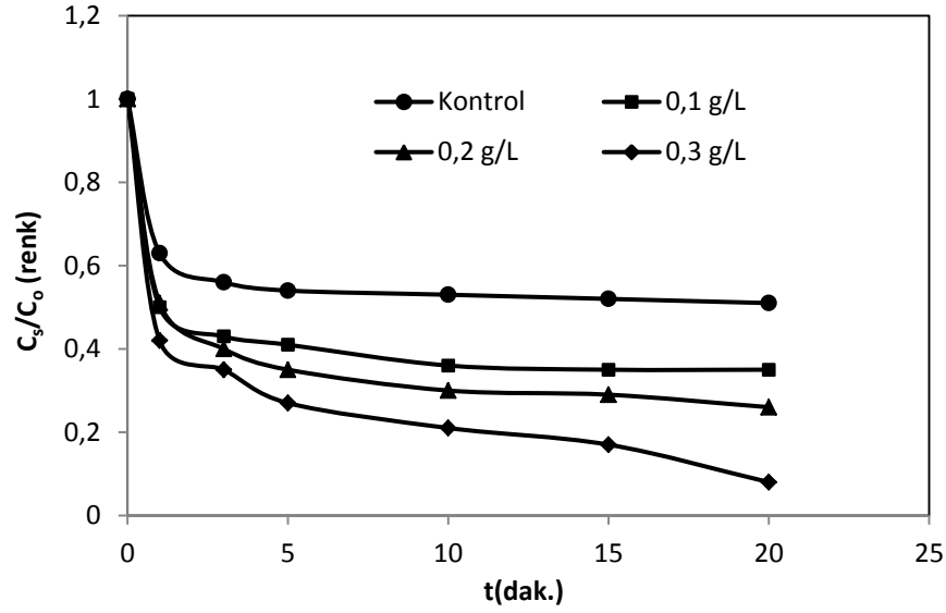
Şekil 4.34. DB71'in ultrasonik parçalanmasına Fe 0 'ın etkisi *(C 0 =50 mgL -1 , pH=2.5, amplitude=%90, T=20°C, t=20 dak.)
