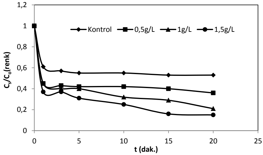
Şekil 4.46. DB71'in ultrasonik parçalanmasına Aktif karbonun etkisi *( C_0=100 \text{ mgL}^{-1} , pH=2.0, amplitude=%90, T=20^\circ\text{C} , t=20 dak.)
