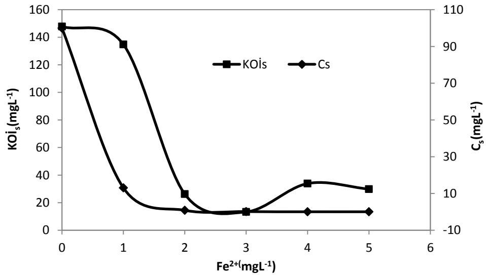
Şekil 4.2. BB9’un Fenton oksidasyonunda \text{Fe}^{2+} miktarının renk ve KOİ giderimine etkisi
