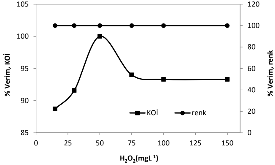
Şekil 4.24. DB71'in Fenton-benzeri oksidasyonunda H 2 O 2 miktarının renk ve KOİ giderme verimine etkisi
