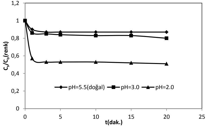
Şekil 4.49. DB71'in ultrasonik parçalanmasına pH'nın etkisi *( C_0=50\text{mgL}^{-1} , butanol = 250\text{mgL}^{-1} , amplitude=%90, T=20^\circ\text{C} , t=20 dak.)
