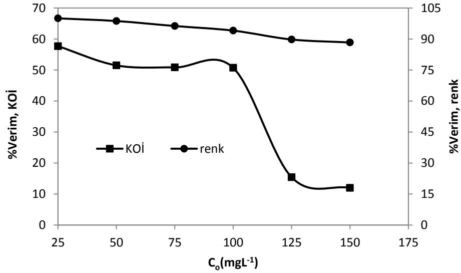
Şekil 4.19. DB71'in Fenton oksidasyonunda başlangıç boya konsantrasyonunun renk ve KOİ giderme verimine etkisi
