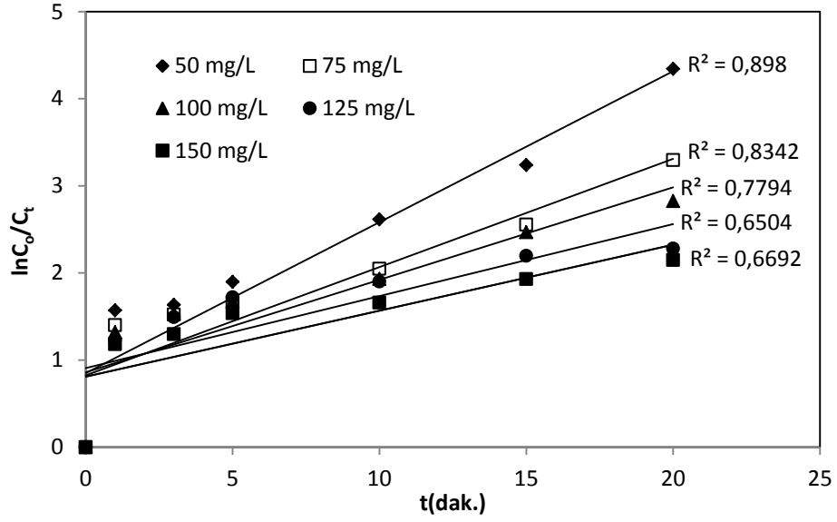
Şekil 4.21. Farklı DB71 konsantrasyonlarının Fenton oksidasyonu ile renk giderimindeki birinci derece kinetik modeli *( Fe^{2+}=3.0 \text{ mgL}^{-1} , H_2O_2=125 \text{ mgL}^{-1} , pH=3.0 , T=20^0C )
