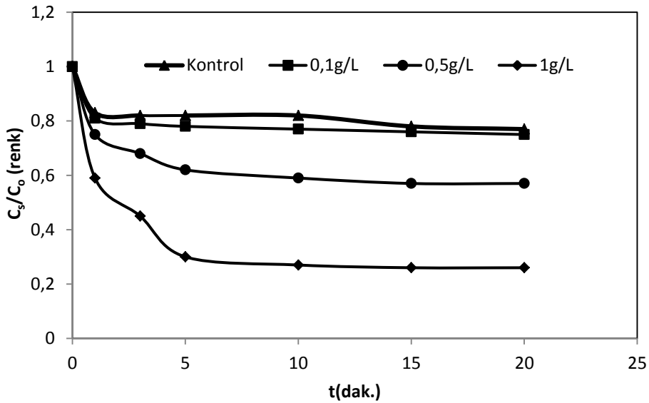
Şekil 4.43. DB71'in ultrasonik parçalanmasına TiO 2 'nin etkisi
