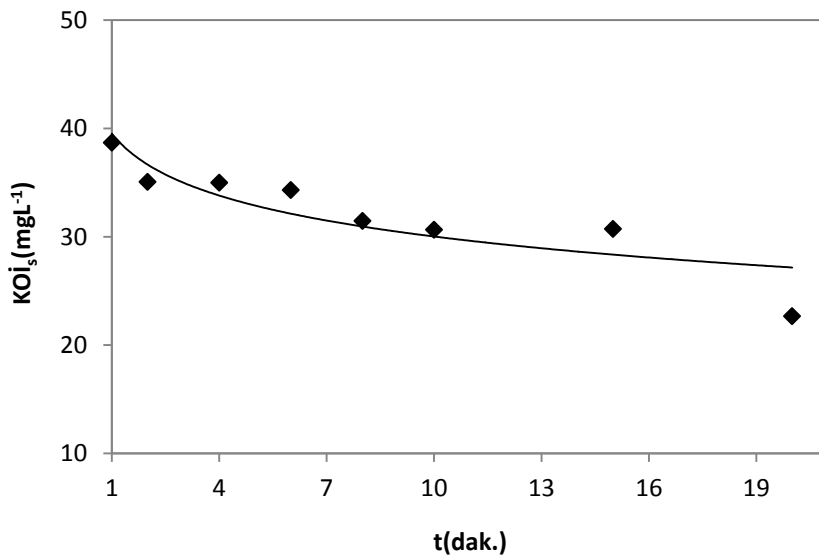
Şekil 4.14. BB9'un Fenton-benzeri oksidasyonunda farklı zamanlarda KOİ giderimi ( C_0=100 \text{ mgL}^{-1} , KOİ_0=147,8 \text{ mgL}^{-1} , Fe^0=0,1 \text{ gL}^{-1} , H_2O_2=75 \text{ mgL}^{-1} , pH=3,0 , T=20^0C , t=20 \text{ dak.} )
