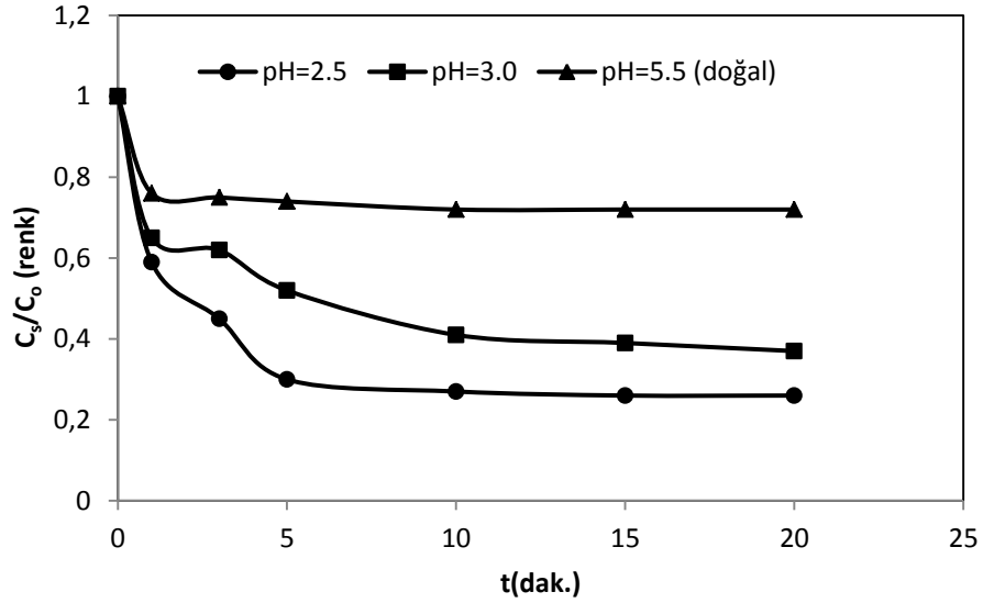
Şekil 4.44. DB71'in ultrasonik parçalanmasına pH değerinin etkisi
