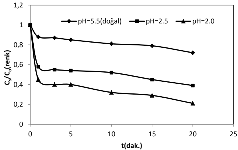
Şekil 4.47. DB71'in ultrasonik parçalanmasına pH'nın etkisi *( C_0=100 \text{ mgL}^{-1} , aktif karbon=1 \text{gL}^{-1} , amplitude=%90, T=20^\circ\text{C} , t=20 dak.)
