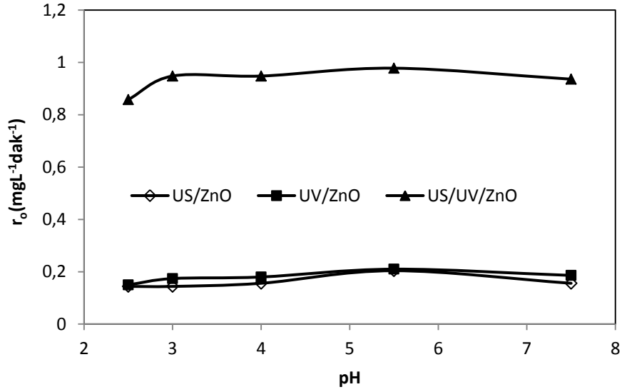
Şekil 4.80. BB9'un farklı şartlardaki renk giderimine pH'nın etkisi *( C_o=60 \text{ mgL}^{-1} , ZnO=400 \text{ mgL}^{-1} , T=20^{\circ}\text{C} , t=60 \text{ dak.} )
