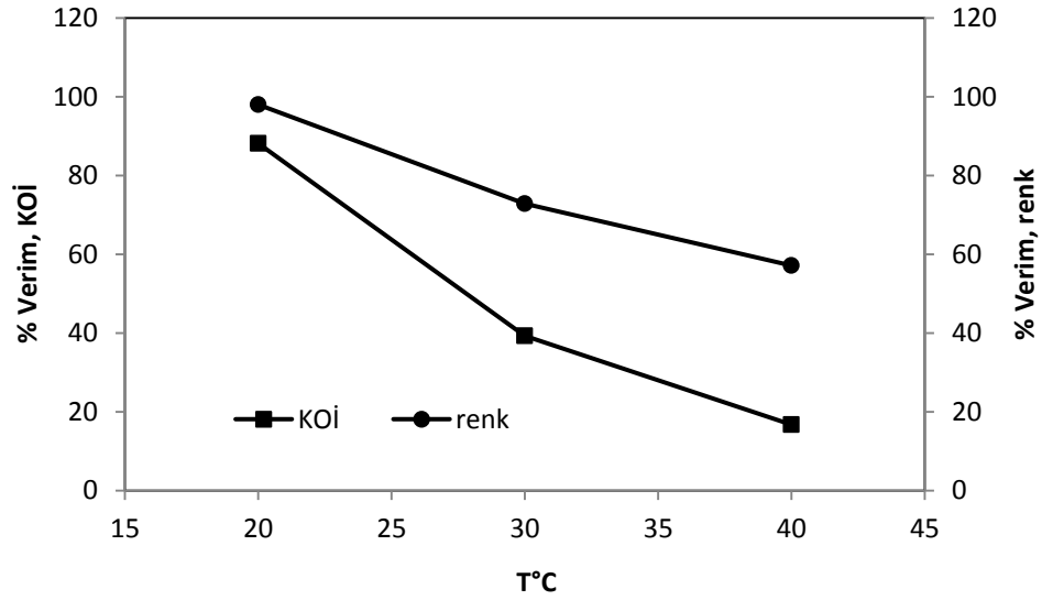
Şekil 4.28. DB71'in Fenton-benzeri oksidasyonunda sıcaklığın renk ve KOİ giderim verimine etkisi ( C_o=500 \text{ mgL}^{-1} , KOİ_o= 593,2 \text{ mgL}^{-1} , Fe^o=0,2 \text{ gL}^{-1} , H_2O_2=50 \text{ mgL}^{-1} , pH=2.5 , t=20 \text{ dak.} )
