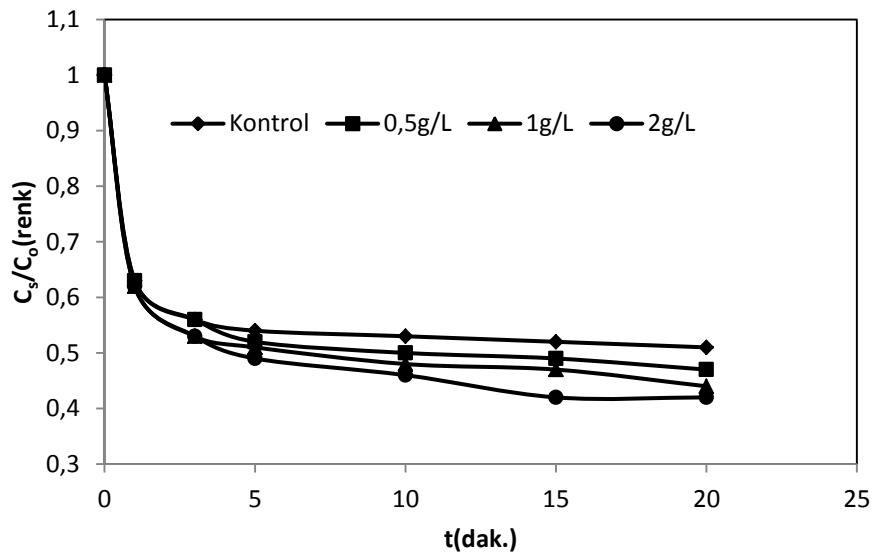
Şekil 4.39. DB71'in ultrasonik parçalanmasına Cu 0 'in etkisi
