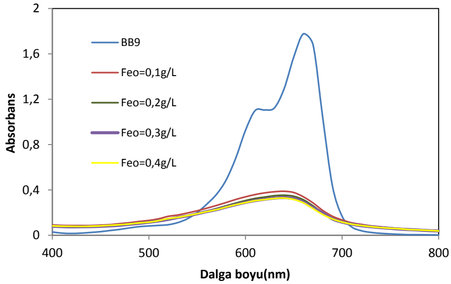
Şekil 4.10. BB9'un Fenton-benzeri oksidasyonunda Fe o konsantrasyonunun absorbanans azalmasına etkisi
