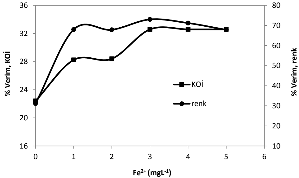
Şekil 4.16. DB71'in Fenton oksidasyonunda Fe +2 miktarının renk ve KOİ giderme verimine etkisi
