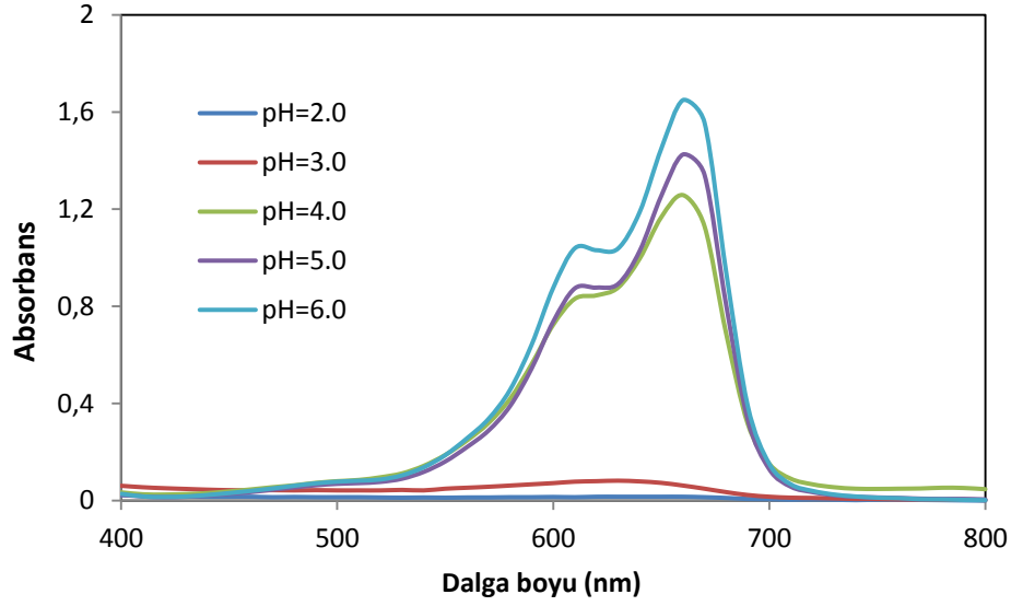
Şekil 4.12. BB9'un Fenton-benzeri oksidasyonunda pH'nin absorptans azalmasına etkisi *( C_0=100 \text{ mgL}^{-1} , Fe^0=0,1 \text{ gL}^{-1} , H_2O_2=75 \text{ mgL}^{-1} , T=20^0C , t=20 \text{ dak.} )
