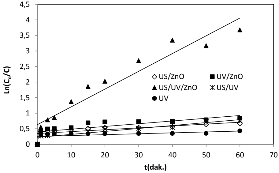
Şekil 4.77. BB9'un farklı şartlardaki renk gideriminin birinci derece kinetik grafiği *( C_0=30 \text{ mgL}^{-1} , \text{ZnO}=400 \text{ mgL}^{-1} , \text{pH}=5.5 , T=20^0\text{C} , t=60 \text{ dak.} )
