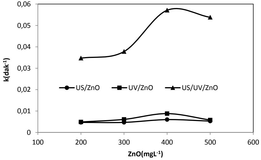
Şekil 4.76. BB9'un farklı şartlardaki renk giderimine ZnO'nun etkisi *( C_0=30 \text{ mgL}^{-1} , \text{pH}=5.5 , T=20^0\text{C} , t=60 \text{ dak.} )
