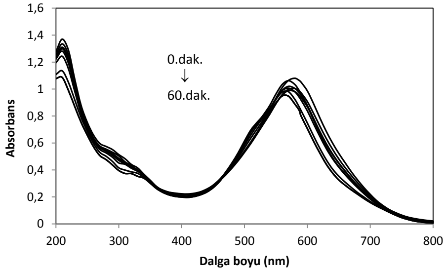
Őekil 4.57. DB71'in 254 nm UV oksidasyonu
