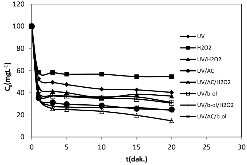
Şekil 4.62. DB71'in heterojen UV oksidasyonu sonucu kalan boyar madde konsantrasyonu
