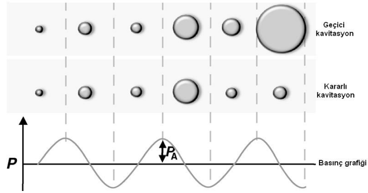
Şekil 2.5. Kaviteasyon oluşumu.
