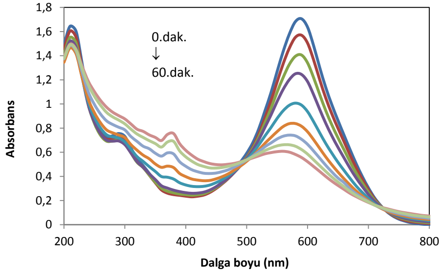
Şekil 4.72. DB71'in sonofotokatalitik oksidasyon ile renk gideriminin absorbans azalması
