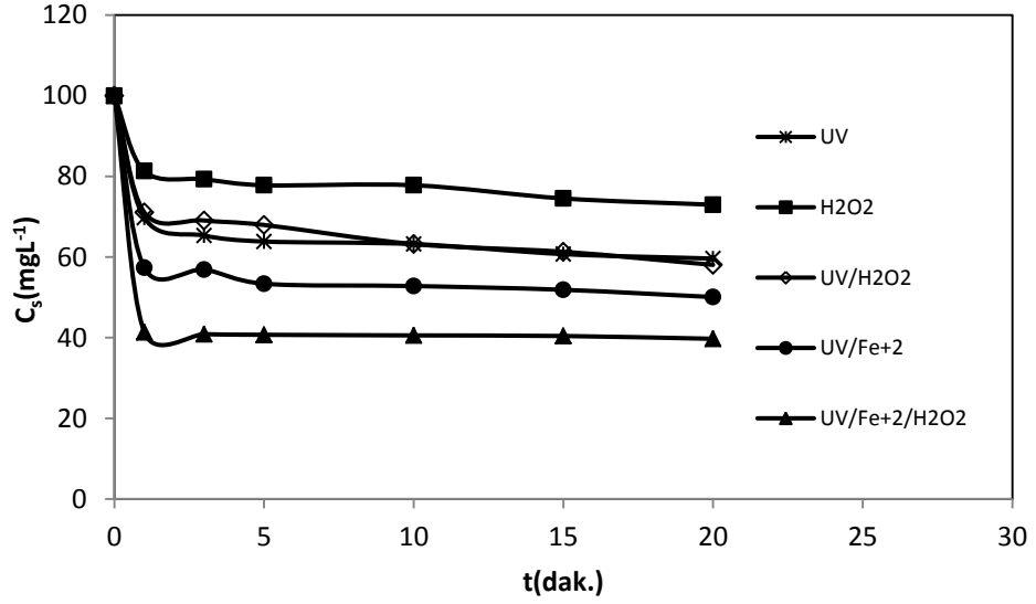
Şekil 4.58. DB71'in homojen UV oksidasyonu sonucu kalan boyar madde konsantrasyonu
