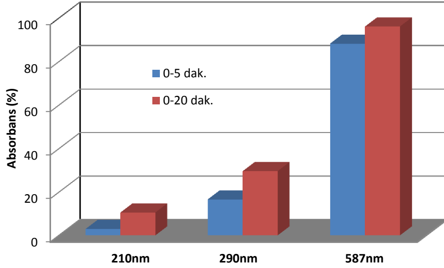
Şekil 4.31. DB71 boyar maddesinin Fenton-benzeri oksidasyonunda farklı pik ve zamanlarda elde edilen absorbanans verimleri ( C_0=30 \text{ mgL}^{-1} , \text{Fe}^0=0,1 \text{ gL}^{-1} , \text{H}_2\text{O}_2=50 \text{ mgL}^{-1} , \text{pH}=3,5 , T=20^\circ\text{C} , t=20 \text{ dak.} )
