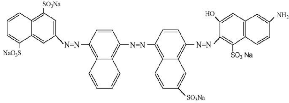
Şekil 3.2. DB71 boyar maddesinin moleküler yapısı (Saien and Soleymani 2007).
