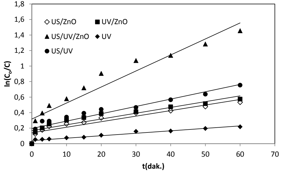
Şekil 4.70. DB71'in farklı şartlardaki renk gideriminin birinci derece kinetik grafiği *( C_0=30 \text{ mgL}^{-1} , \text{ZnO}=400 \text{ mgL}^{-1} , \text{pH}=5.5 , T=20^0\text{C} , t=60 \text{ dak.} )
