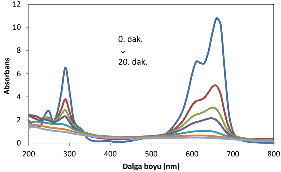
Şekil 4.1. BB9'un Fenton oksidasyonunda renk gideriminin absorbans azalması *( C_0=60 \text{ mgL}^{-1} , \text{Fe}^{2+}=1,5 \text{ mgL}^{-1} , \text{H}_2\text{O}_2=50 \text{ mgL}^{-1} , \text{pH}=3,0 , T=20^\circ\text{C} , t=20 \text{ dak.} )
