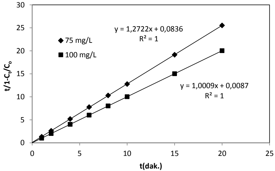
Şekil 4.9. Farklı H 2 O 2 konsantrasyonları ile BB9'un Fenton oksidasyonu ile renk giderimindeki BMG kinetik modeli *(C 0 =100 mgL -1 , Fe 2+ =3 mgL -1 , pH=3.0, T=20 0 C)
