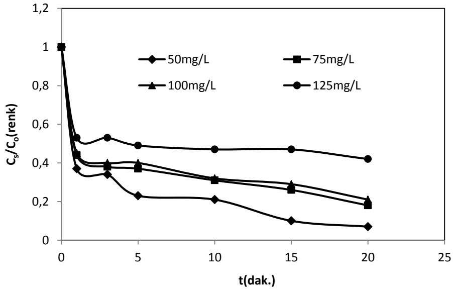
řekil 4.48. DB71'in ultrasonik paręalanmasına boyar madde konsantrasyonunun etkisi *(aktif karbon =1g -1 , pH=2.0, amplitude=%90, T=20 0 C, t=20 dak.)
