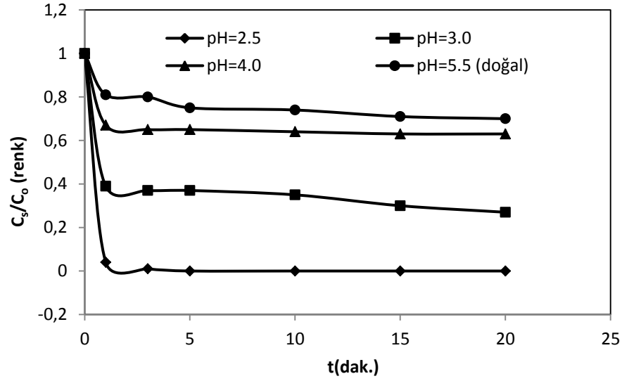
Şekil 4.41. DB71'in ultrasonik parçalanmasına pH değerinin etkisi *( C_0=50 \text{ mgL}^{-1} , \text{ZnO}=2 \text{ gL}^{-1} , amplitude=%90, T=20^\circ\text{C} , t=20\text{dak.} )
