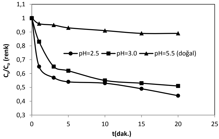
Şekil 4.38. DB71'in ultrasonik parçalanmasına pH'nin etkisi
