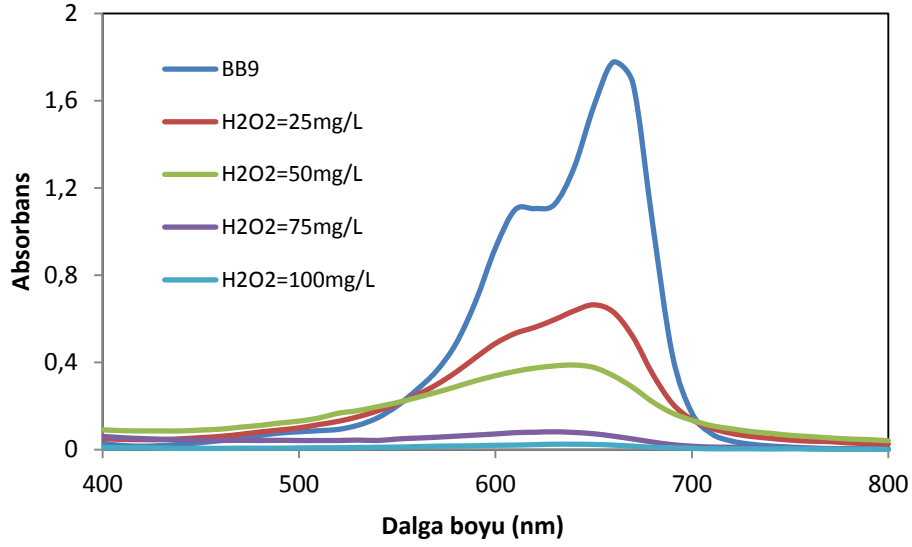
Şekil 4.11. BB9'nun Fenton-benzeri oksidasyonunda H_2O_2 konsantrasyonunun absorbands azalmasına etkisi
