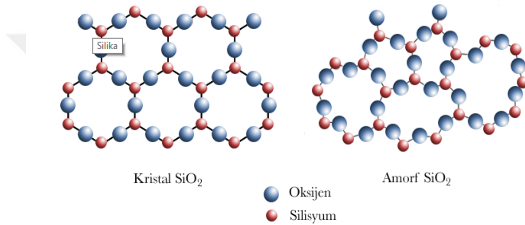
Şekil 2.2. Kristalin ve amorf formundaki silisyum dioksit [23].
