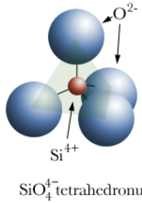
Şekil 2.1. Silisyum dioksit [23].
