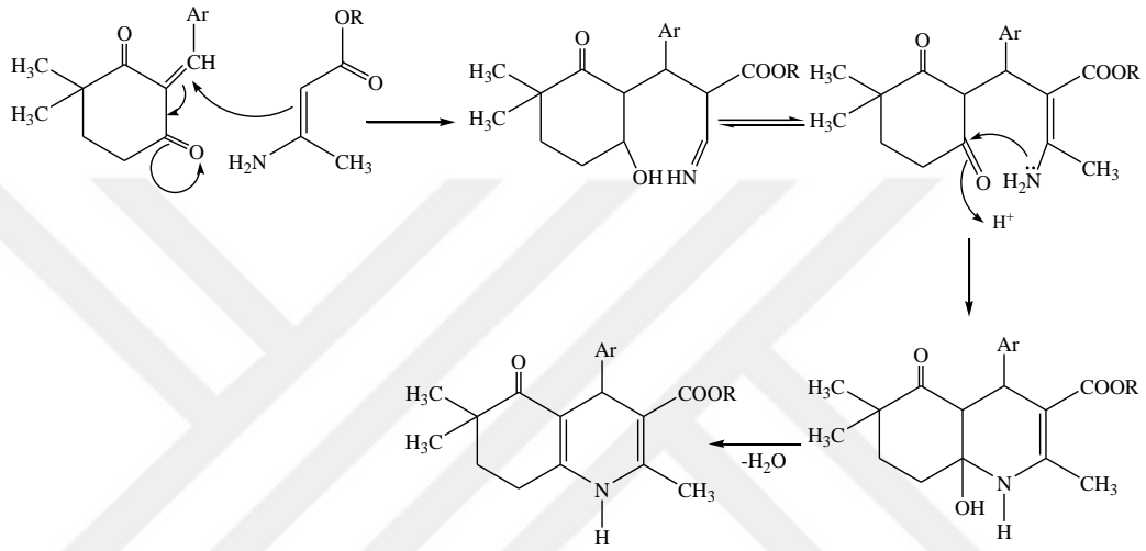
Şekil 5.2. Hekzahidrokinolin oluşum mekanizması.
