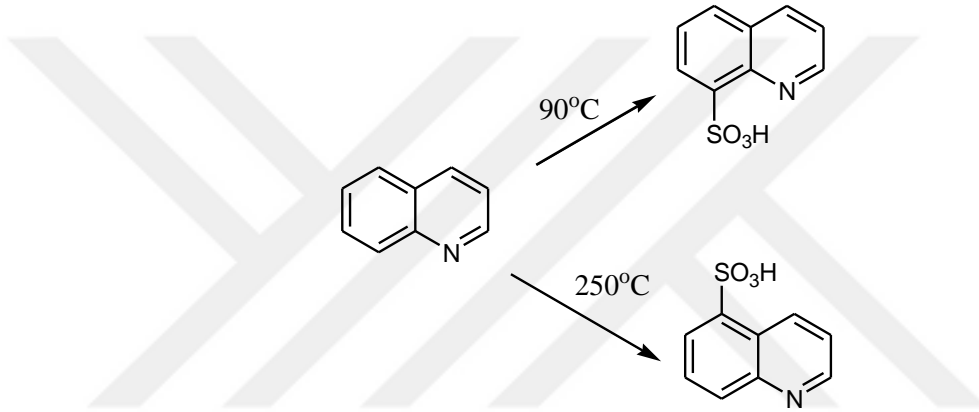
Şekil 2.41. Kinolinin sülfonlanması.
