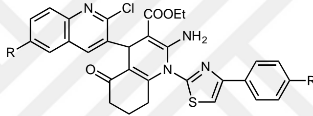
Şekil 2.54. Tiyazolilbikinolin türevleri.
