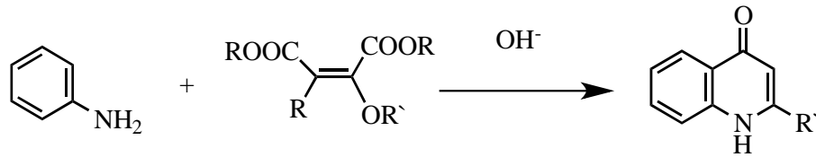
Şekil 2.39. Gould-Jacobs sentezi.
