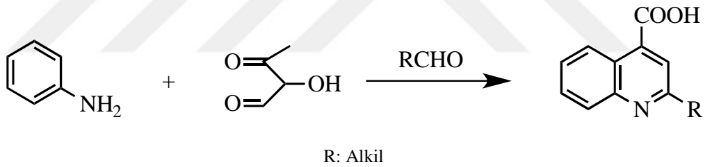
Şekil 2.36. Doebner Reaksiyonu
