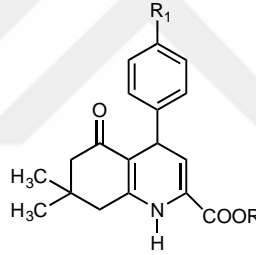
Şekil 2.70. 2,4-Disübstitüe hekzahidrokinolin türevleri.
