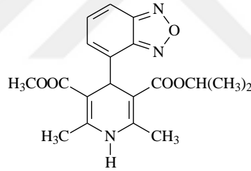
Şekil 2.65. İsradipin.
