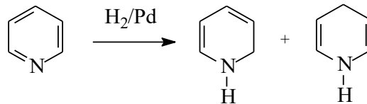
Şekil 2.23. Piridin ve piridinyum tuzlarının katalitik indirgenmesi.
