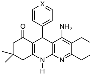
Şekil 2.66. Takrin-hekzahidrokinolin türevi.
