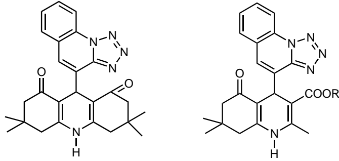
Şekil 2.53. Tetrazolokinolin türevleri.
