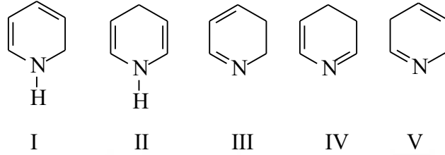
Şekil 2.1. DHP izomerleri.
