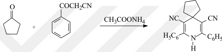
Şekil 2.16. Spiro-1,4-DHP'lerin sentezi.
