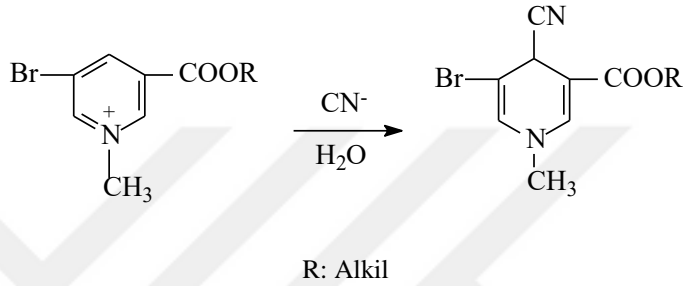
Şekil 2.25. 4-Siyano-1,4-DHP türevlerinin sentezi.
