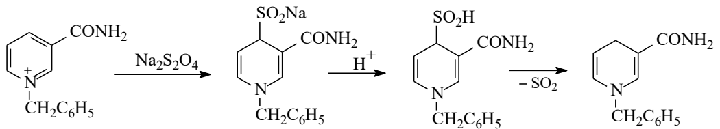
Şekil 2.26. Ditiyonit reaksiyonu.
