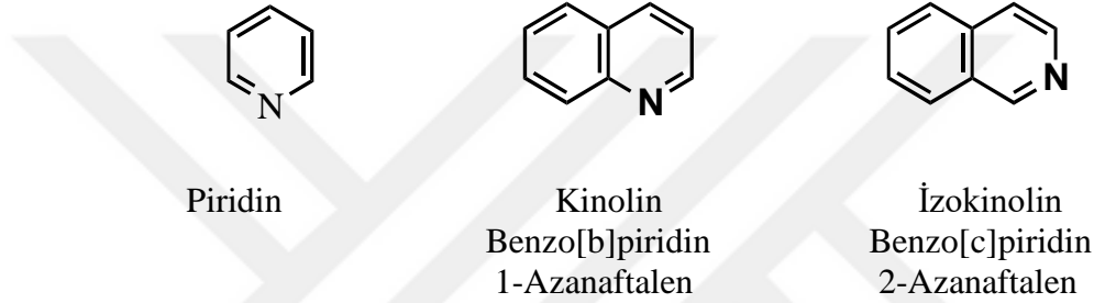
Şekil 2.32. Piridin ve kinolinler.
