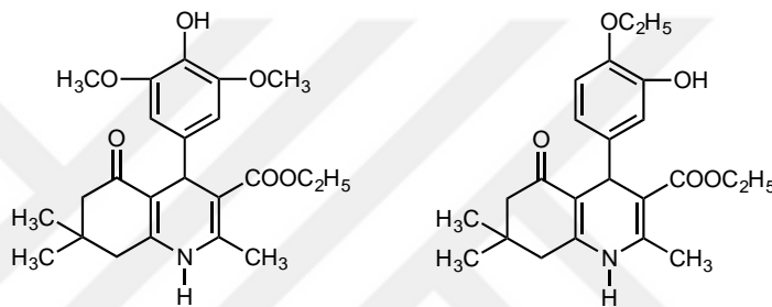
Şekil 1.5. 5-Oksoheksahidrokinolin-3-karboksilat türevleri.
