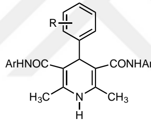
Şekil 1.3. 3,5-Dikarbamoil-4-aril-1,4-DHP.
