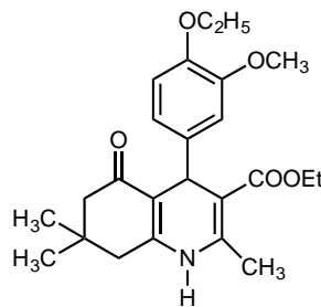
Şekil 2.58. 5-Hekzahidrokinolin türevleri.
