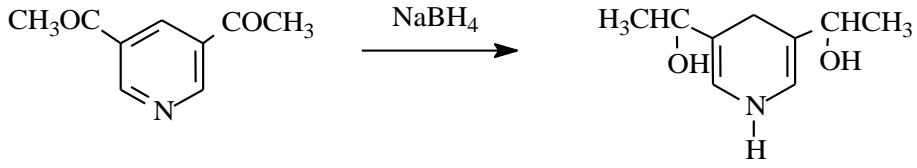
Şekil 2.24. 3,5-Diasetilpiridin'in sodyum borohidürle redüksiyonu.
