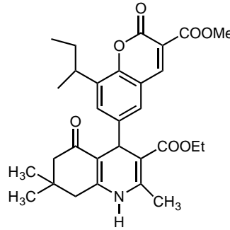
Şekil 2.68. Kumarin-hekzahidrokinolin türevi.
