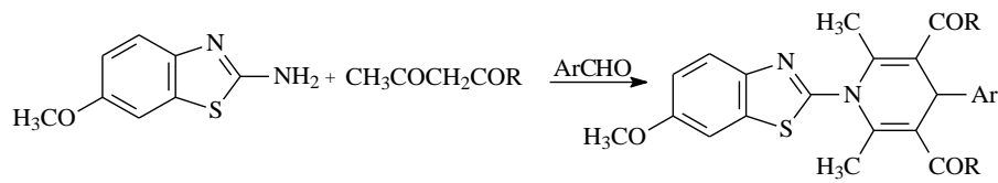
Şekil 2.20. N-(2-benzotiyazolil)-4-aril-1,4-DHP sentezi.
