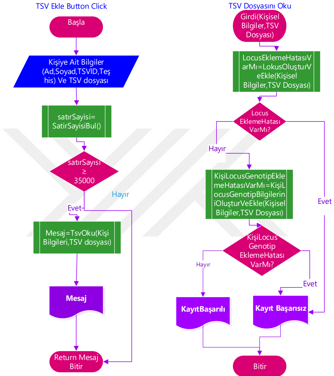
Şekil 3.6. Veri aktarım uygulaması akış diyagramı. Uygulama arayüzünde yer alan “Dosya Seç” tuşuna tıkladığında “ExcelReading” ClassLibrary projesinde gerçekleştirilen işlemlere ilişkin akış diyagramı solda, diyagram içerisinde çağrılan “TSVDosyasınıOku” fonksiyonun gerçekleştirdiği işlemlere ilişkin akış diyagramı ise sağda gösterilmiştir.
