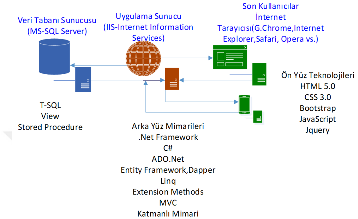
Şekil 3.1. Çalışmada kullanılan 3 katmanlı mimari. Sol tarafta veri tabanı sunucusu ve veri tabanın oluşturulmasında kullanılan teknolojiler; ortada veri tabanı ile ön yüzün birbiriyle iletişimi sağlayan arka yüzde bulunan uygulama sunucusu ve bunun oluşturulmasında kullanılan teknolojiler; sağ tarafta ise ön yüzde son kullanıcının oluşturulan sistemi kullanmasını sağlayan ve kolaylaştıran teknolojiler yer almaktadır.
