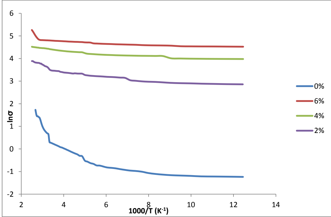
Şekil 4.6 10 katlı numune için farklı katkılama miktarlarında \ln(\sigma) - 1000/T grafiği
