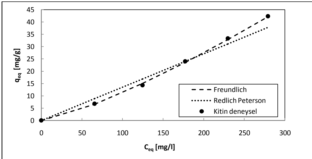
Şekil 6.73. Kitin ile metil kırmızısı boyar maddesi adsorpsiyonu için Freundlich ve Redlich Peterson modellerinin karşılaştırılması ( T=25^{\circ}\text{C} , \text{pH}=5 , m_{\text{sorbent}}= 0.8 \text{ g} , 150 \text{ rpm} ).
