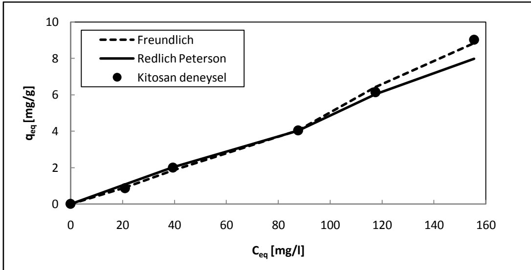
Şekil 6.33. Kitosan ile çinko(II) adsorpsiyonu için Langmuir, Freundlich ve Redlich Peterson modellerinin karşılaştırılması ( T=25^{\circ}\text{C} , \text{pH}=5 , m_{\text{sorbent}}= 0.8\text{g}, 150 \text{ rpm} ).
