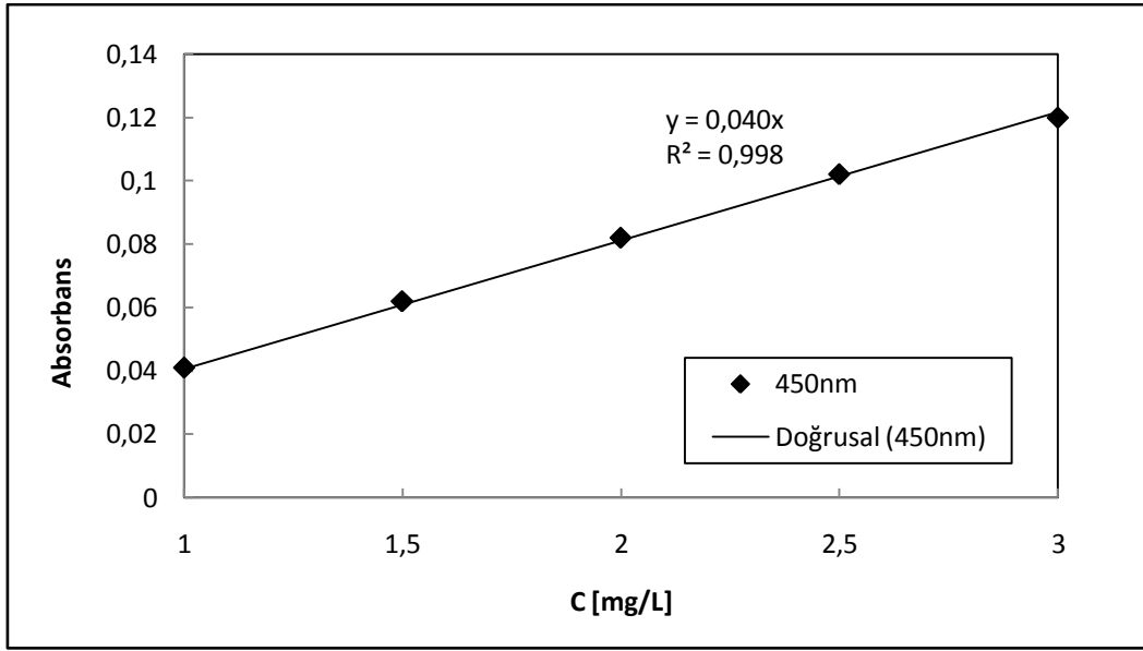
Şekil E.3. Metil Kırmızısı boyar maddesi kalibrasyon grafiđi
