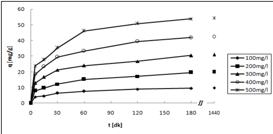
Şekil 6.71. Artan başlangıç boyar madde derişimlerinde birim sorbent ağırlığı başına kitosana adsorplanan metil kırmızısı boyar maddesi miktarının zamanla deęiřimi ( T=25^{\circ}\text{C} , \text{pH}=5 , m_{\text{sorbent}}= 0.8 \text{ g} , 150 \text{ rpm} ).
