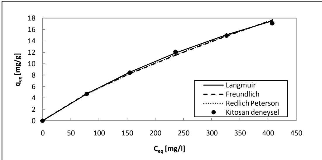
Şekil 6.61. Kitosan ile kristal viyole boyar maddesi adsorpsiyonu için Langmuir, Freundlich ve Redlich Peterson modellerinin karşılaştırılması ( T=25^{\circ}\text{C} , \text{pH}=5 , m_{\text{sorbent}}= 0.8 \text{ g} , 150 \text{ rpm} ).
