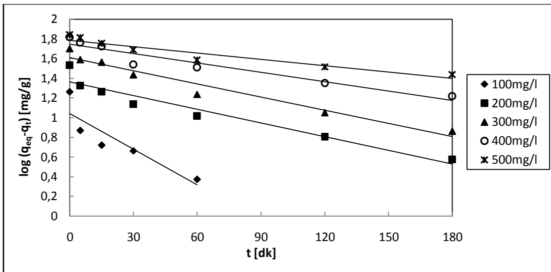
Şekil 6.62. Kitin ile kristal viyole adsorpsiyonunun yalancı birinci dereceden kinetik modele uyumu ( T=25^{\circ}\text{C} , \text{pH}=5 , m_{\text{sorbent}}= 0.8 \text{ g} , 150 \text{ rpm} ).
