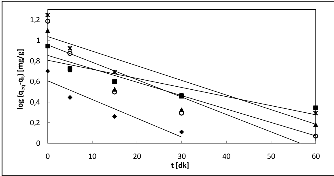
Şekil 6.63. Kitosan ile kristal viyole adsorpsiyonunun yalancı birinci dereceden kinetik modele uyumu ( T=25^{\circ}\text{C} , \text{pH}=5 , m_{\text{sorbent}}= 0.8 \text{ g} , 150 \text{ rpm} ).
