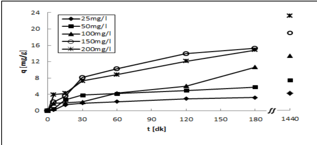
Şekil 6.25. Artan başlangıç çinko(II) iyonu derişimlerinde birim sorbent ağırlığı başına kitine adsorplanan çinko(II) miktarının zamanla deęiřimi ( T=25^{\circ}\text{C} , \text{pH}=5 , m_{\text{sorbent}}= 0.8\text{g} , 150\text{rpm} ).
