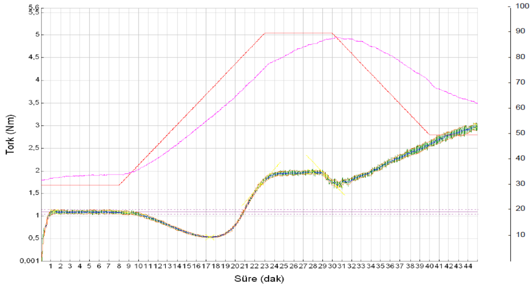
Ek 2. Kuvvetli Unun Miksolab Grafiği
