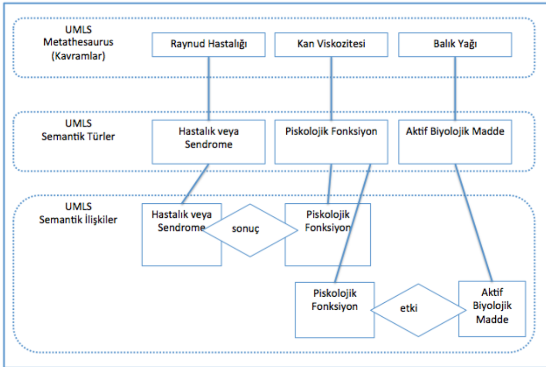
Şekil 4. UMLS Modülleri [51]
