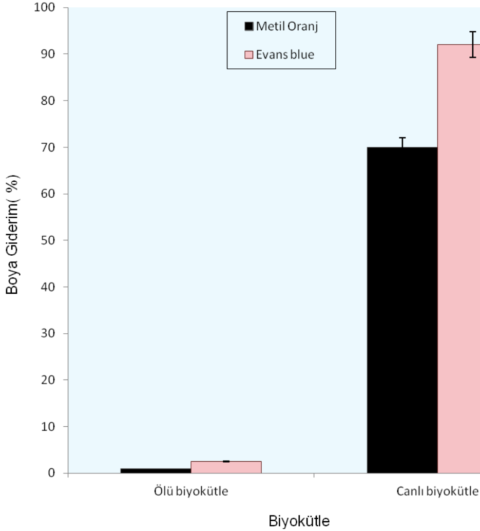
Şekil 4.9. Biyosorpsiyonun Boya Gideriminde Etkisi
