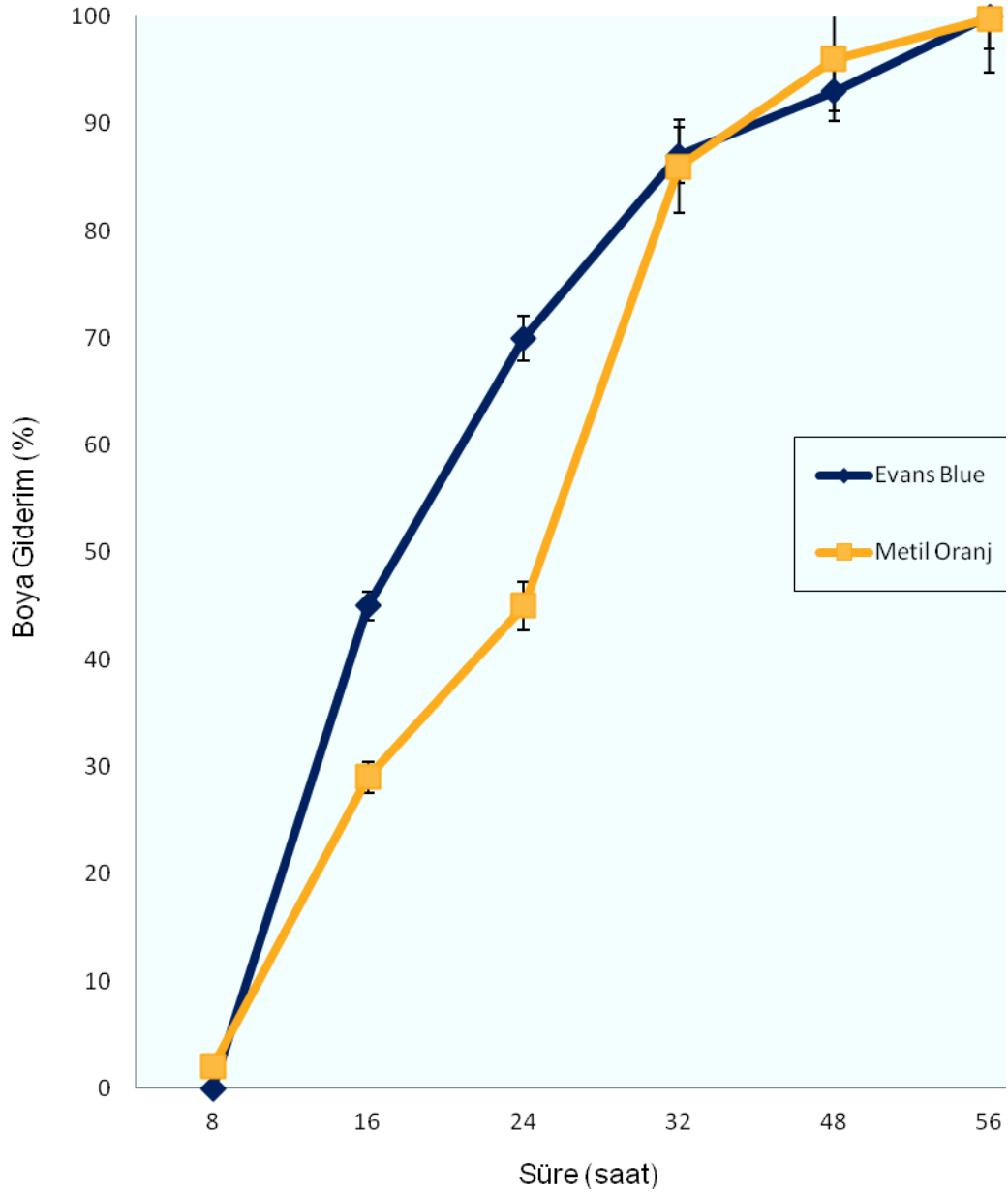
Şekil 4.7. İnkübasyon Süresinin Boya Gideriminde Etkisi.
