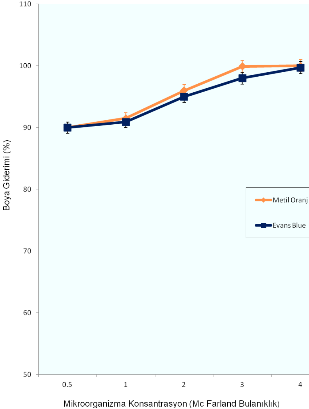
Şekil 4.8. Başlangıç Mikroorganizma Konsantrasyonunun Boya Gideriminde Etkisi. Üretimler bölüm 3.3.3.'te anlatıldığı şekilde gerçekleştirildi. Sonuçlar üç çalışmanın ortalamasıdır. Standart sapmalar grafik üzerinde gösterilmektedir.
