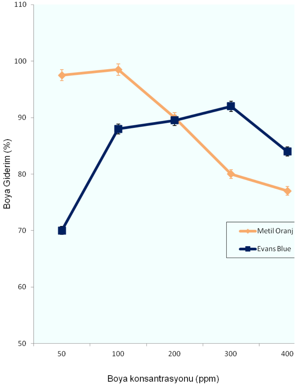
Şekil 4.5. Başlangıç Boya Konsantrasyonunun Boya Gideriminde Etkisi.
