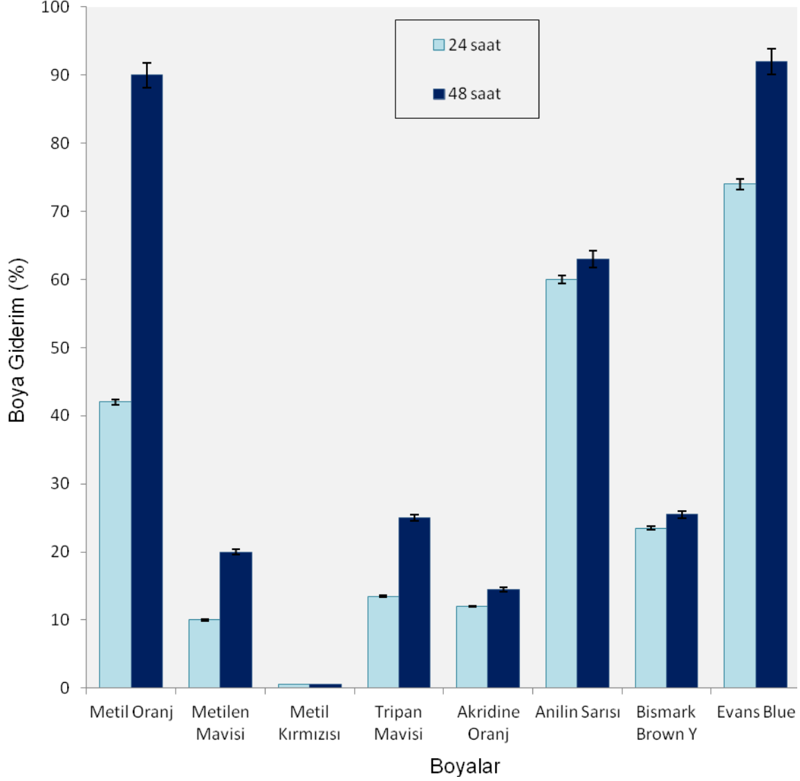
Şekil 4.3. İnkübasyon Süresinin Boya Gideriminde Etkisi.
