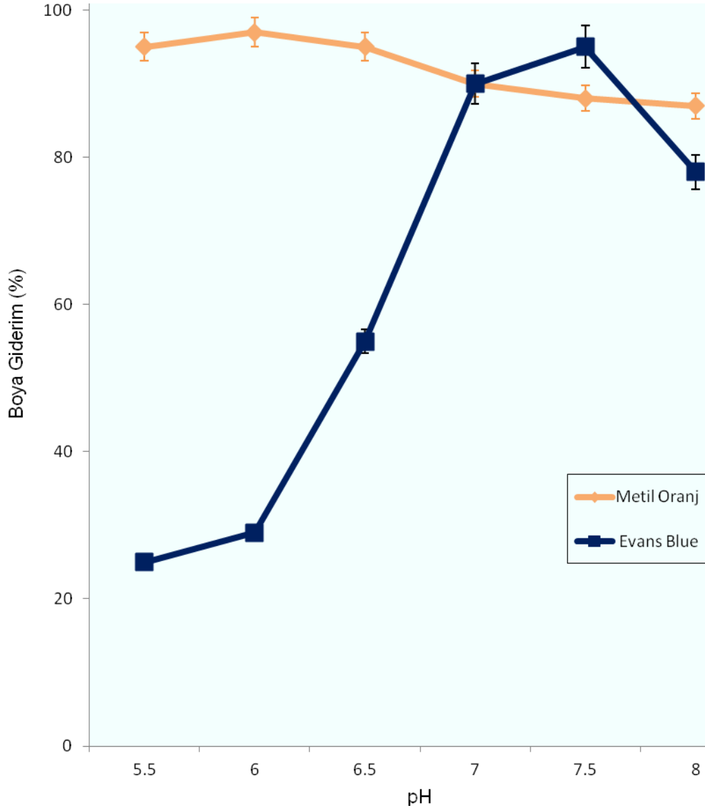
Şekil 4.4. Başlangıç pH Değerinin Boya Gideriminde Etkisi.
