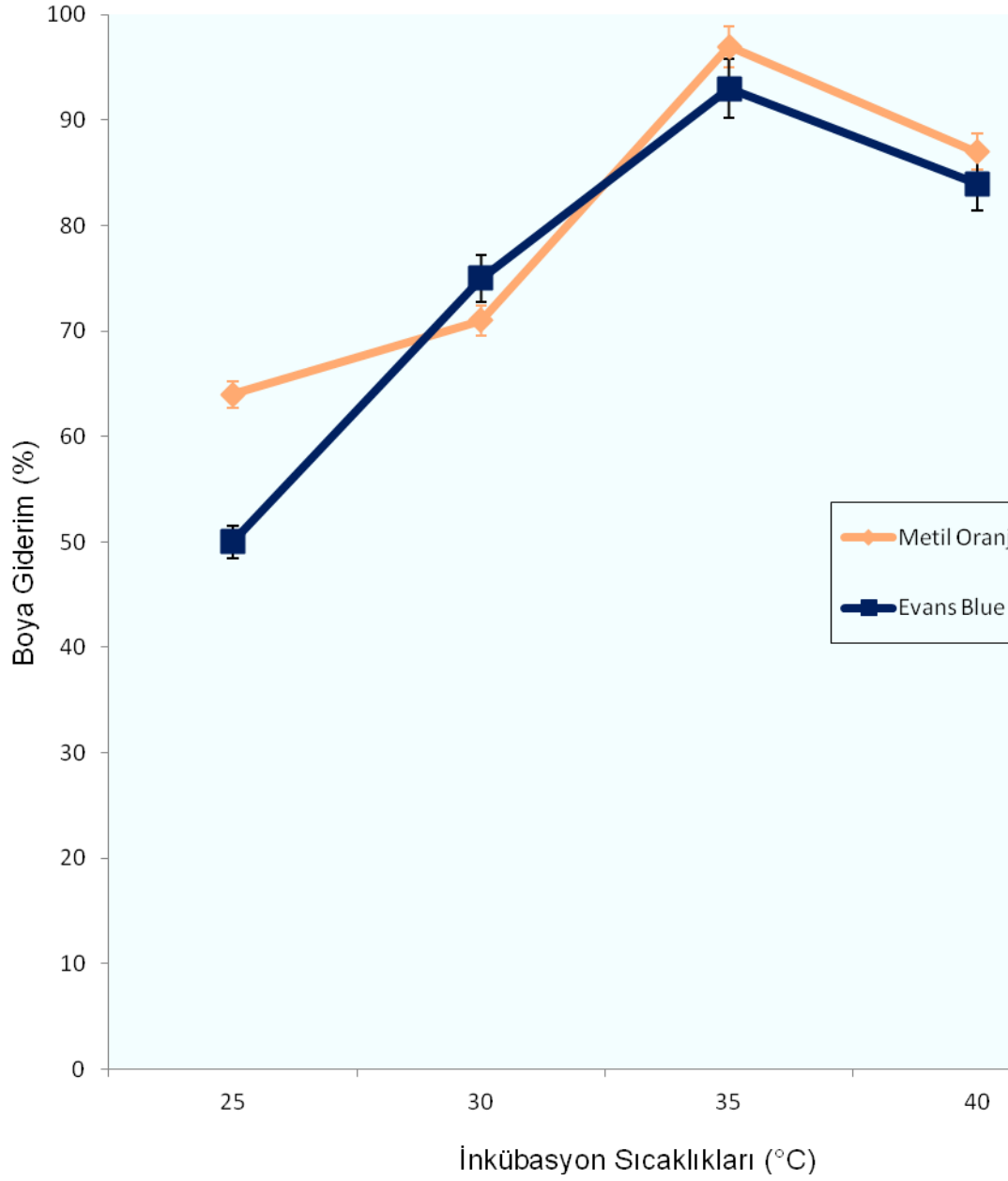
Şekil 4.6. İnkübasyon Sıcaklığının Boya Gideriminde Etkisi.
