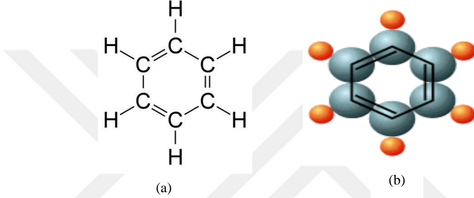
Şekil 2.4. Benzenin yapısı
